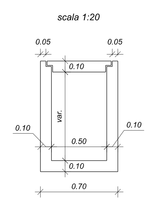
Dettaglio "2" - Canaletta idraulica
