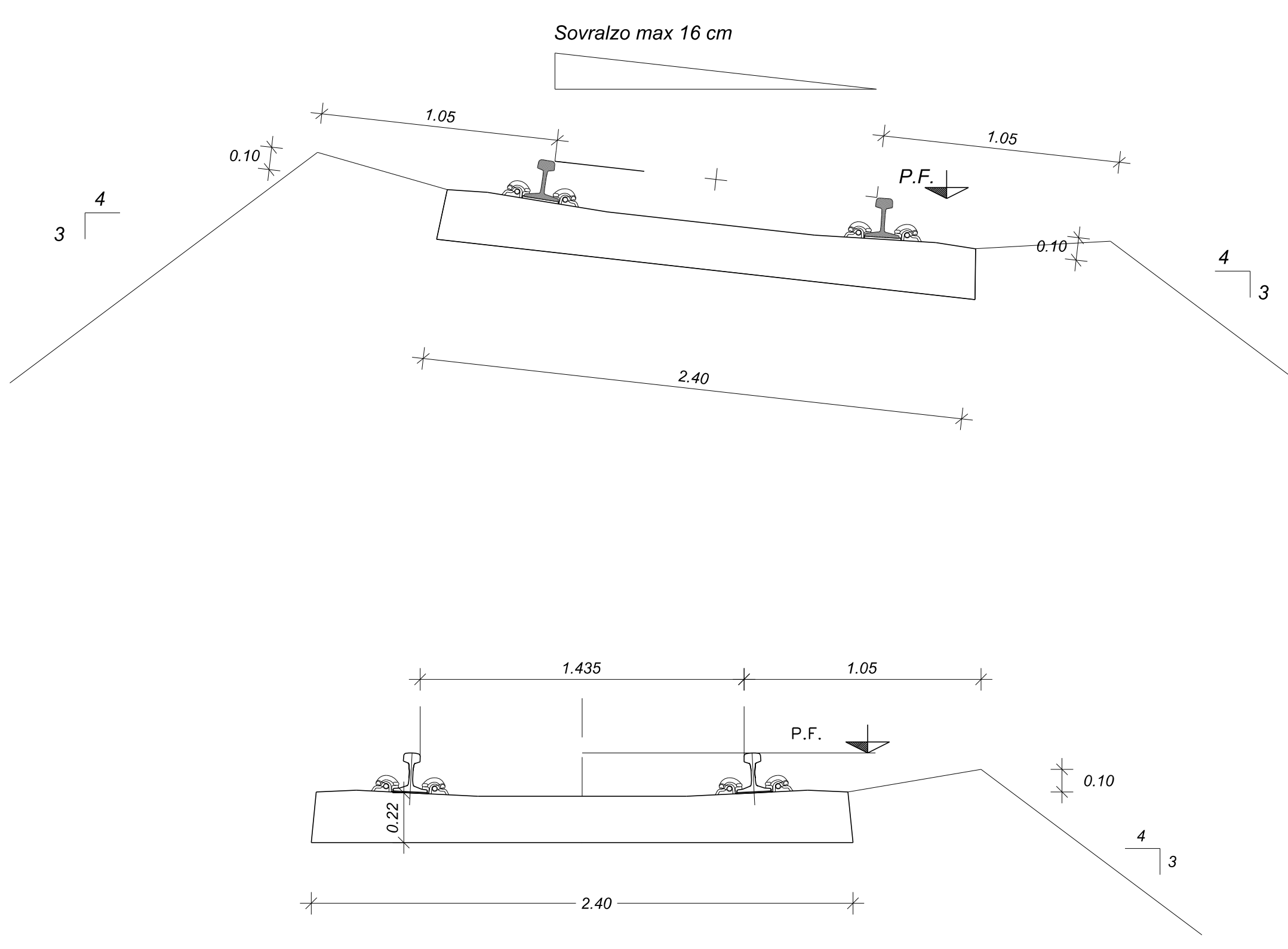
Dettaglio 1 - Andamento traversa in rettilo ed in curva
