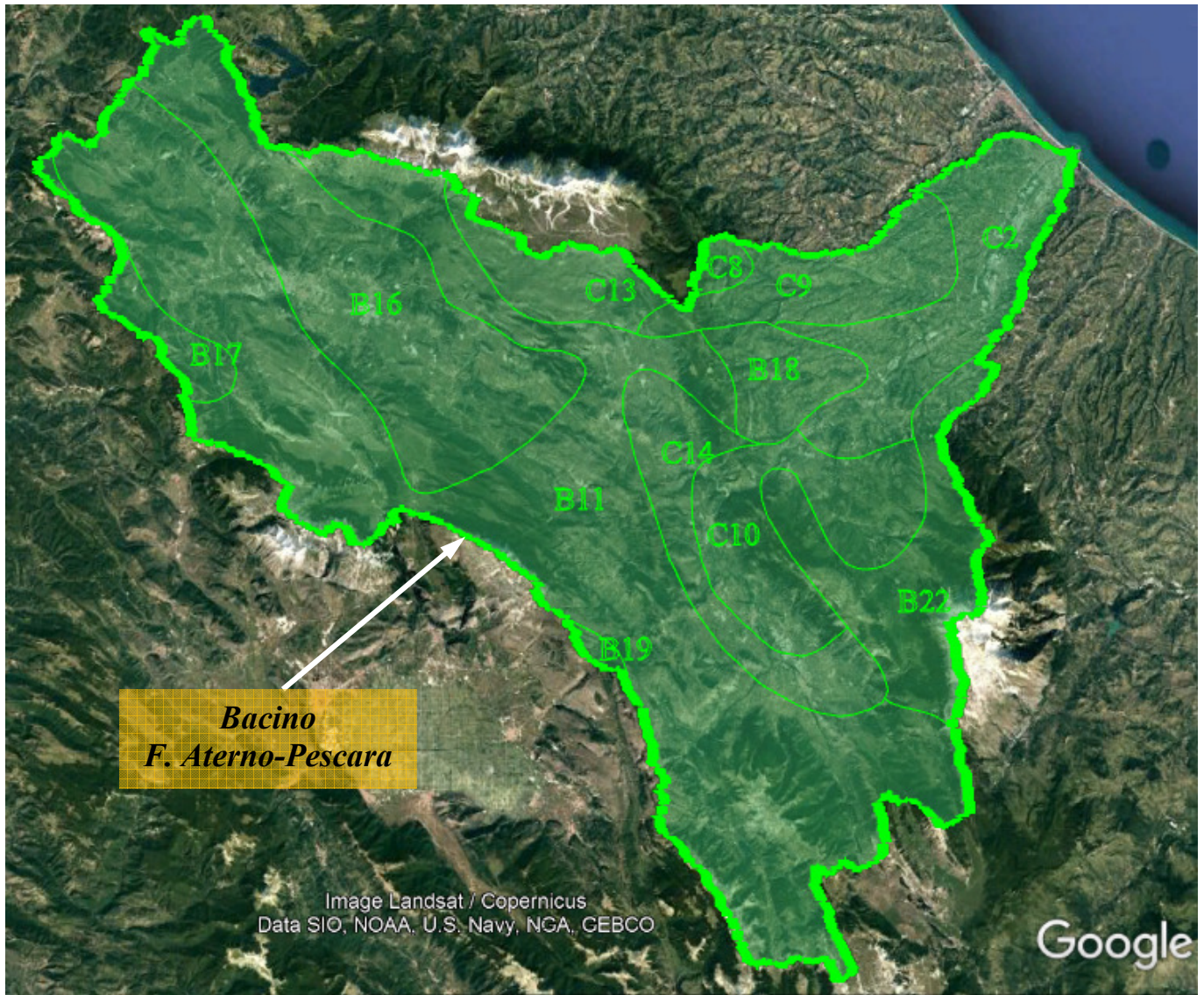
Fig. 6 – Sottozone pluviometriche omogenee (Va.Pi.) all'interno del Bacino del F. Aterno-Pescara.
