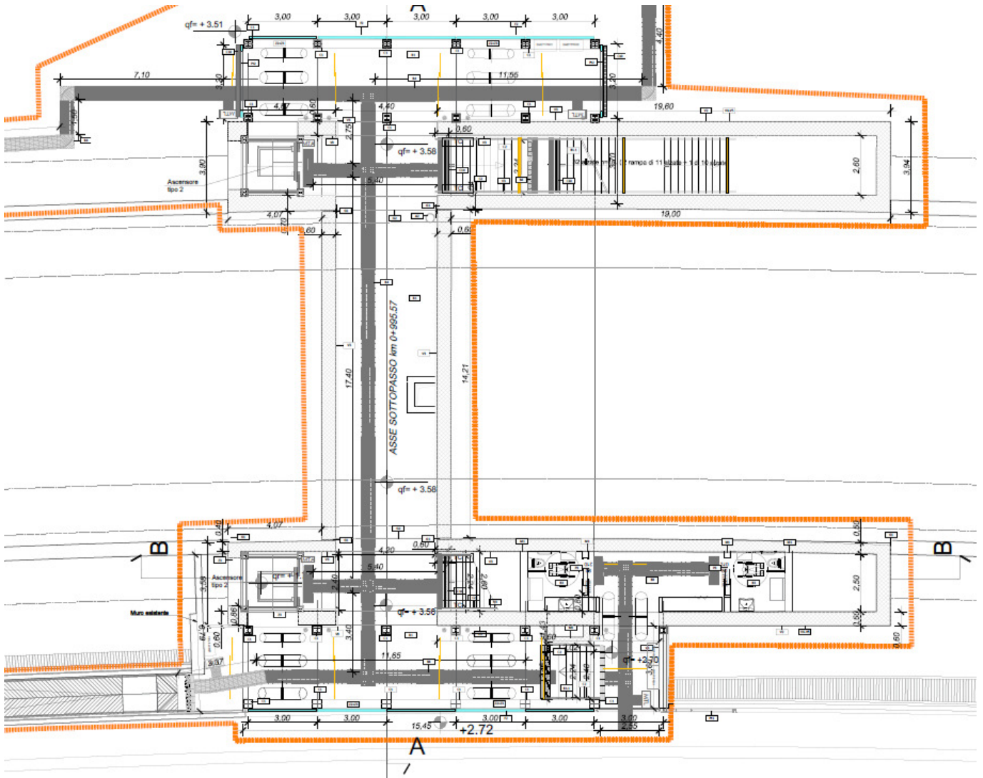
Figura 3. Pianta sottopasso
