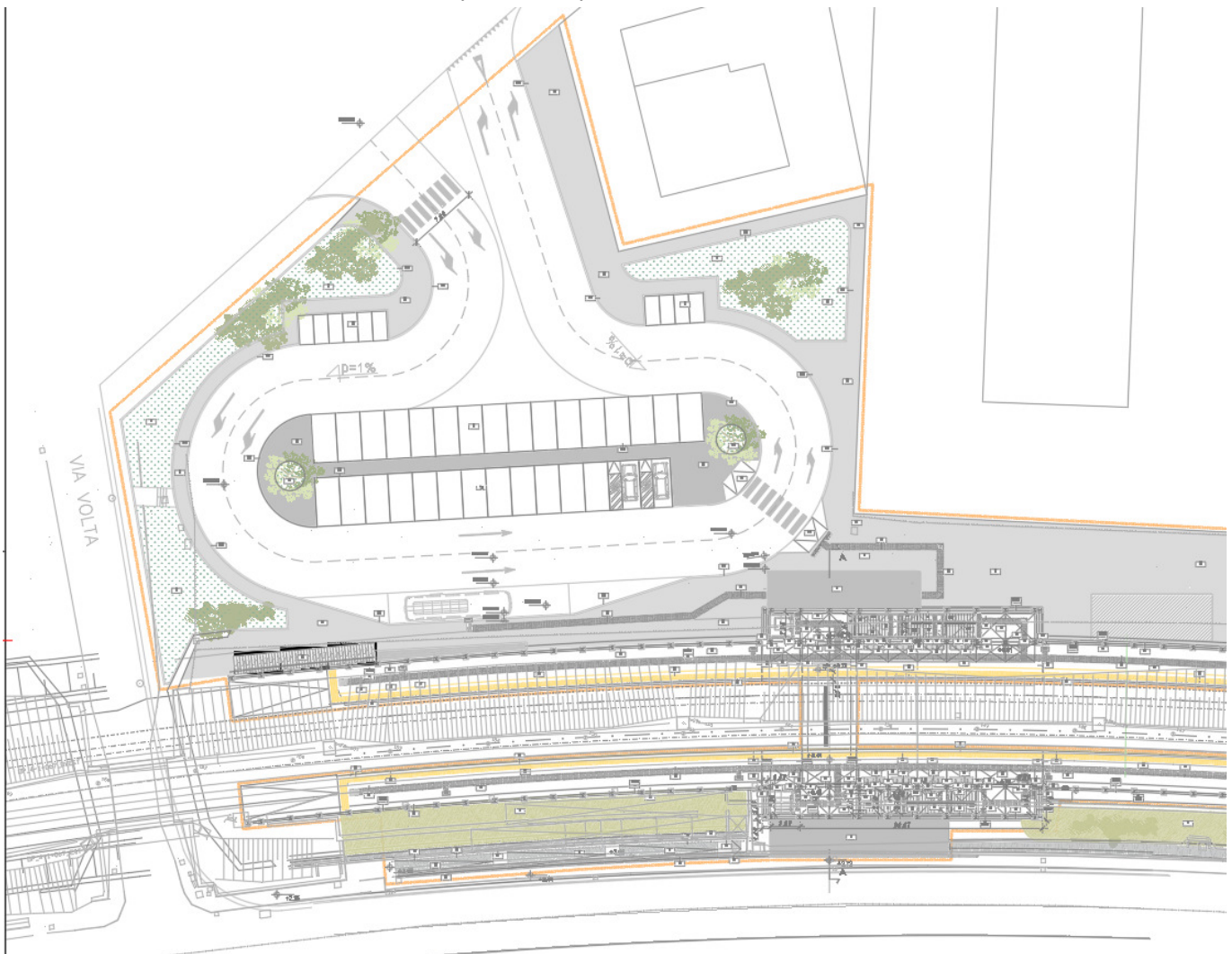
Figura 1. Planimetria
