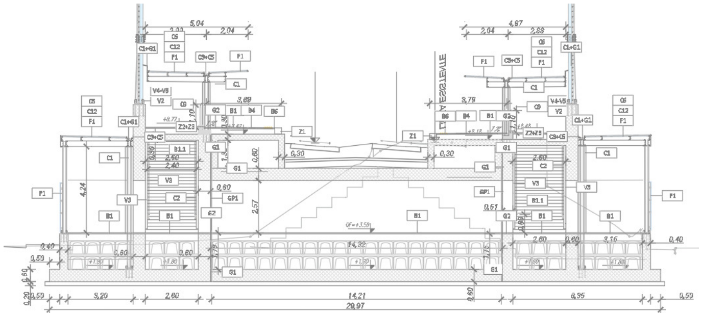
Figura 4. Sezione sottopasso
