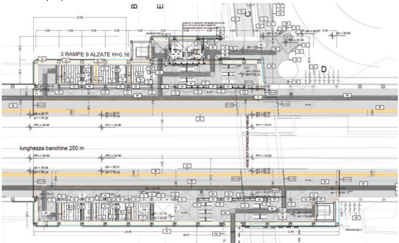
Figura 2. Banchina
