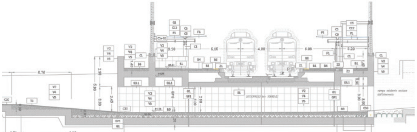
Figura 4. Sezione sottopasso
