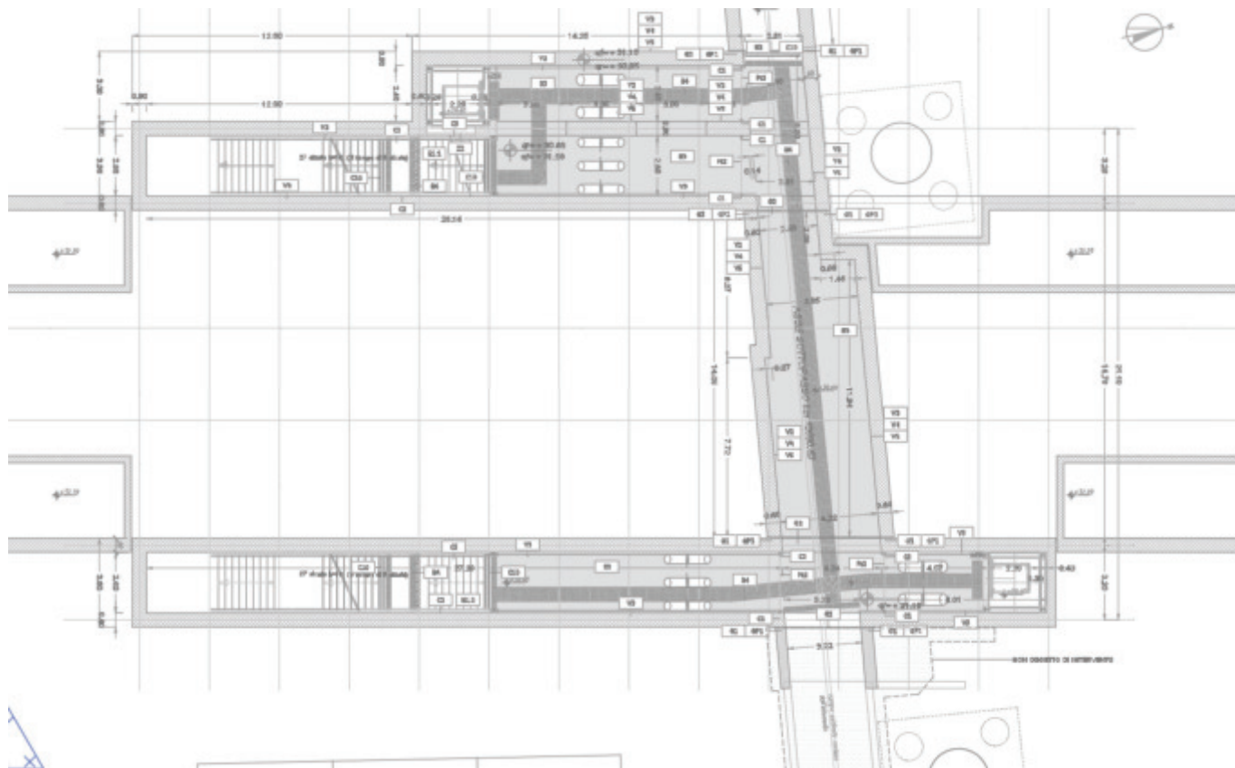
Figura 3. Pianta sottopasso
