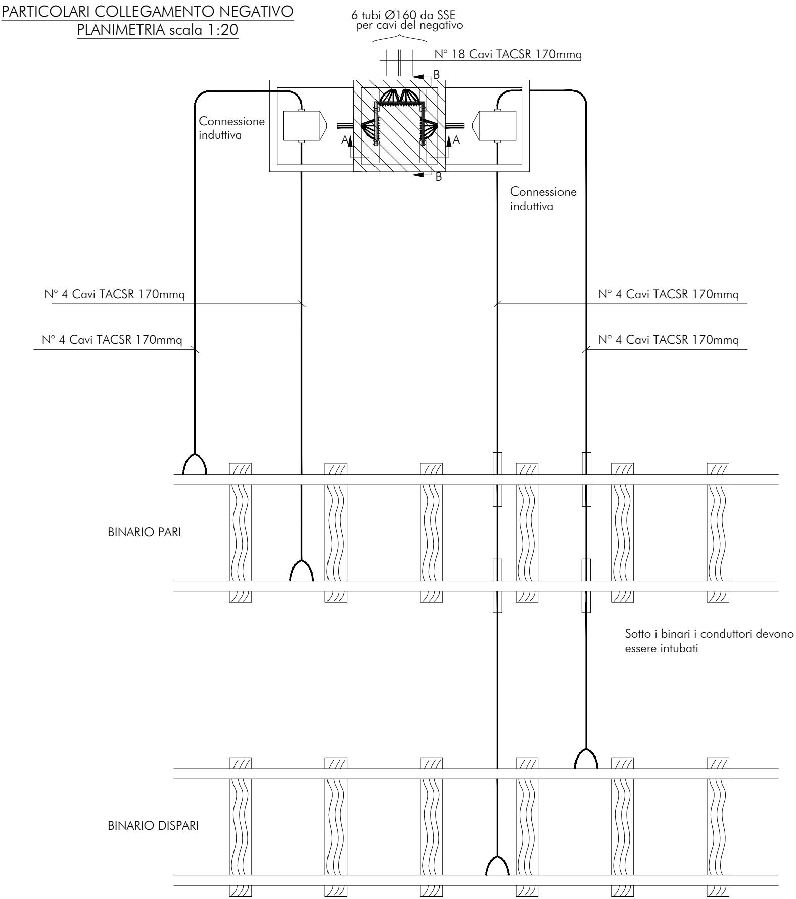
PARTICOLARI - CONNESSIONE AL BINARIO
