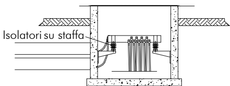
SEZIONE B-B scala 1:20
