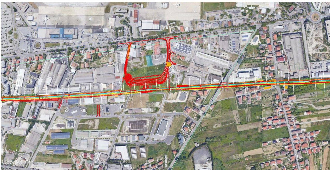
Figura 2-4 – Raddoppio ferroviario dal km 2+400 al km 3+200
