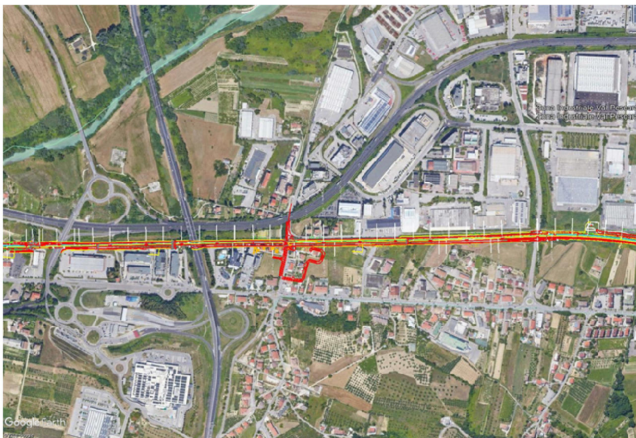
Figura 2-2 – Raddoppio ferroviario dal km 6+800 al km 7+700
