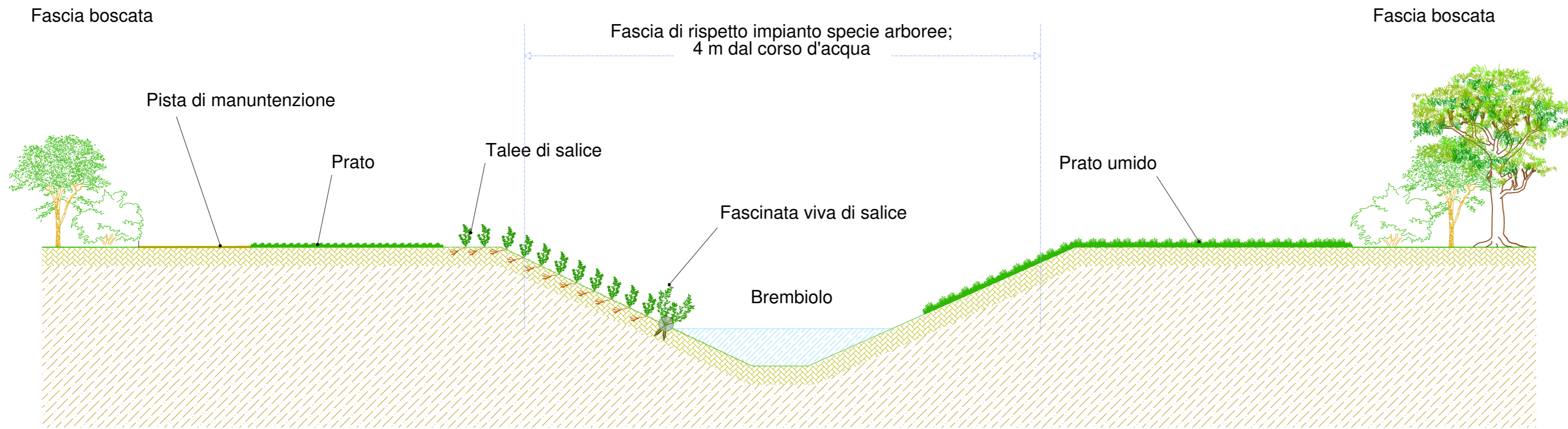
SEZIONE A-A' - SCALA 1:100. INTERVENTO INTERNO AL PLIS BREMBIOLO
