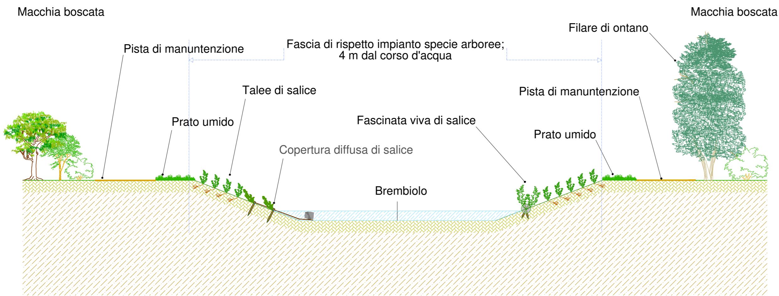
SEZIONE B-B' - SCALA 1:100. INTERVENTO INTERNO AL PLIS BREMBIOLO
