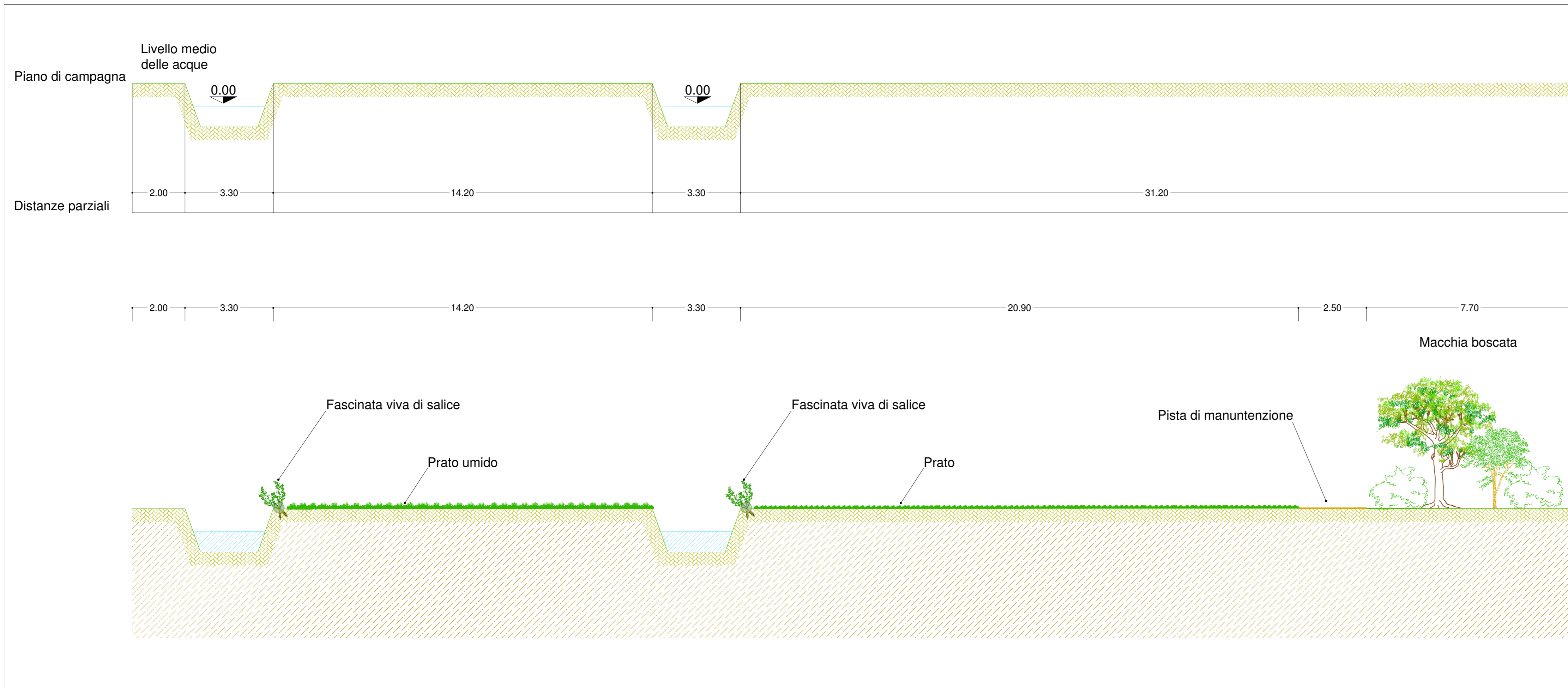
SEZIONE C-C' - SCALA 1:100.
