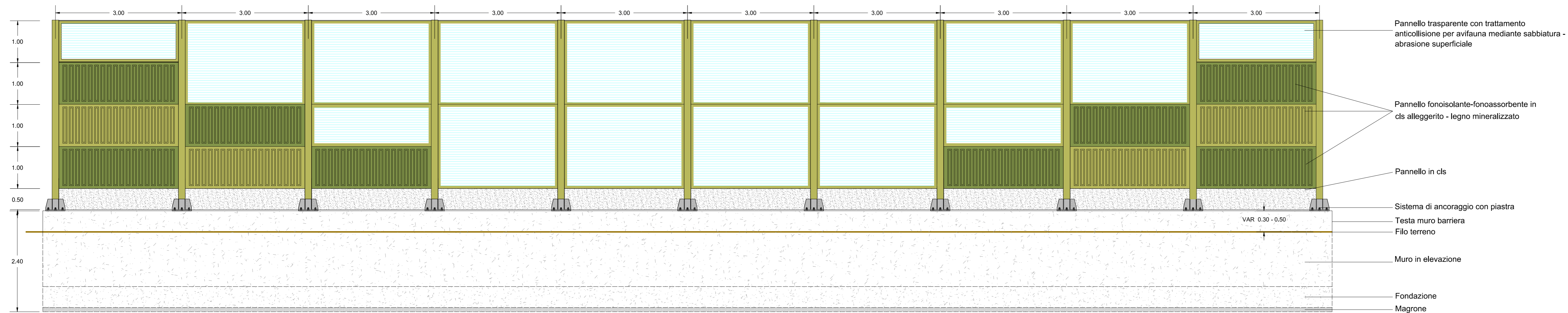
Barriera acustica (h 4.5 m) - soluzione finestrata
