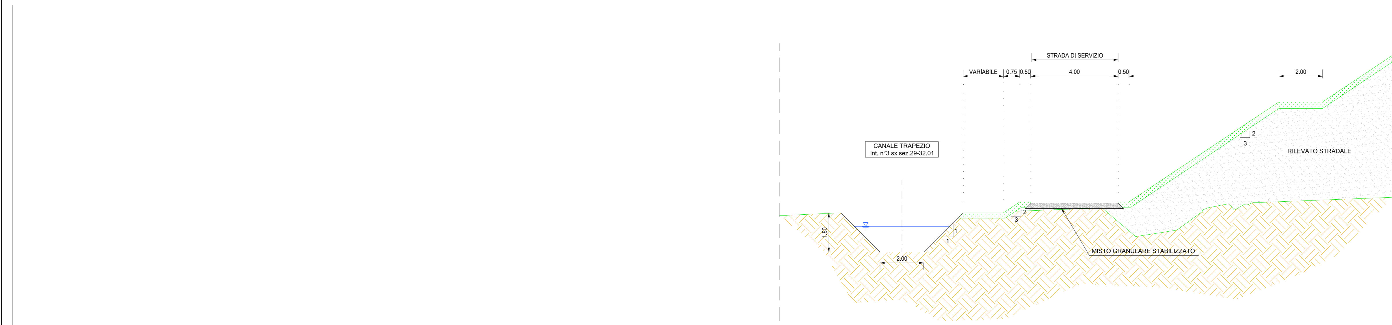
SEZIONI TIPO CANALE SX N°3 SCALA 1:100
