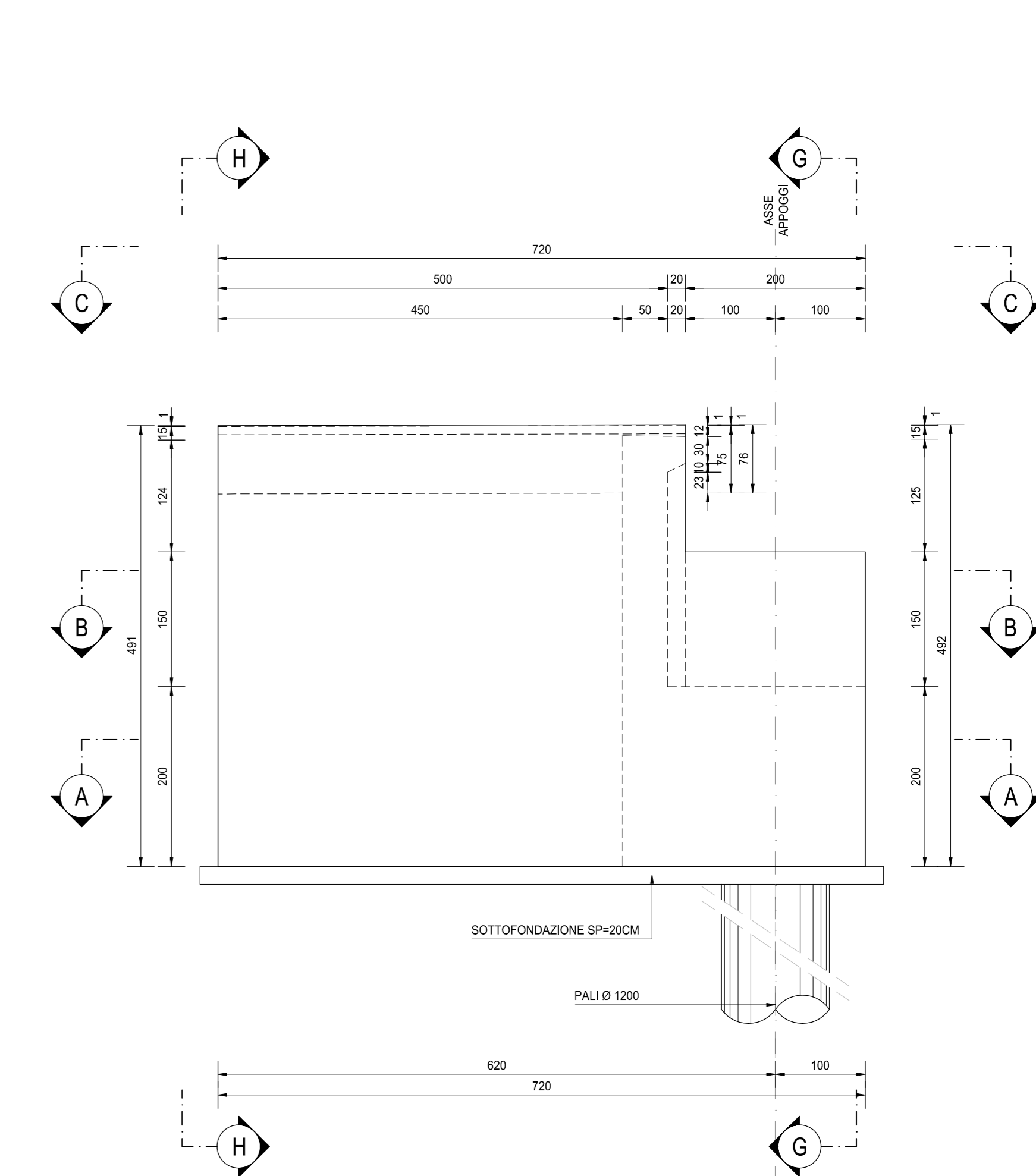
VISTA E-E SCALA 1:50
