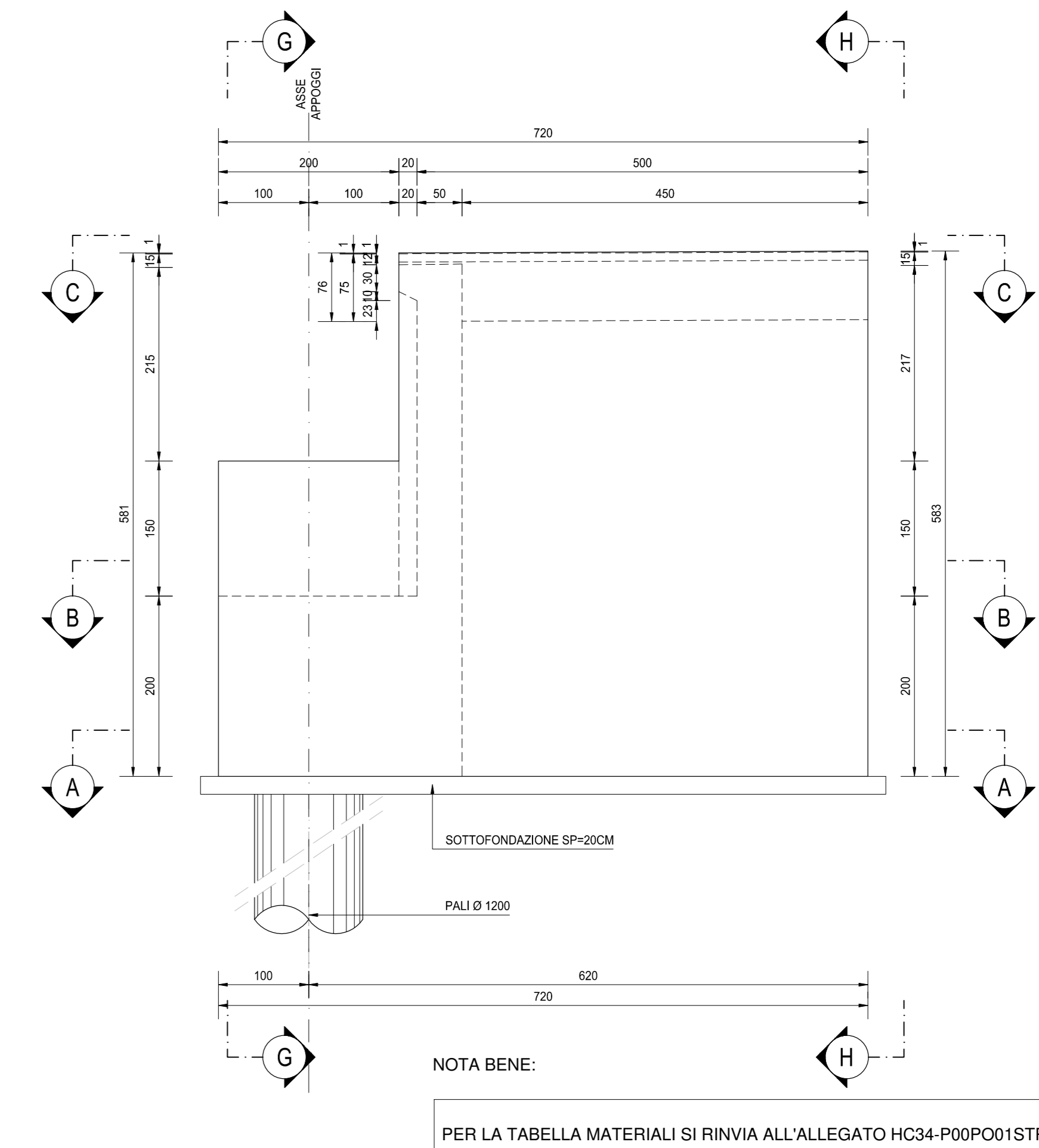
VISTA F-F SCALA 1:50
