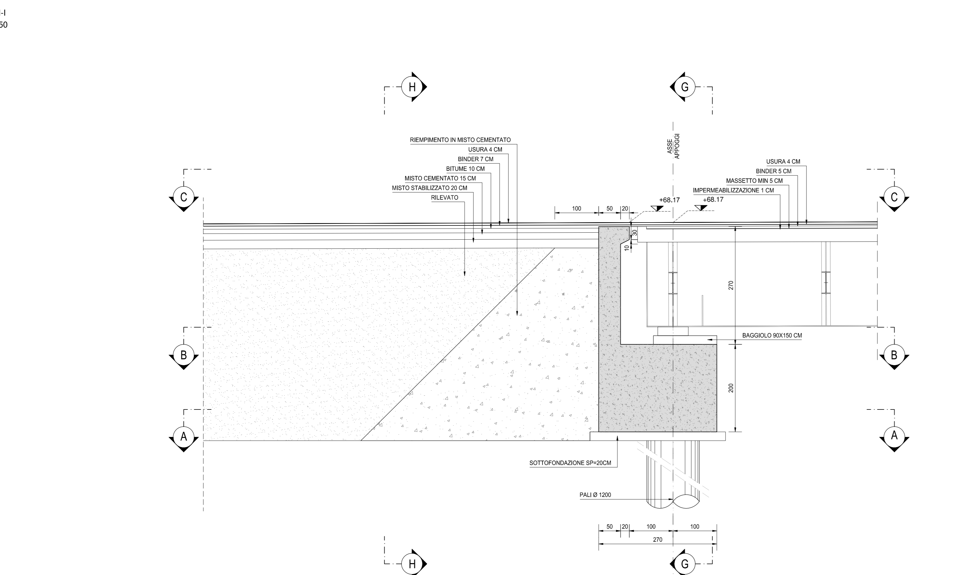
SEZIONE D-D SCALA 1:50
