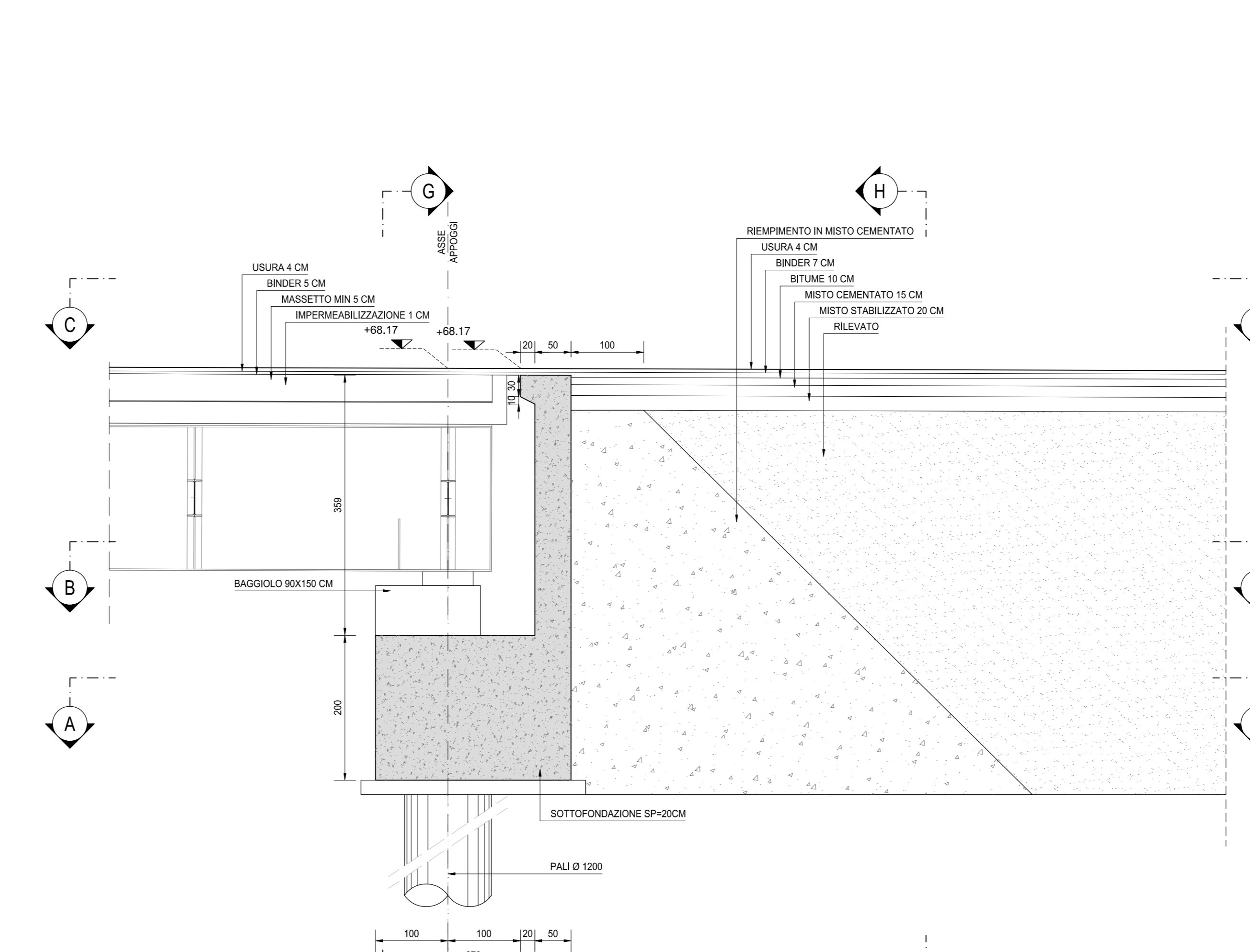
SEZIONE D-D SCALA 1:50
