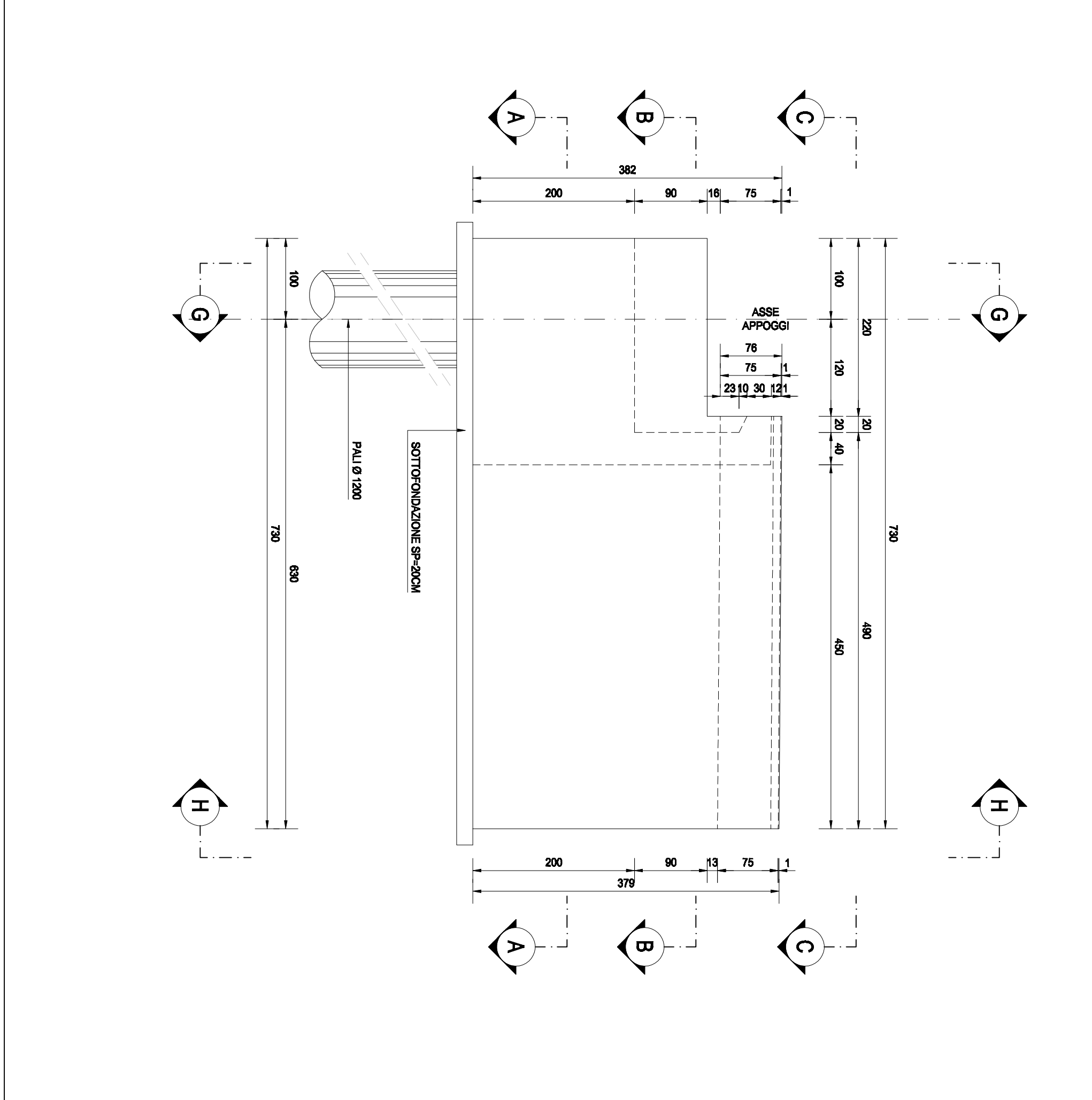
VISTA EE SCALA 1:50
