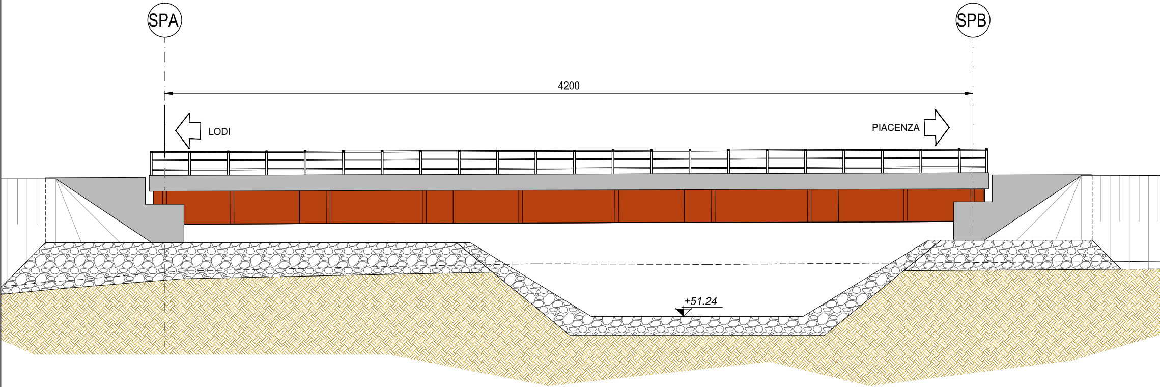
PROSPETTO OVEST SCALA 1:200
