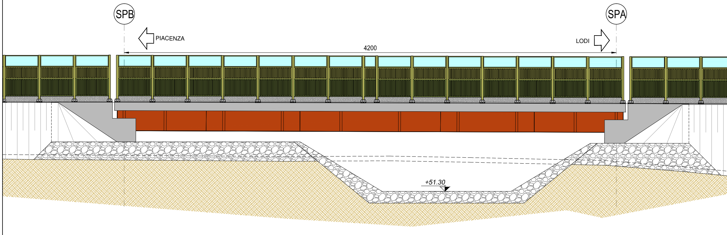
PROSPETTO EST SCALA 1:200
