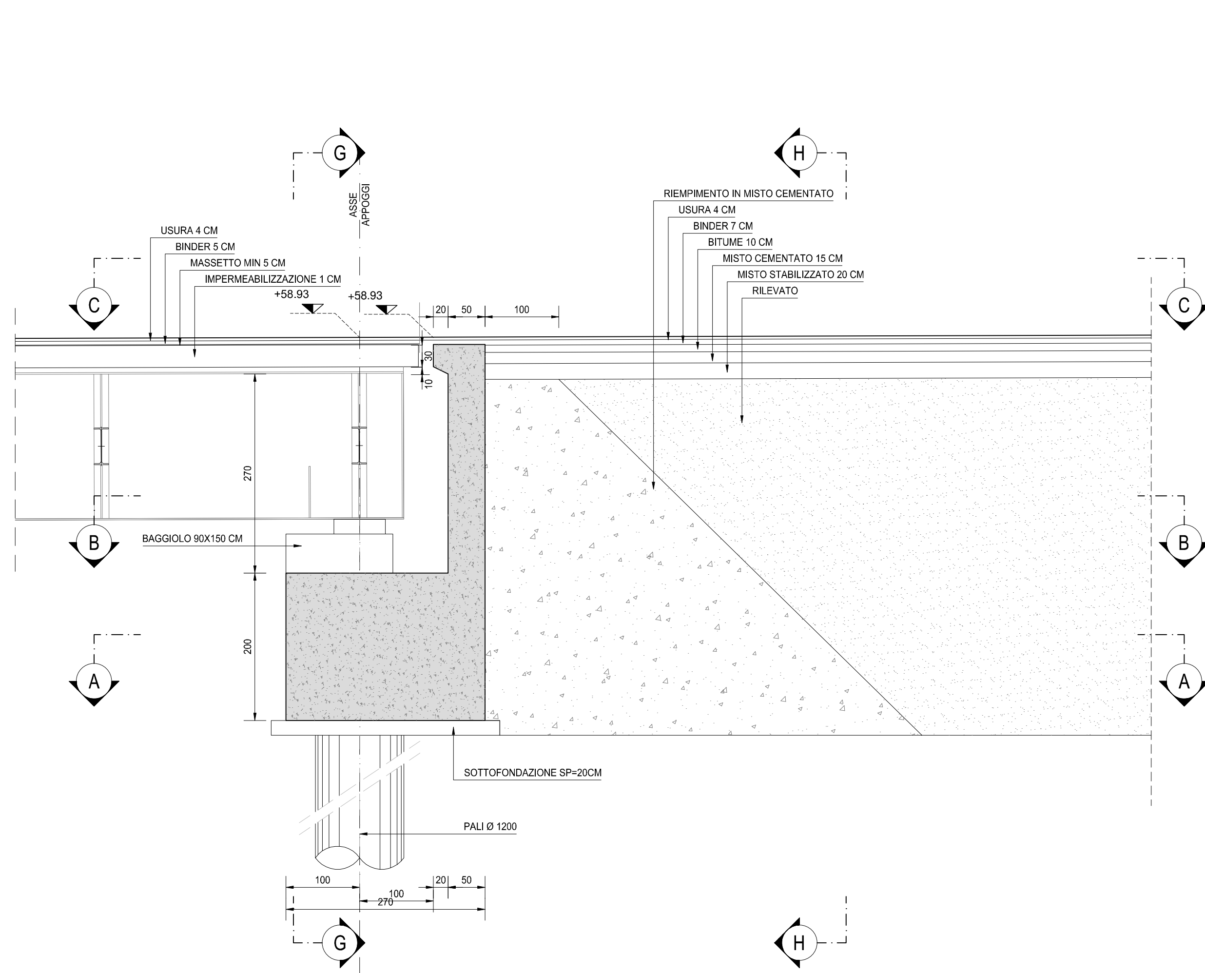
SEZIONE D-D SCALA 1:50
