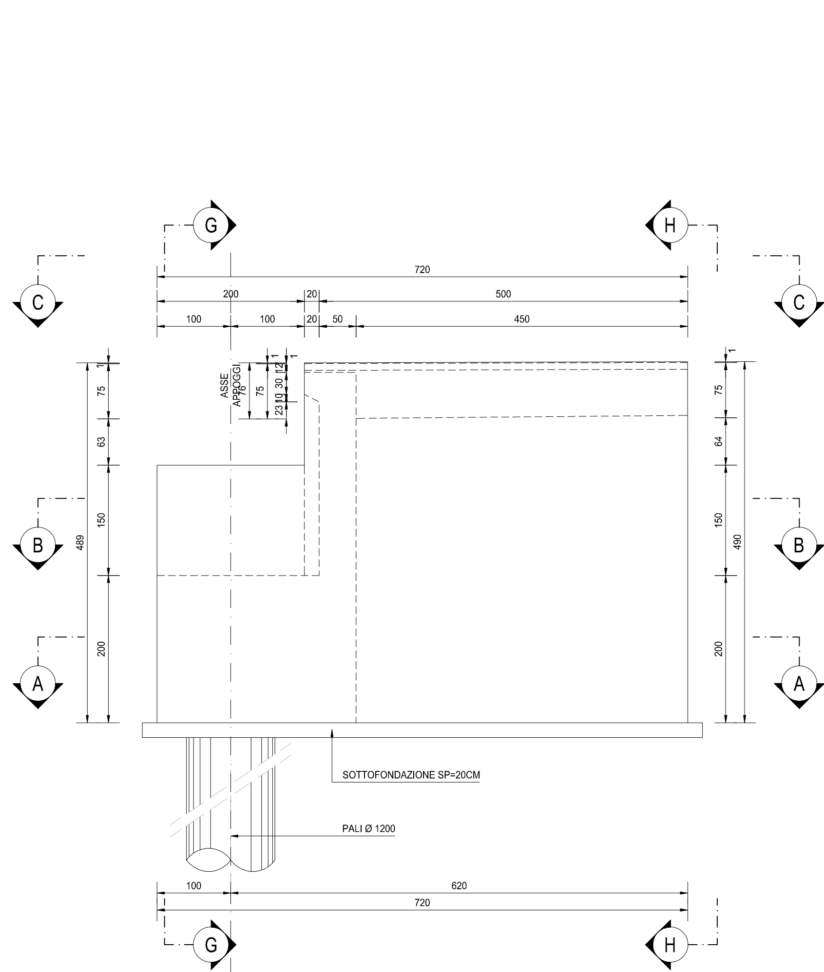
SEZIONE E-E SCALA 1:50
