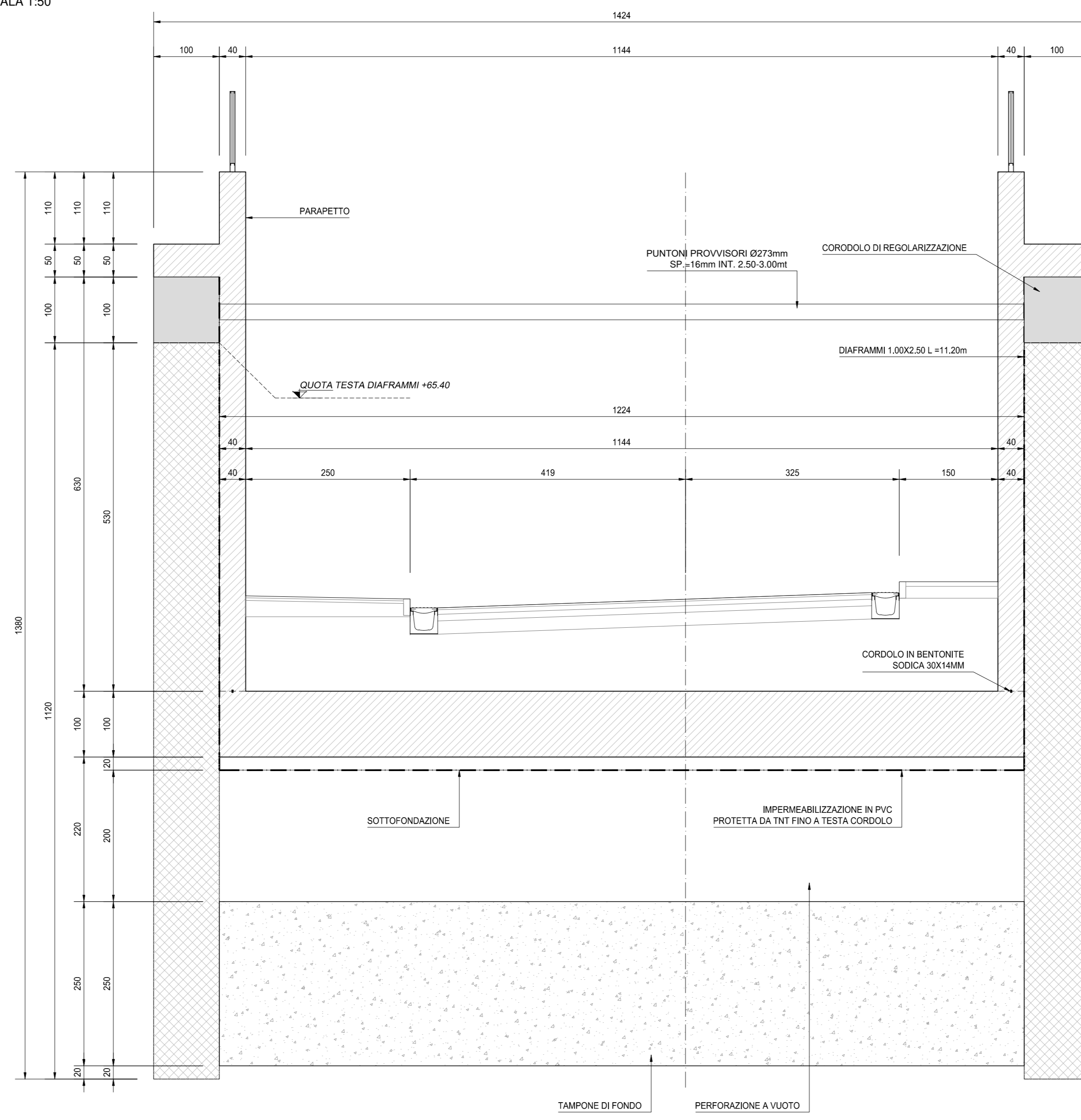
SEZIONE TIPO B - CONCIO 4 - PARTE SCOPERTA SCALA 1:50
