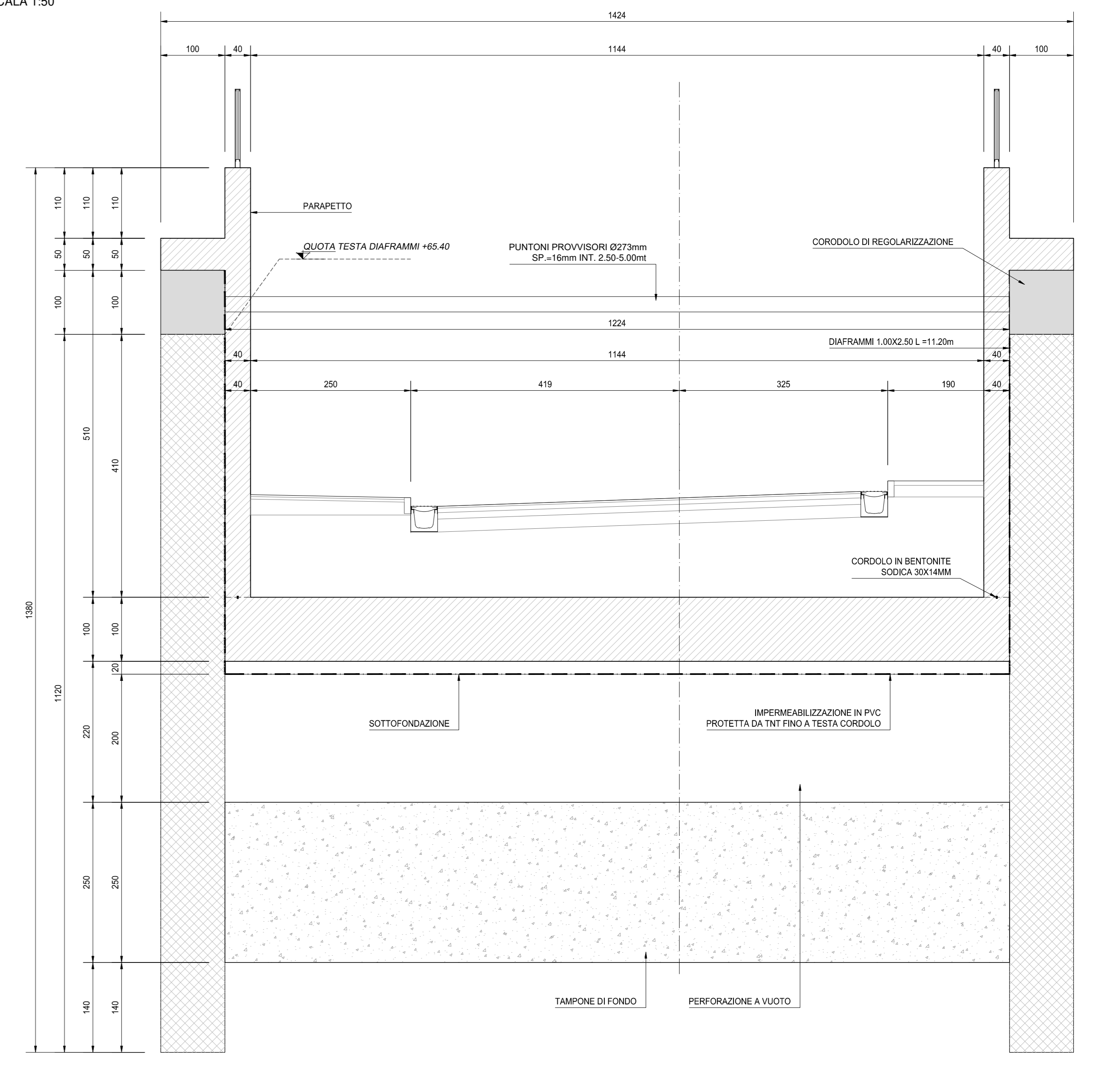
SEZIONE TIPO C - CONCIO 3 SCALA 1:50
