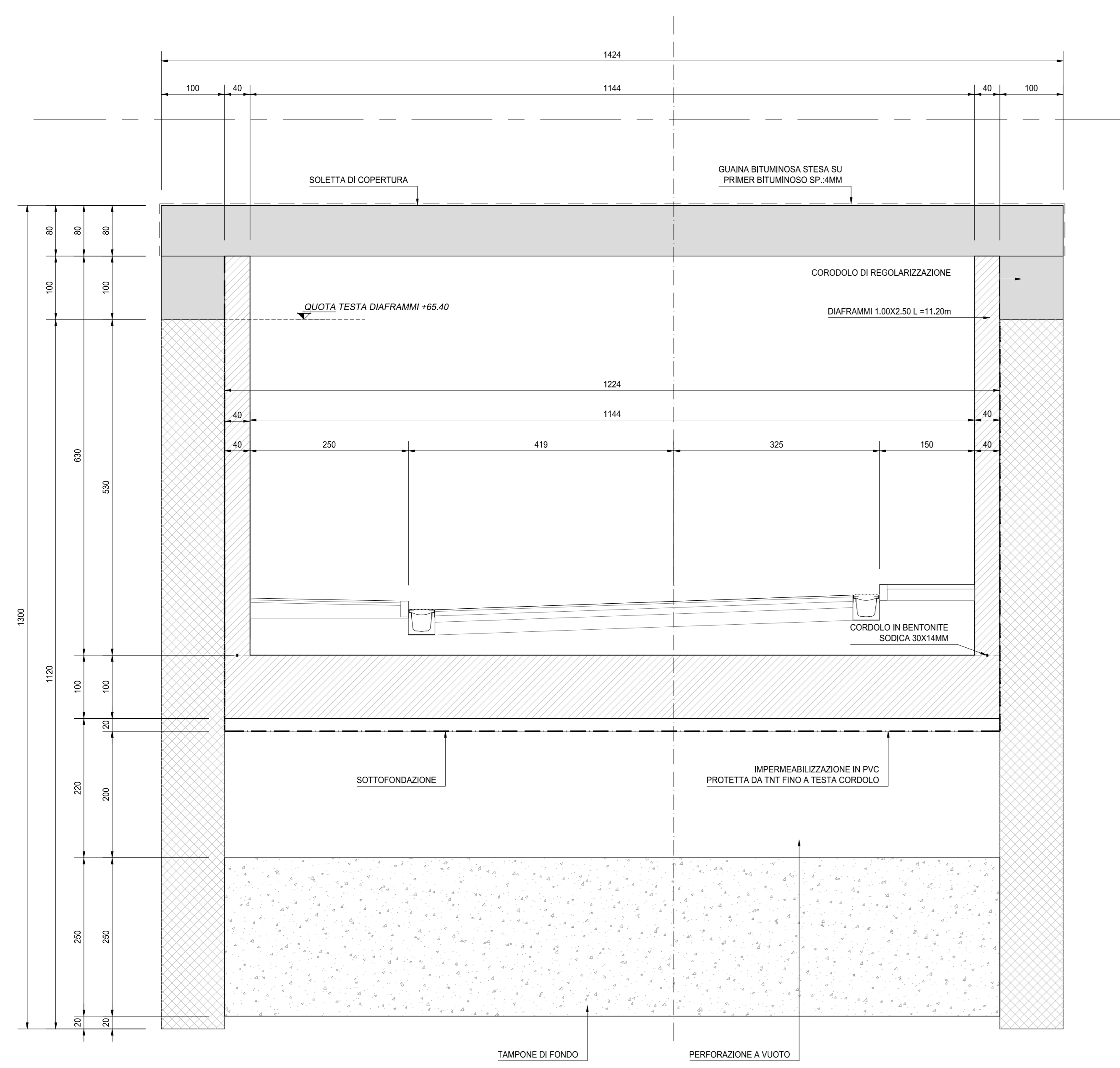
SEZIONE TIPO A - CONCIO 4 - PARTE COPERTA SCALA 1:50
