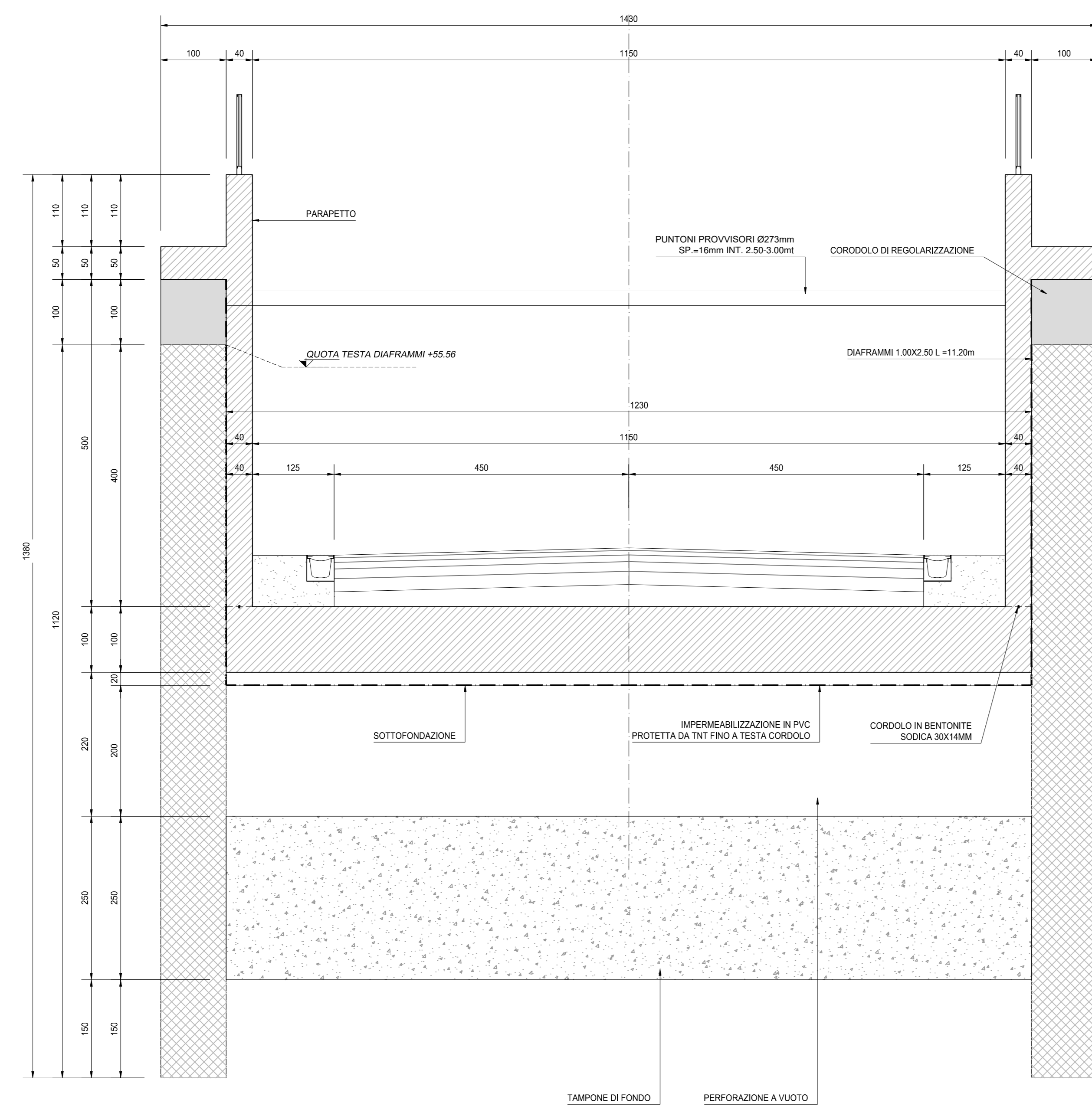
SEZIONE TIPO C - CONCIO 5 SCALA 1:50
