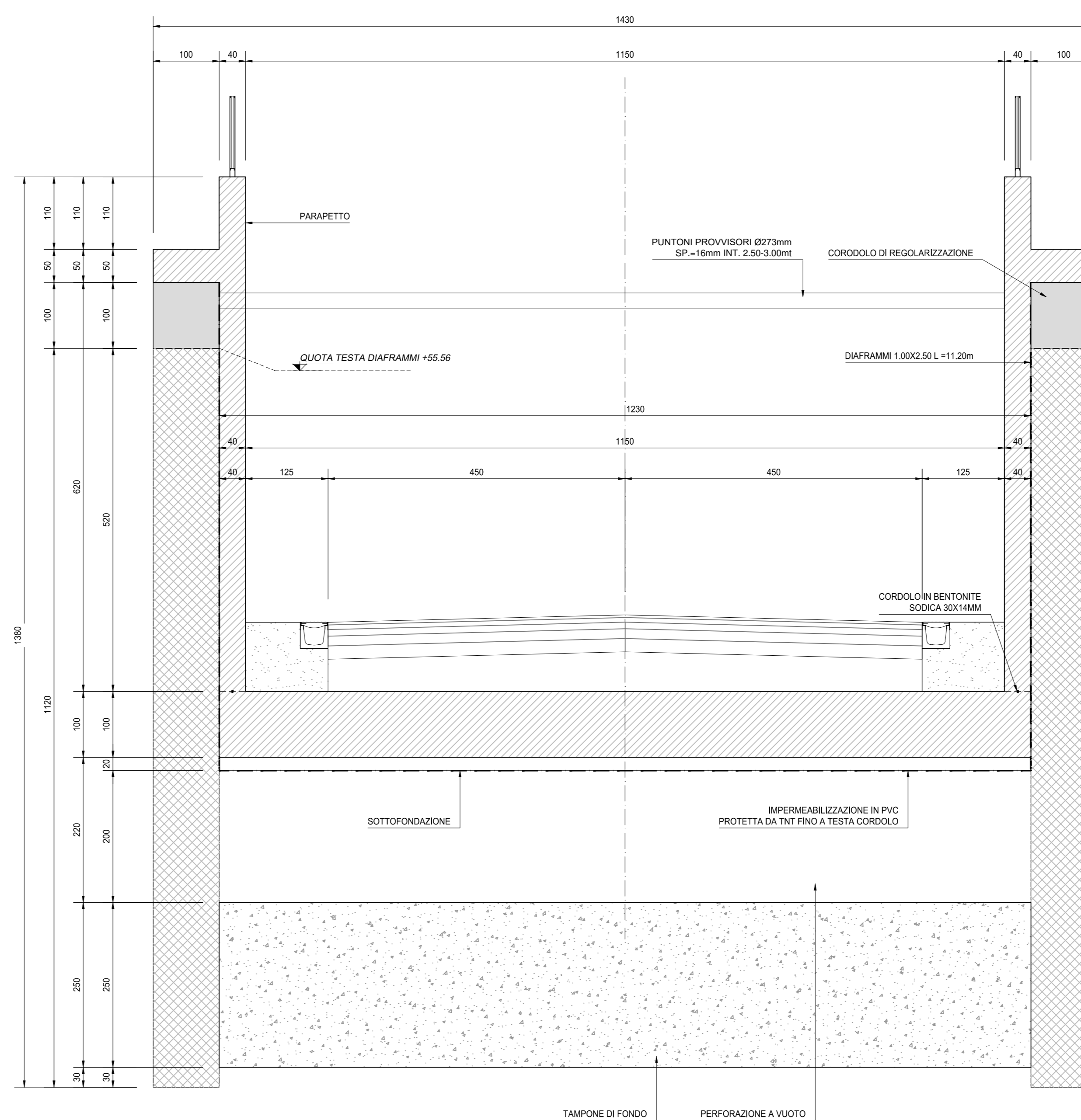
SEZIONE TIPO B - CONCIO 6 - PARTE SCOPERTA SCALA 1:50
