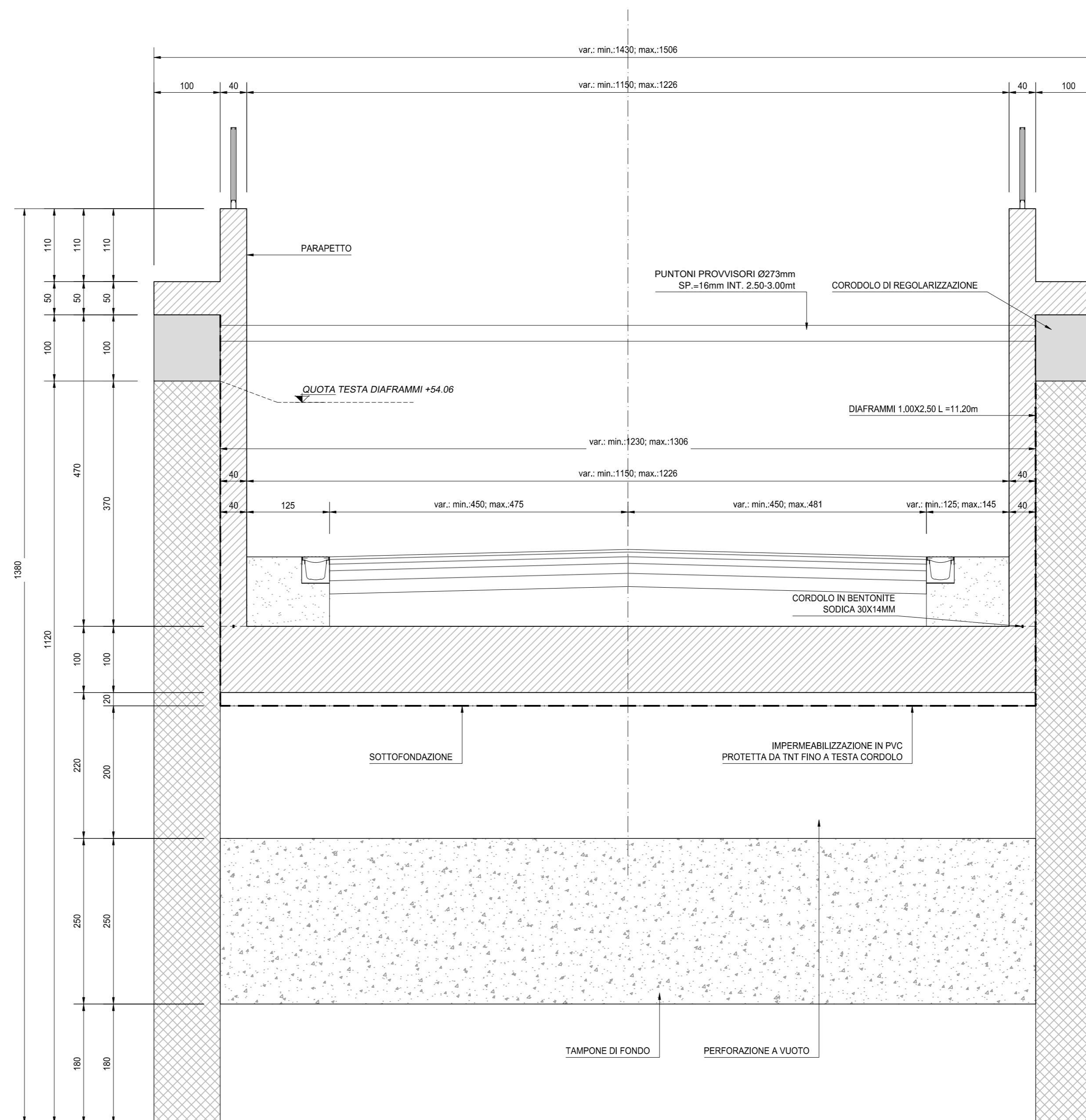
SEZIONE TIPO D - CONCIO 6 - PARTE SCOPERTA SCALA 1:50
