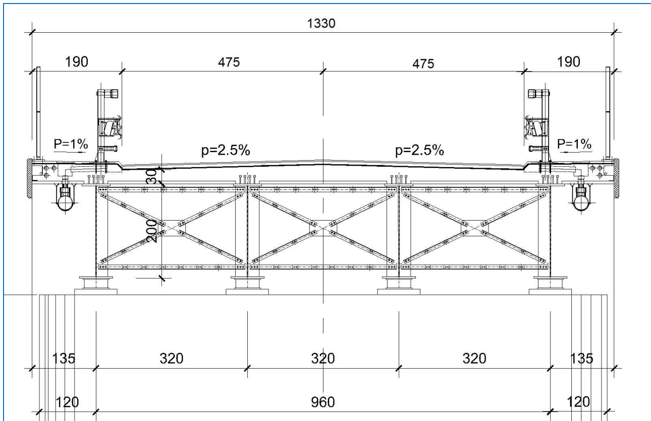
FIGURA 2- SEZIONE IMPALCATO (SU PILA)
