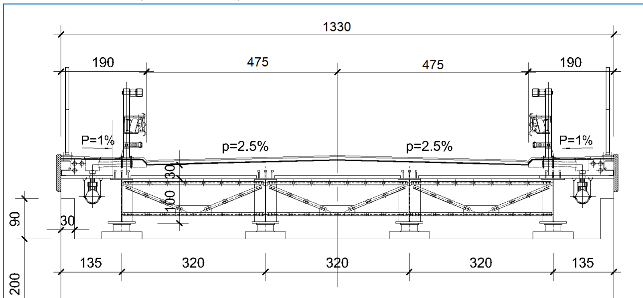
FIGURA 1 - SEZIONE TIPICA IMPALCATO (SU SPALLA)
