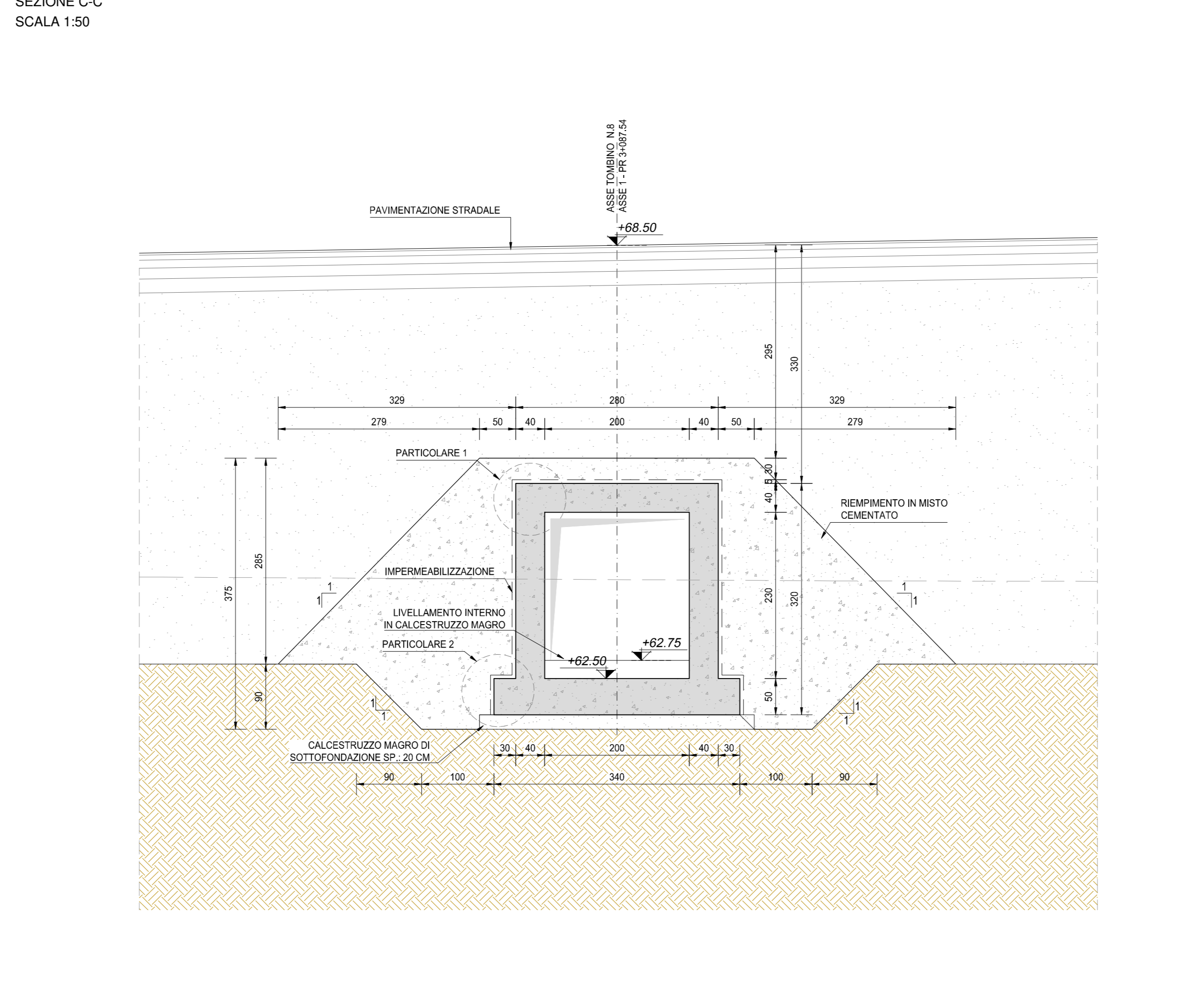
SEZIONE C-C SCALA 1:50
