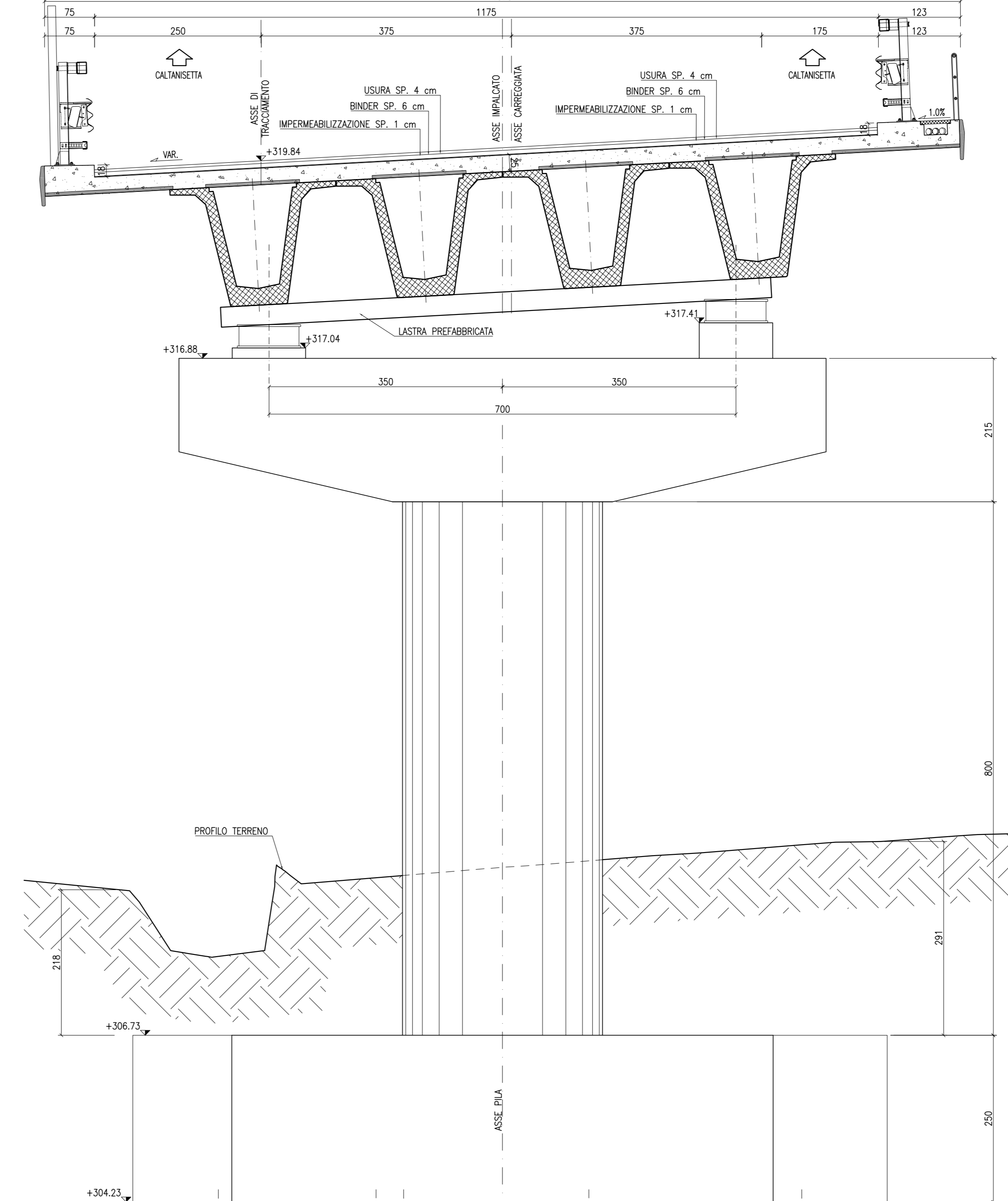
SEZIONE PILA 11 (DESTRA) Progr. 25+499.015 SCALA 1:50
