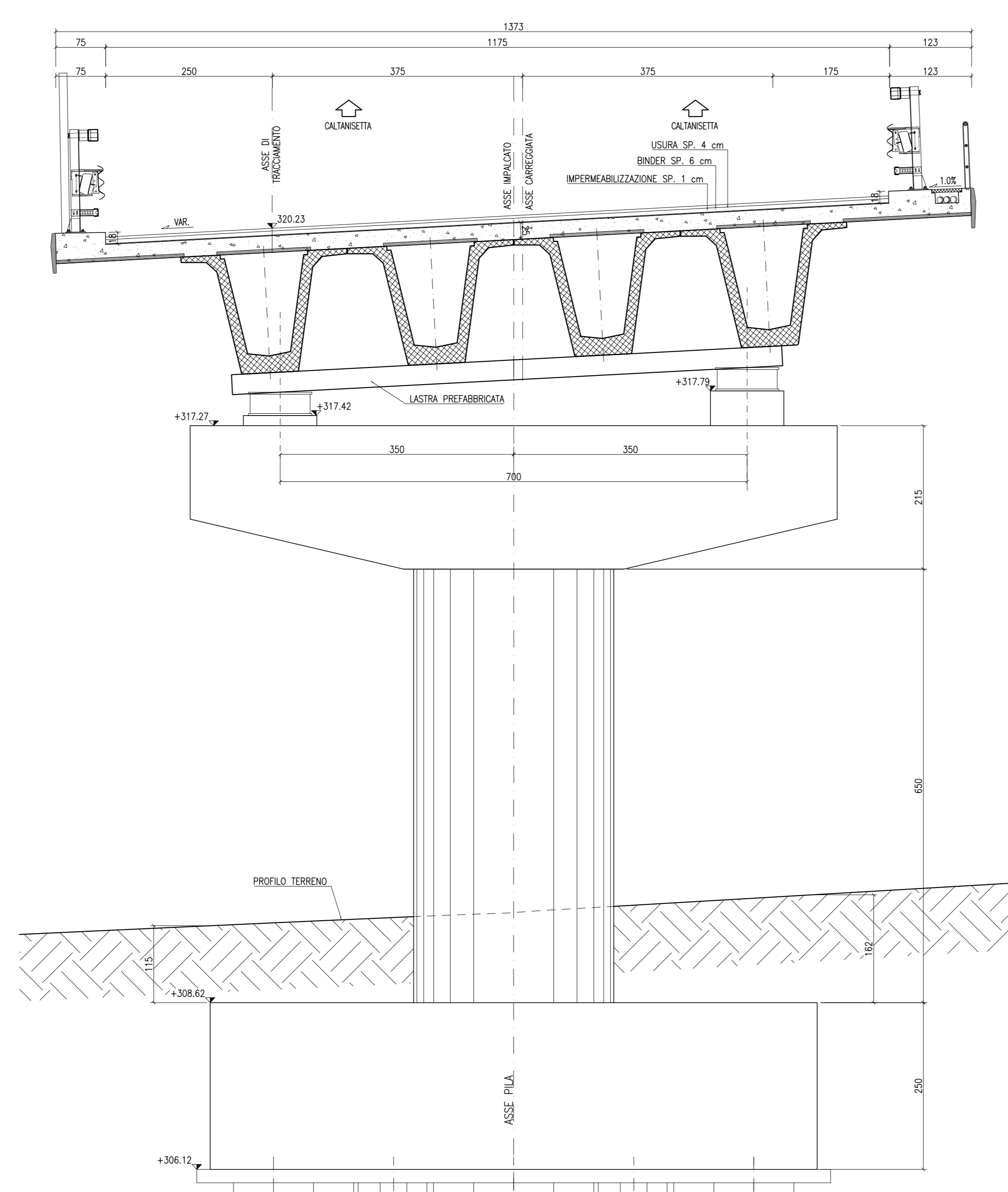
SEZIONE PILA 10 (DESTRA) Progr. 25+468.122 SCALA 1:50
