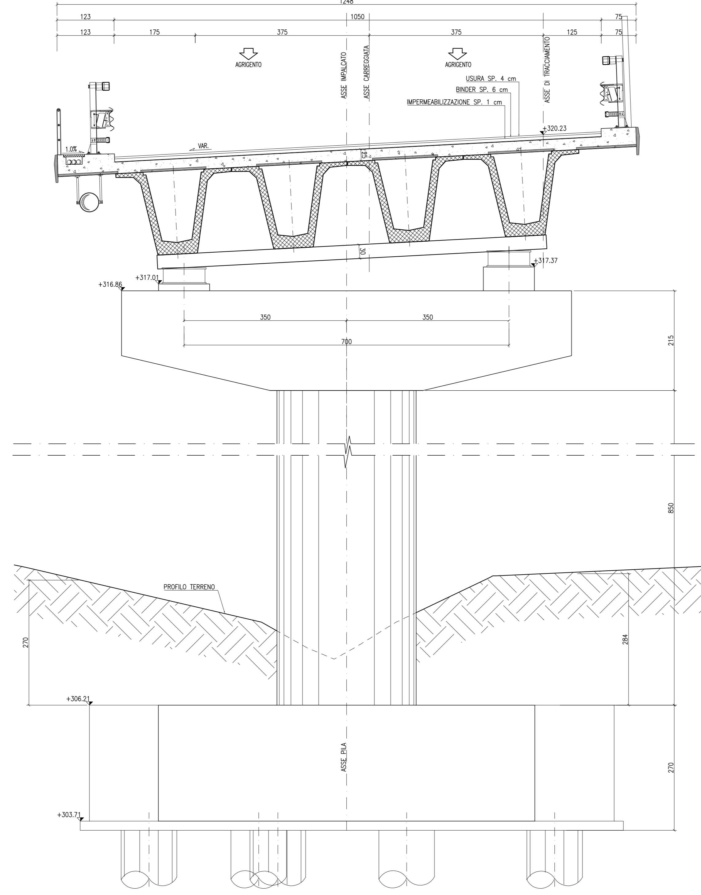
SEZIONE PILA 10 (DESTRA) Progr. 25+468.122 SCALA 1:50
