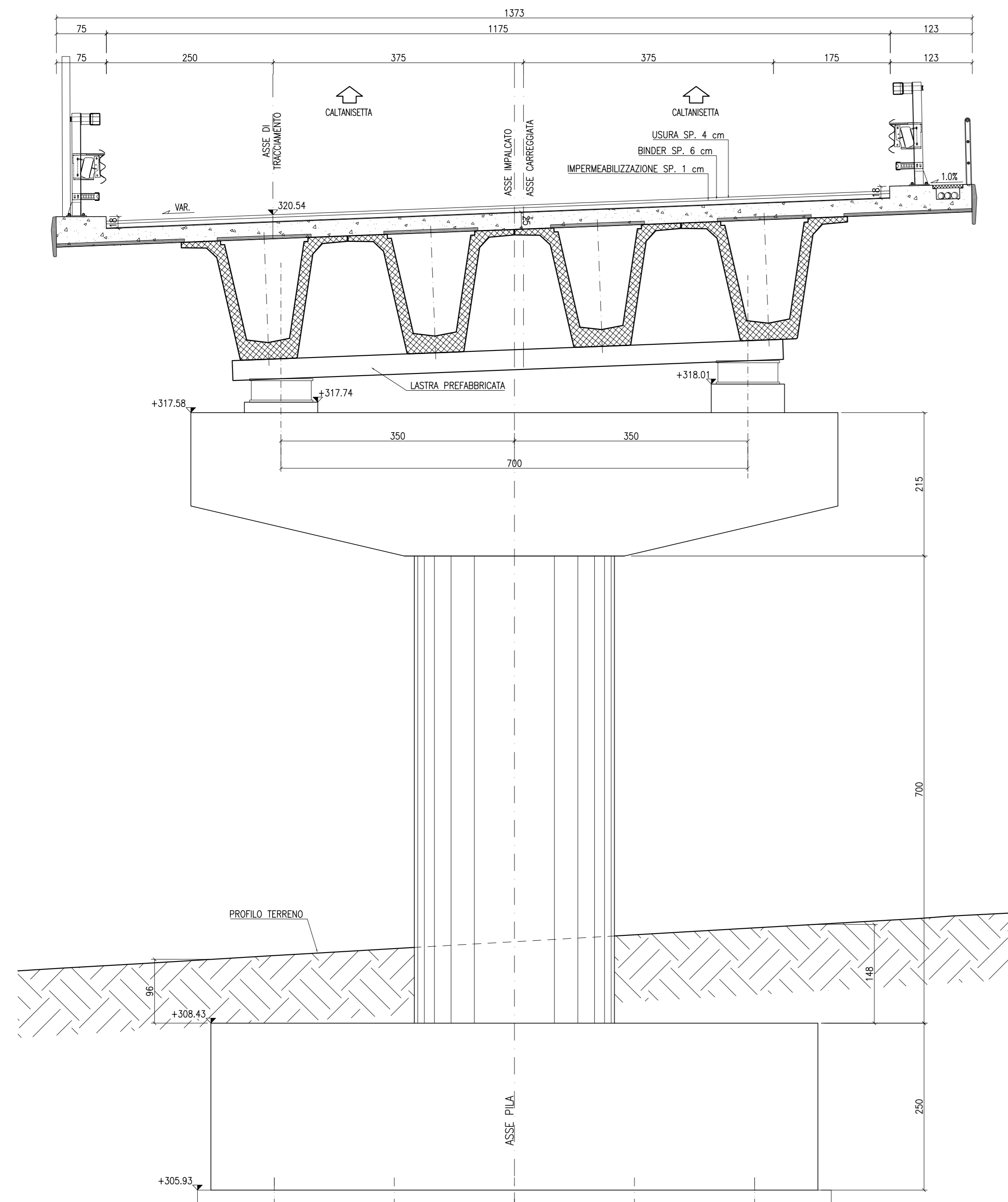
SEZIONE PILA 9 (DESTRA) Progr. 25+438.217 SCALA 1:50
