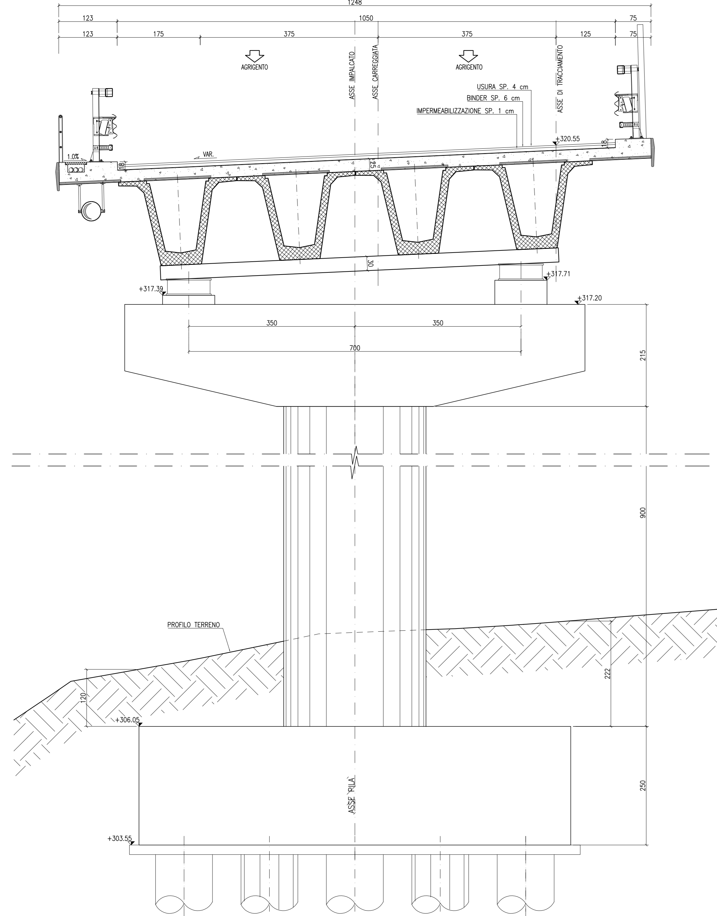
SEZIONE PILA 9 (DESTRA) Progr. 25+438.217 SCALA 1:50
