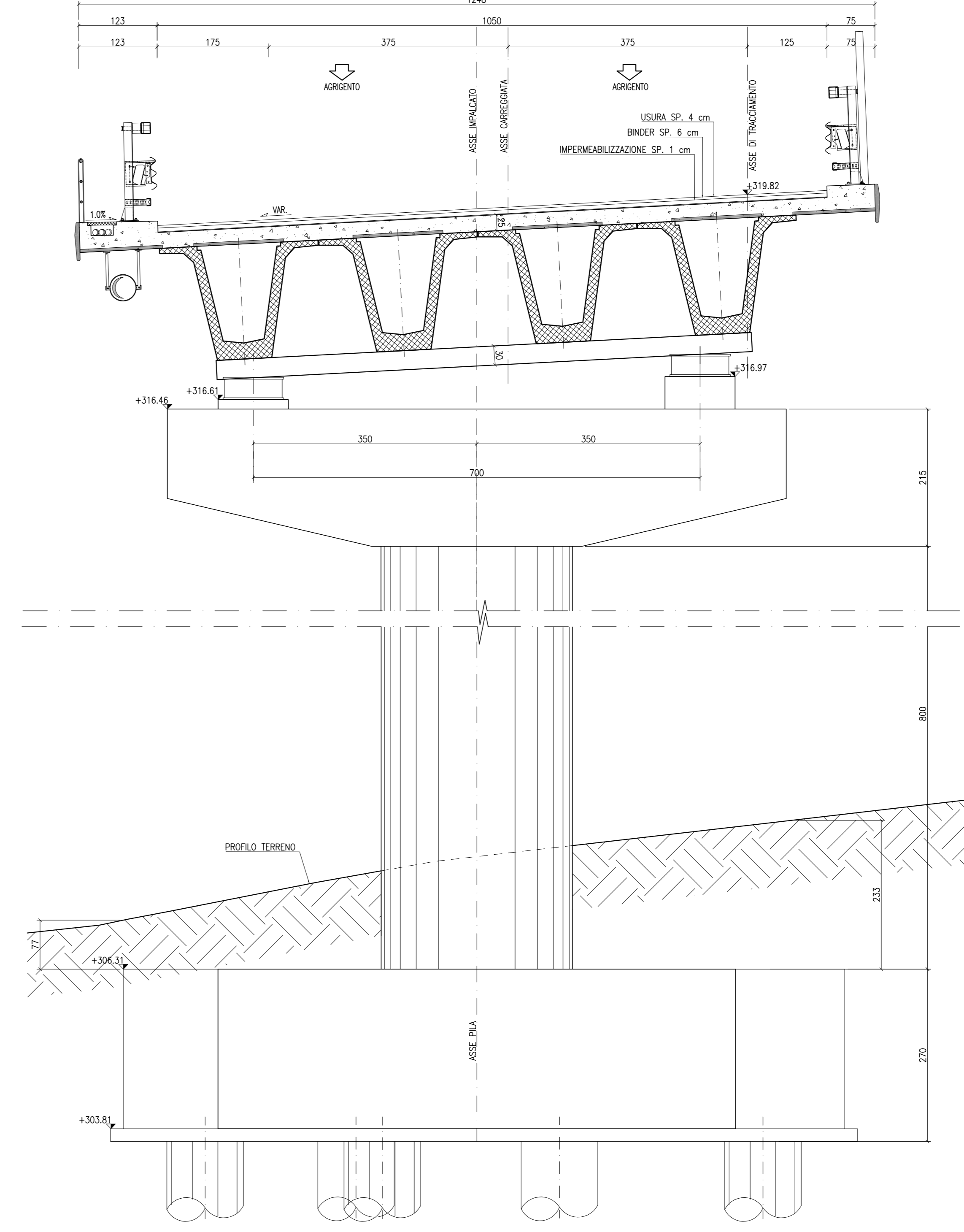
SEZIONE PILA 11 (DESTRA) Progr. 25+499.015 SCALA 1:50
