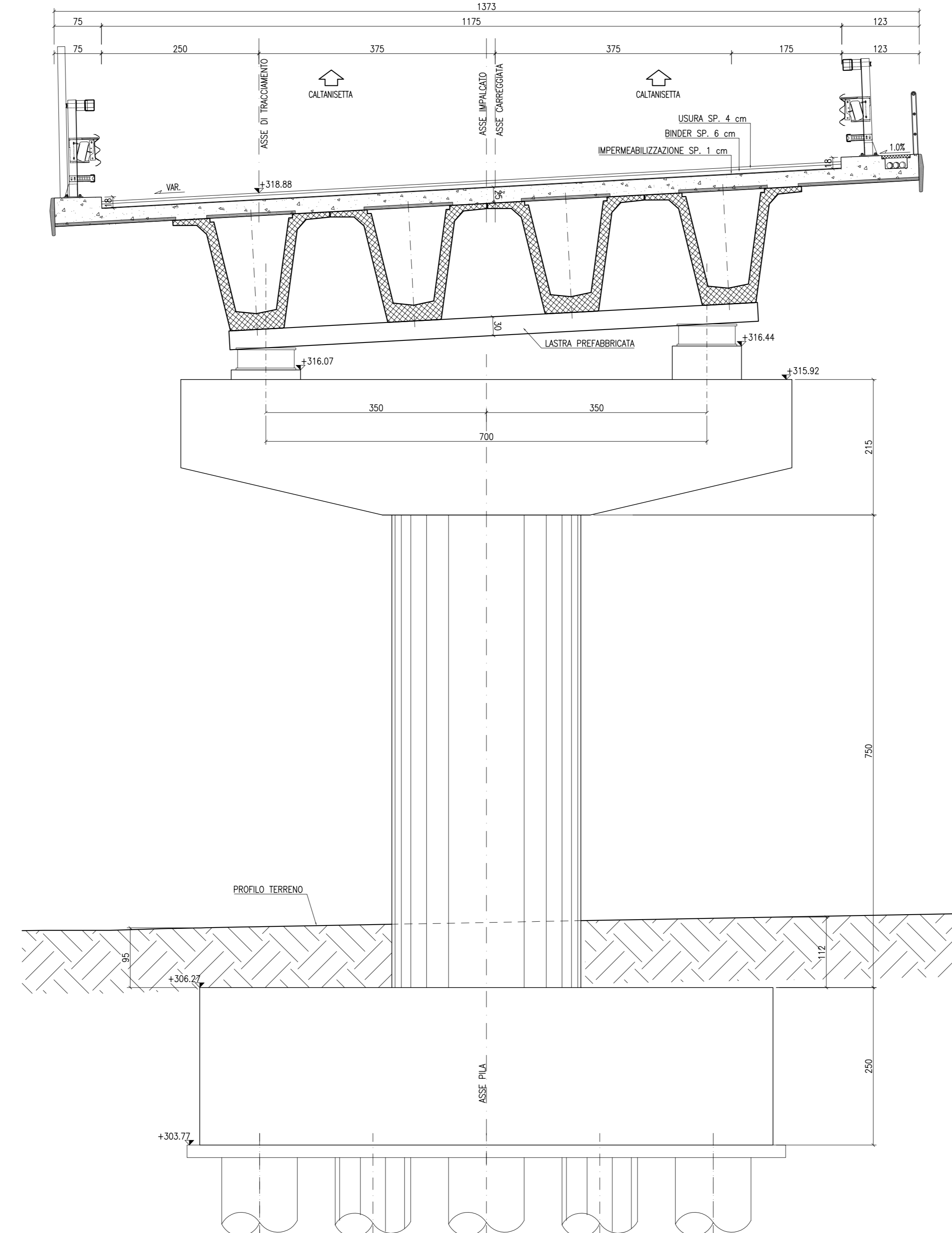
SEZIONE PILA 13 (DESTRA) Progr. 25+560.783 SCALA 1:50
