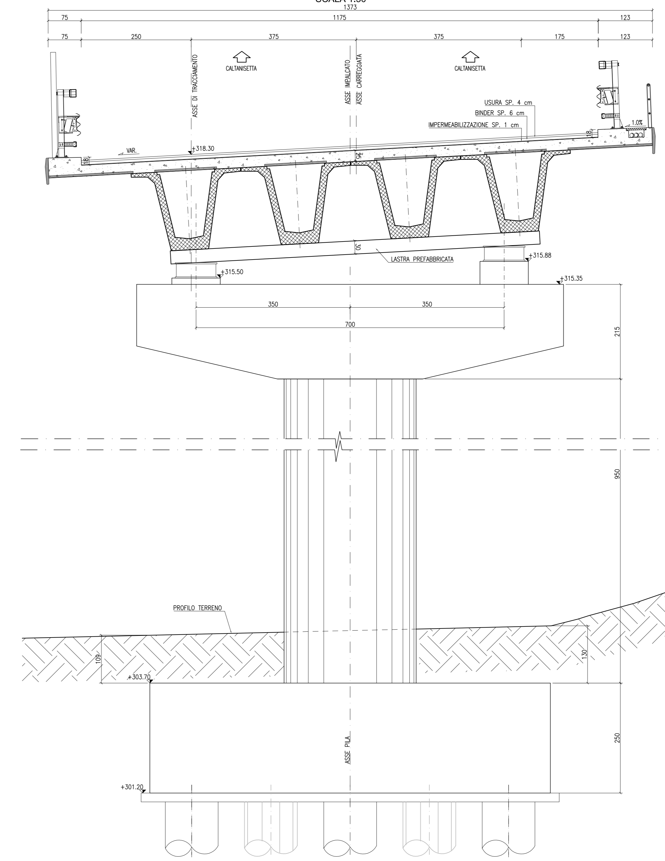
SEZIONE PILA 14 (DESTRA) Progr. 25+591.677 SCALA 1:50
