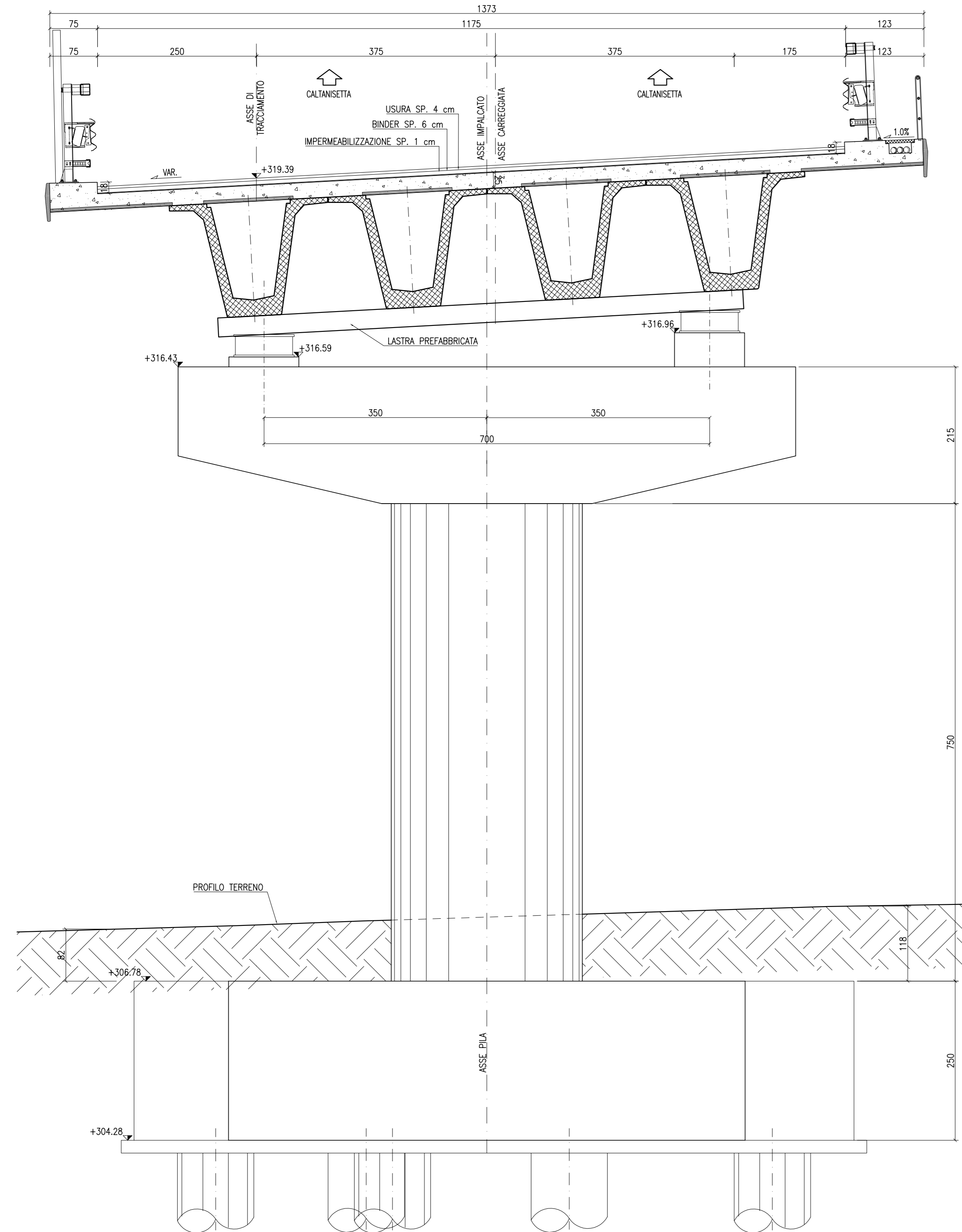
SEZIONE PILA 12 (DESTRA) Progr. 25+529.912 SCALA 1:50
