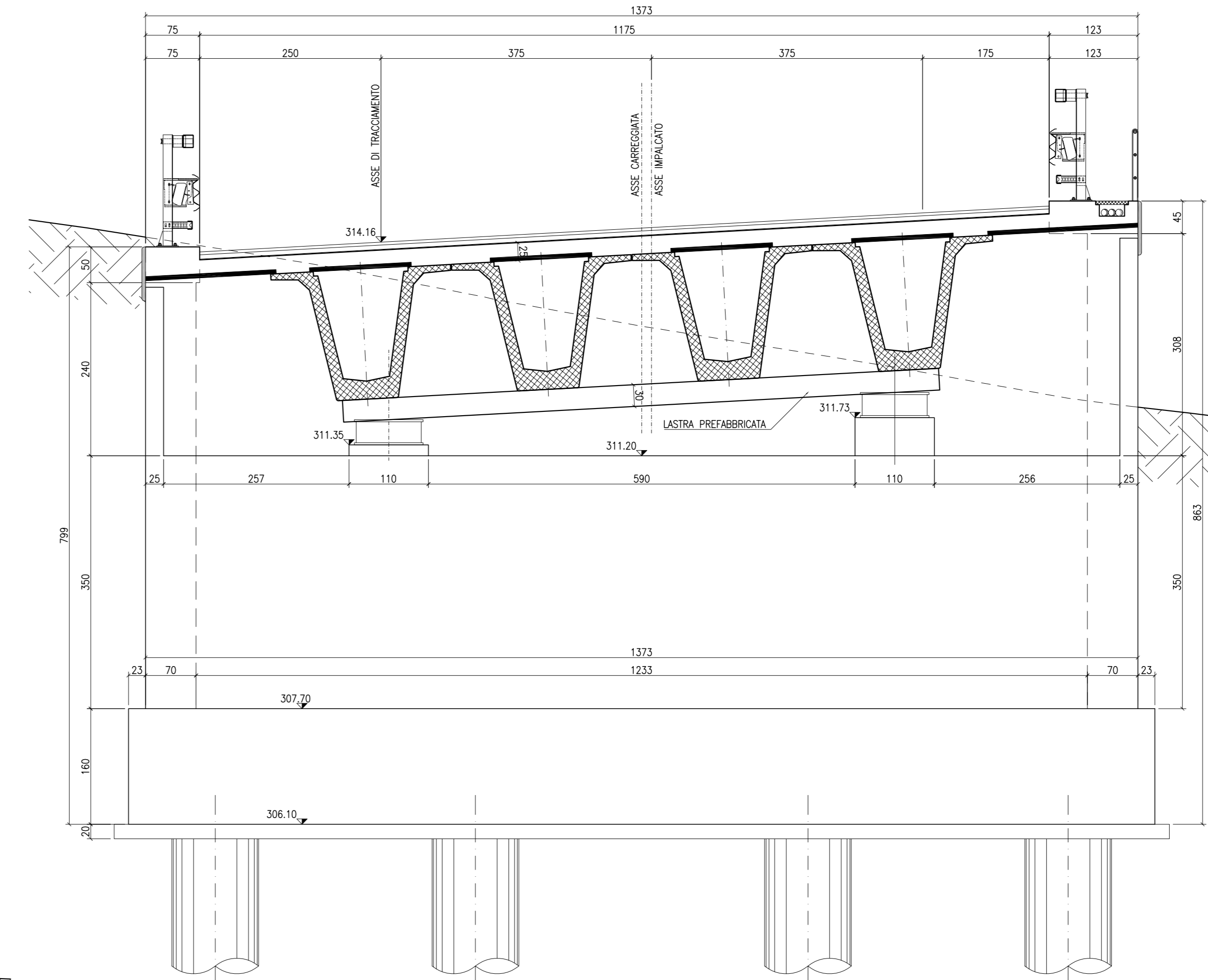
SEZIONE PILA SPB (DESTRA) Progr. 25+776.010 SCALA 1:50
