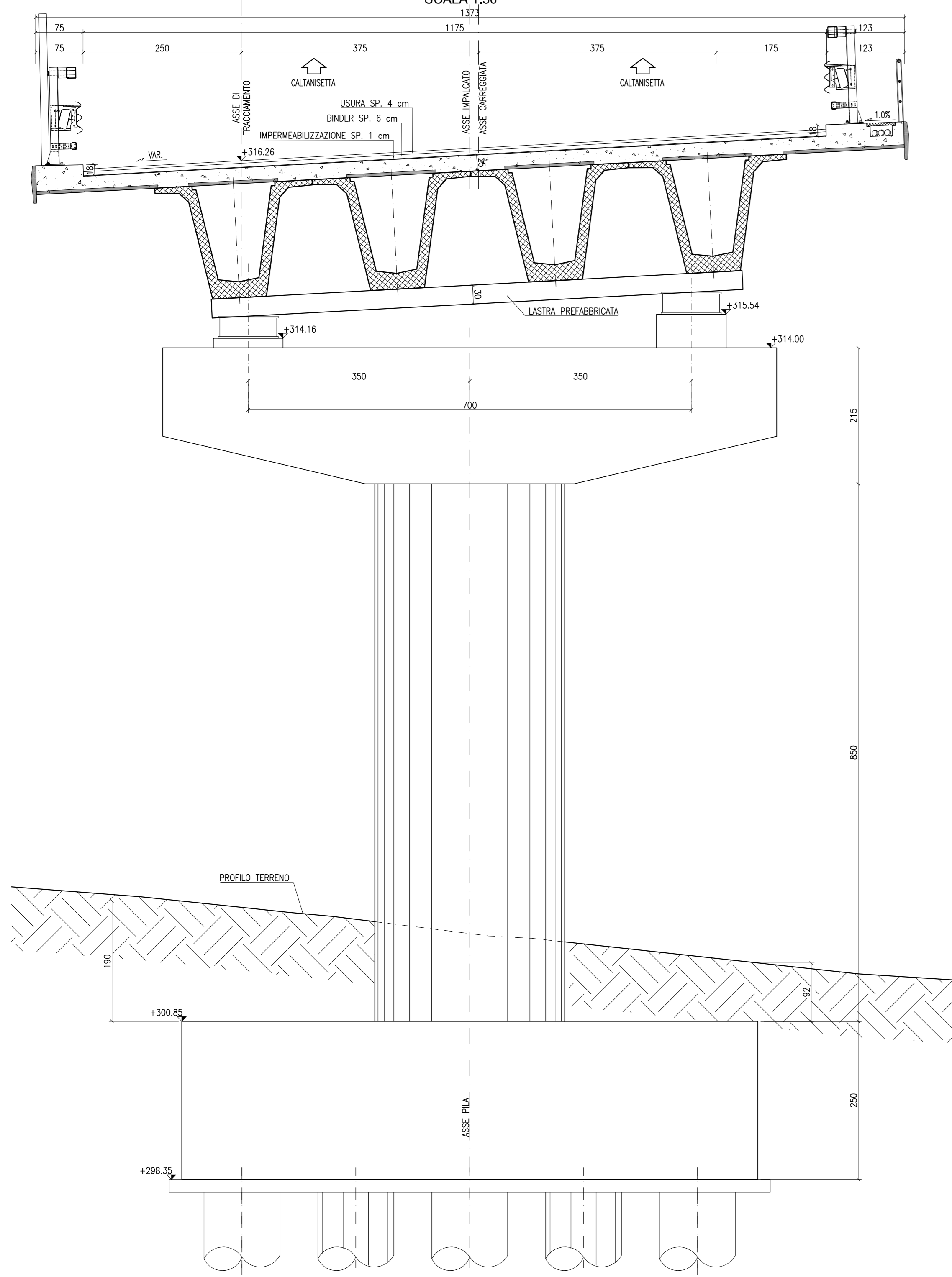
SEZIONE PILA 17 (DESTRA) Progr. 25+684.336 SCALA 1:50
