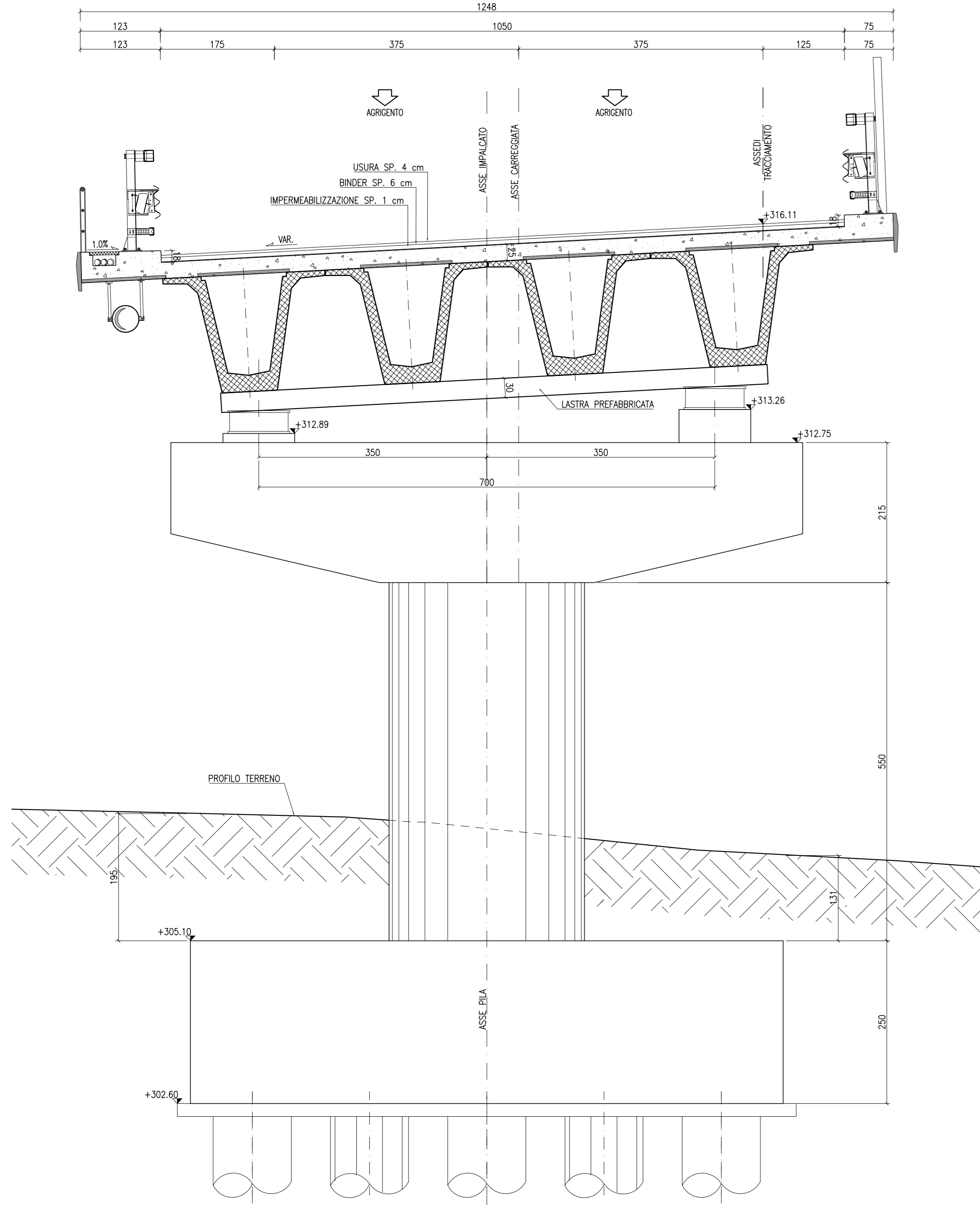
SEZIONE PILA 17 (DESTRA) Progr. 25+684.336 SCALA 1:50
