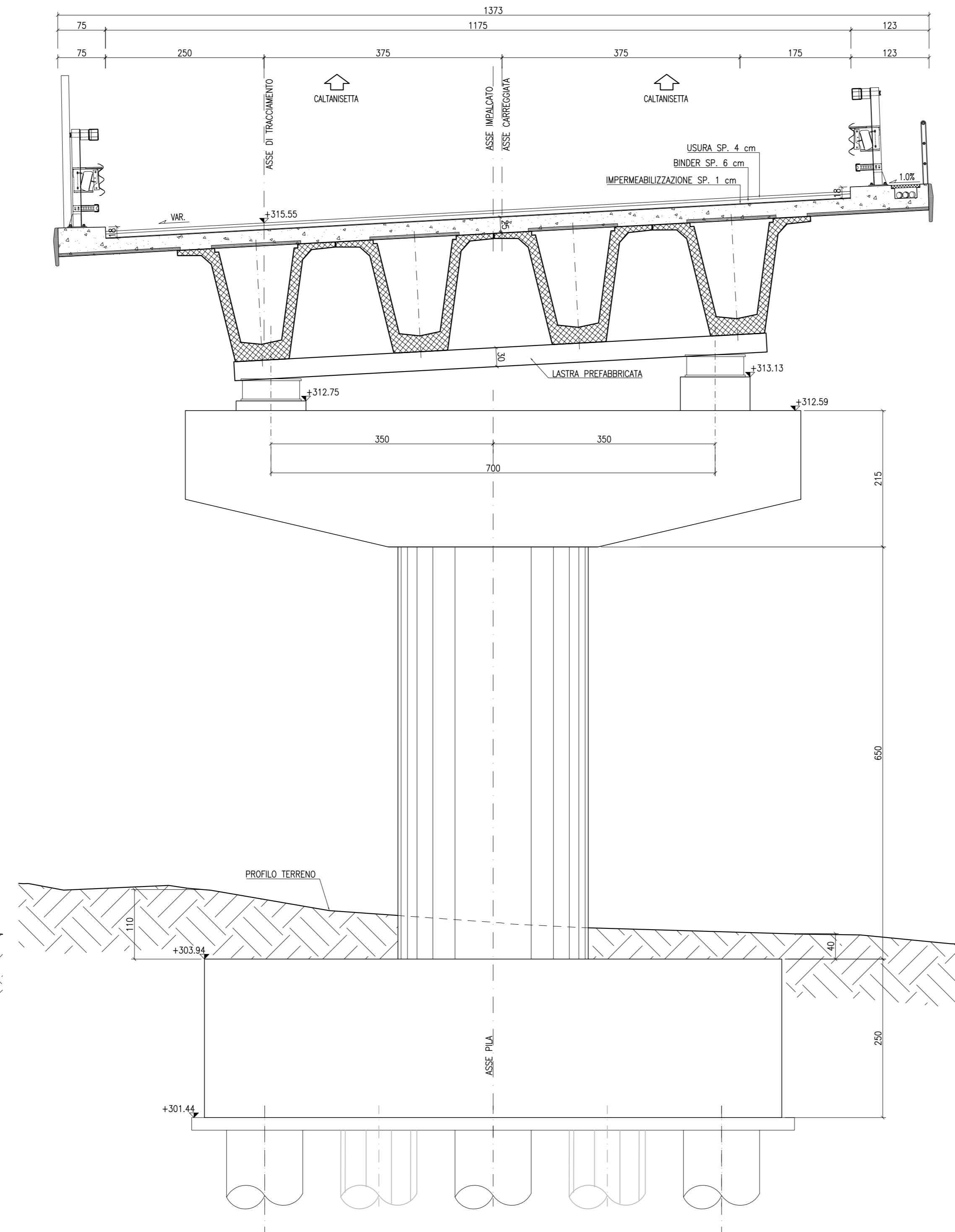
SEZIONE PILA 18 (DESTRA) Progr. 25+715.235 SCALA 1:50
