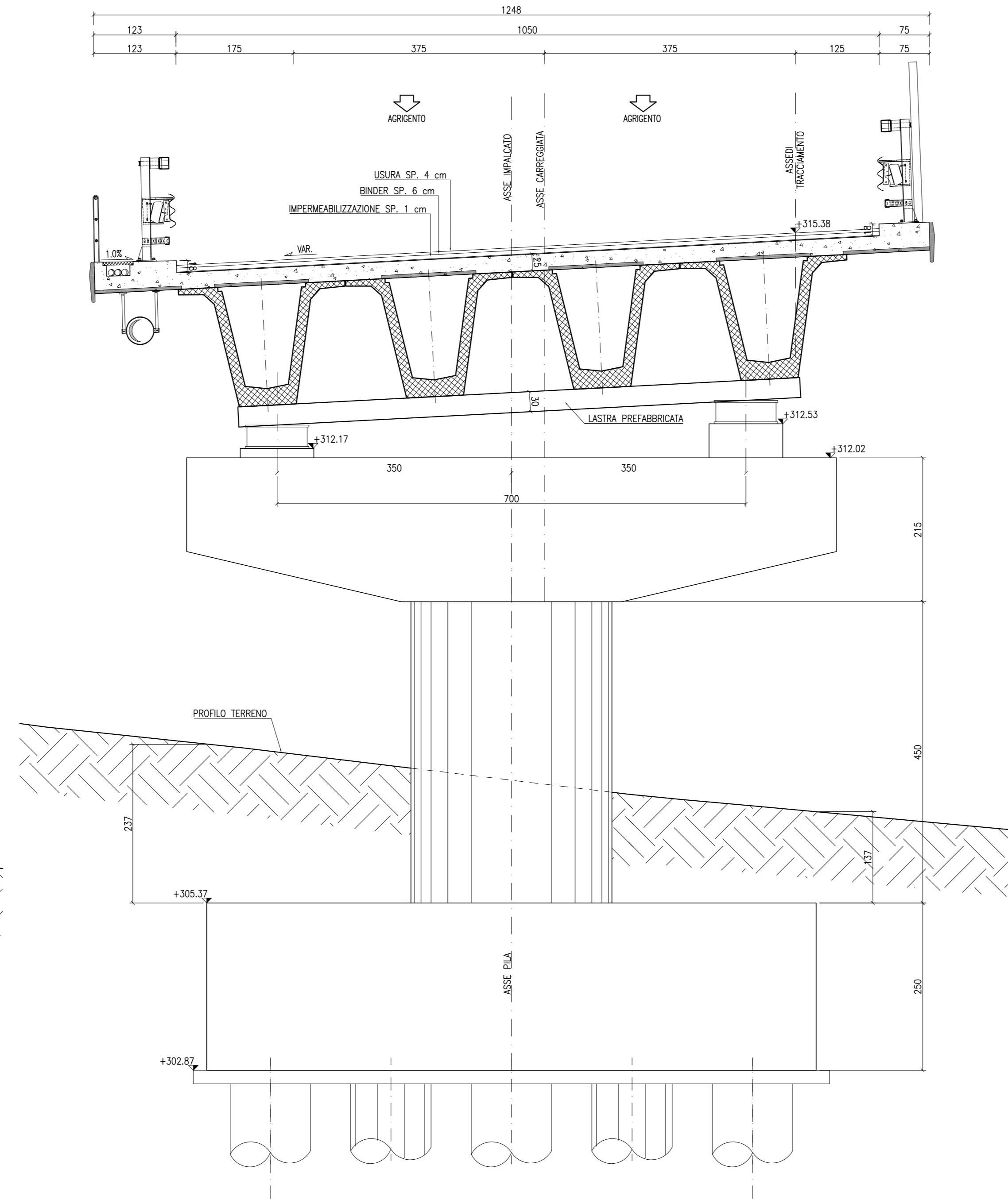
SEZIONE PILA 18 (SINISTRA) Progr. 25+730.369 SCALA 1:50
