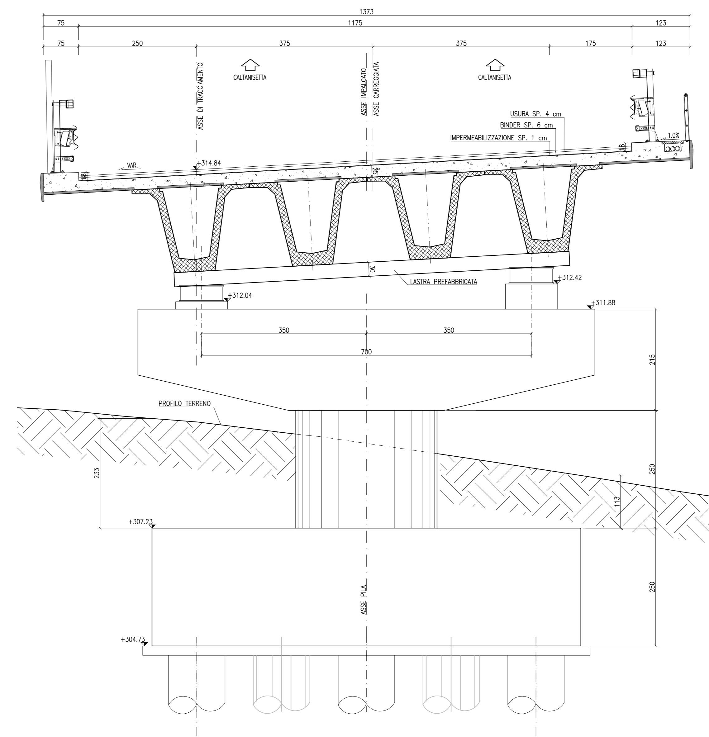
SEZIONE PILA SPB (DESTRA) Progr. 25+776.010 SCALA 1:50
