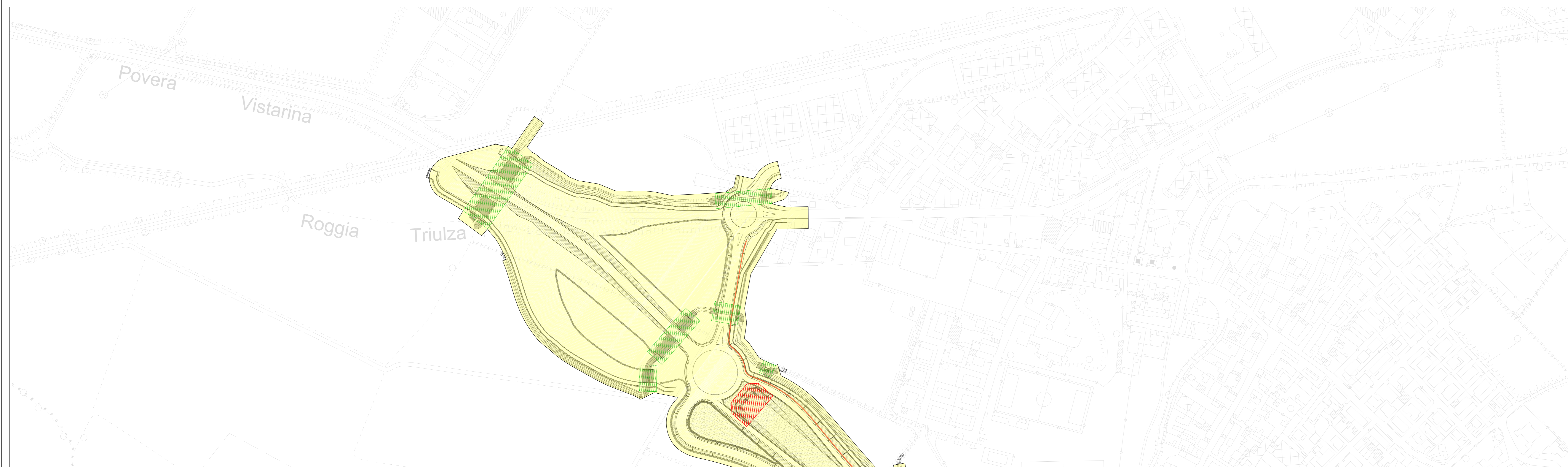
PLANIMETRIA AREE BONIFICA ORDIGNI ESPLOSIVI CON SOVRAPPOSIZIONE PLANIMETRIA DI PROGETTO - TRATTO 01 (SOLO 1° STRALCIO FUNZIONALE) SCALA 1:2.000
