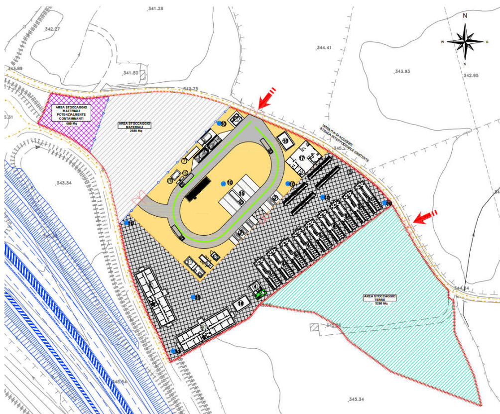
Layout del Campo base
