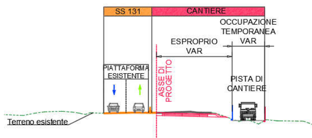
Intervento Fuori Sede Parziale (F.S.P.) – MACROFASE 1 - Sezione trasversale tipologica di cantierizzazione
