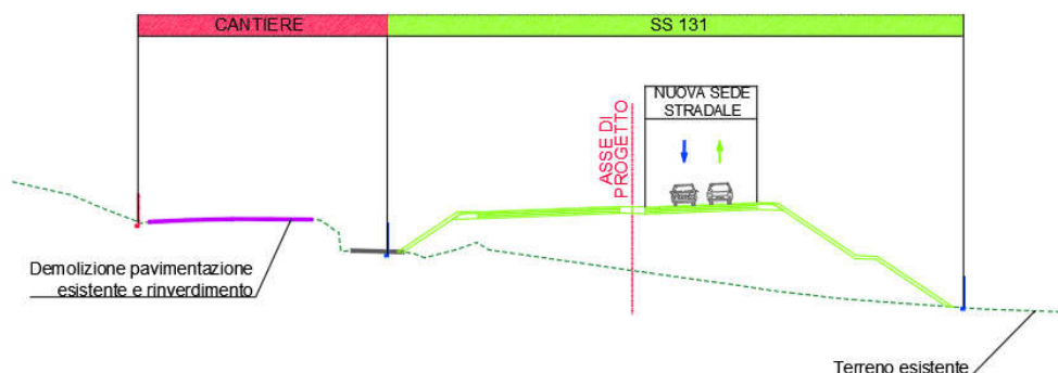
Intervento Fuori Sede (F.S.) – MACROFASE 2 Sezione trasversale tipologica di cantierizzazione
