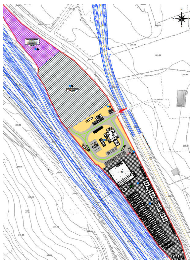
Layout del Campo base
