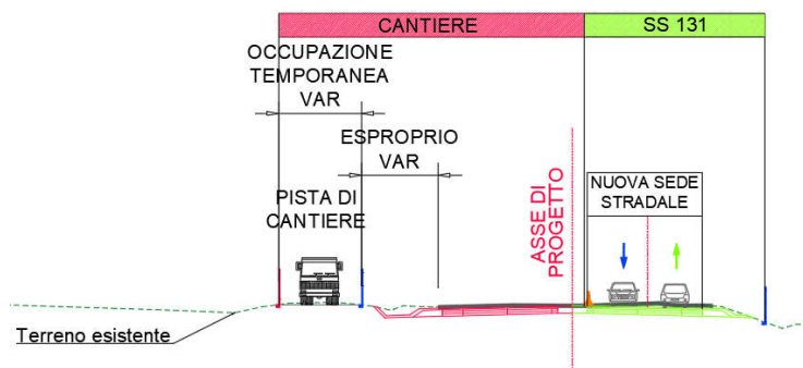
Intervento Fuori Sede Parziale (F.S.P.) – MACROFASE 2 - Sezione trasversale tipologica di cantierizzazione
