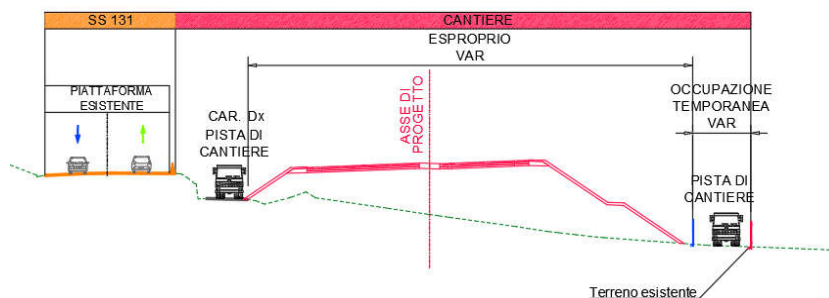
Intervento Fuori Sede (F.S.) – MACROFASE 1 Sezione trasversale tipologica di cantierizzazione
