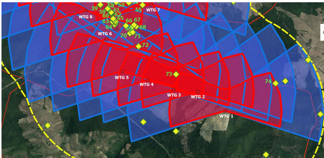
Figura f-2: Effetto della WTG 01 – WTG 02 – WTG 03 – WTG 04 – WTG 05
