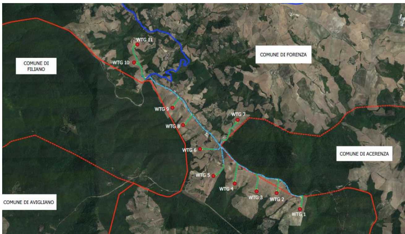
Figura 4: Layout parco eolico e opere di connessione
