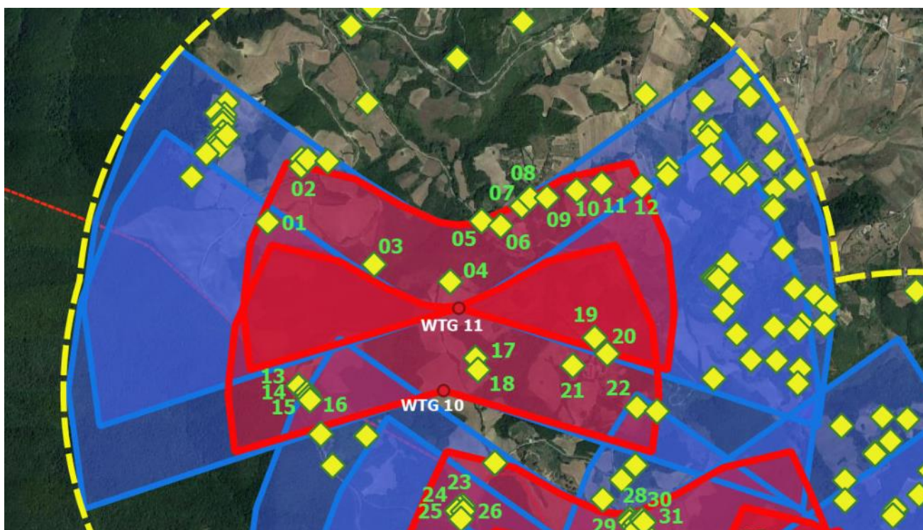
Figura f-4: Effetto della WTG 10 – WTG 11
