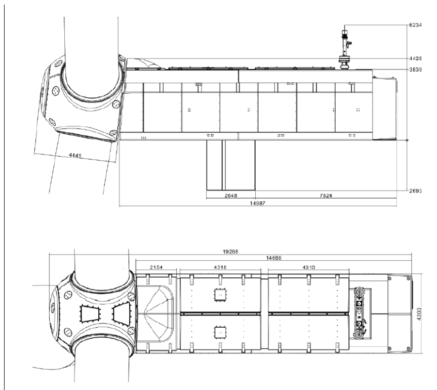
Figura b-2: Tipico navicella WTG
