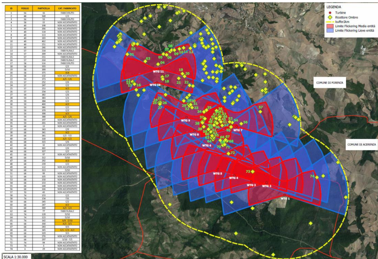
Figura e-1: Recettori all'interno dell'area a effetto flickering di media intensità
