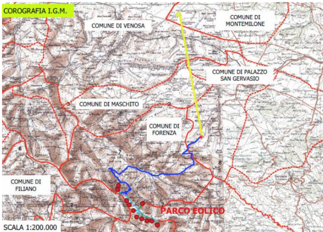
Figura a-1: Inquadramento intervento di area vasta
