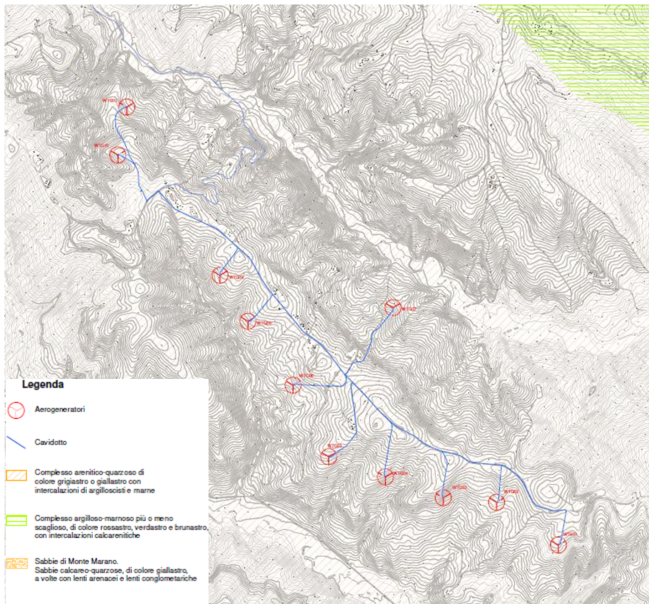
Figura f-1: Stralcio Carta Geologica
