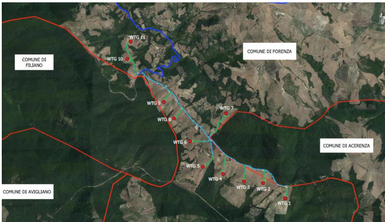
Figura a-4: Area di intervento: dettaglio layout di progetto su ortofoto
