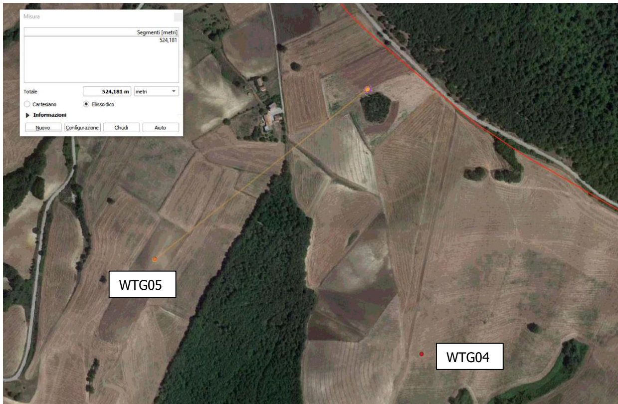
Figura 4-5: Distanza della WTG05 dal minieolico in esercizio.
