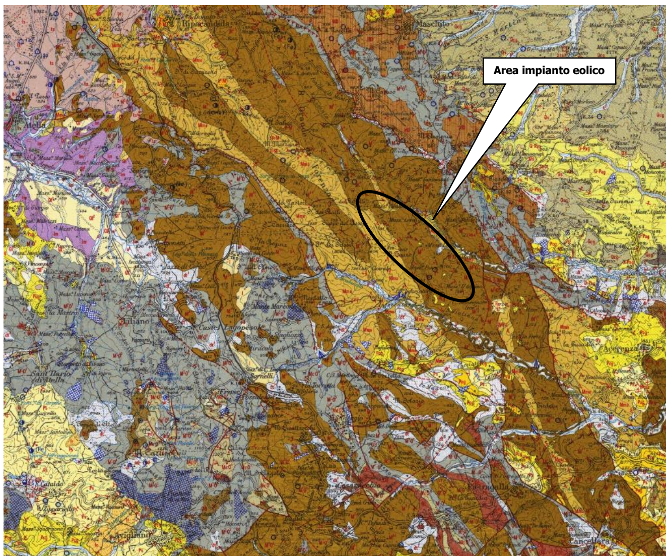
Figura 2-14: Stralcio Carta Geologica d'Italia – Foglio 187 "Melfi"
