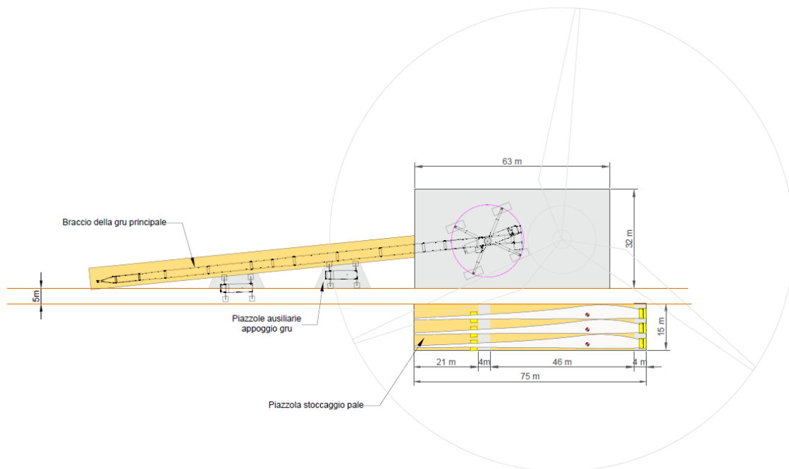
Figura 1 - Schema piazzola in fase di cantiere per il montaggio dell'aerogeneratore
