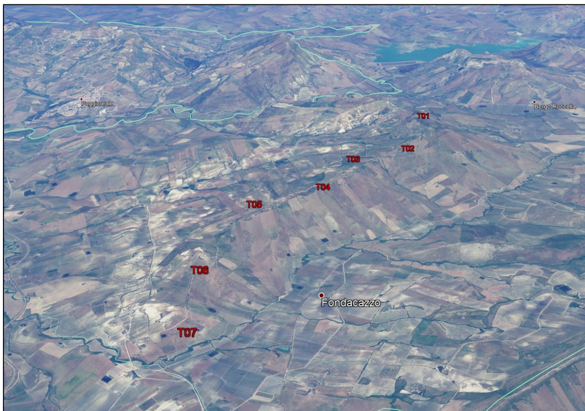
Figura 4: Individuazione degli aerogeneratori di progetto (etichette in rosso) su ortofoto 3D con vista da Sud verso Nord.
