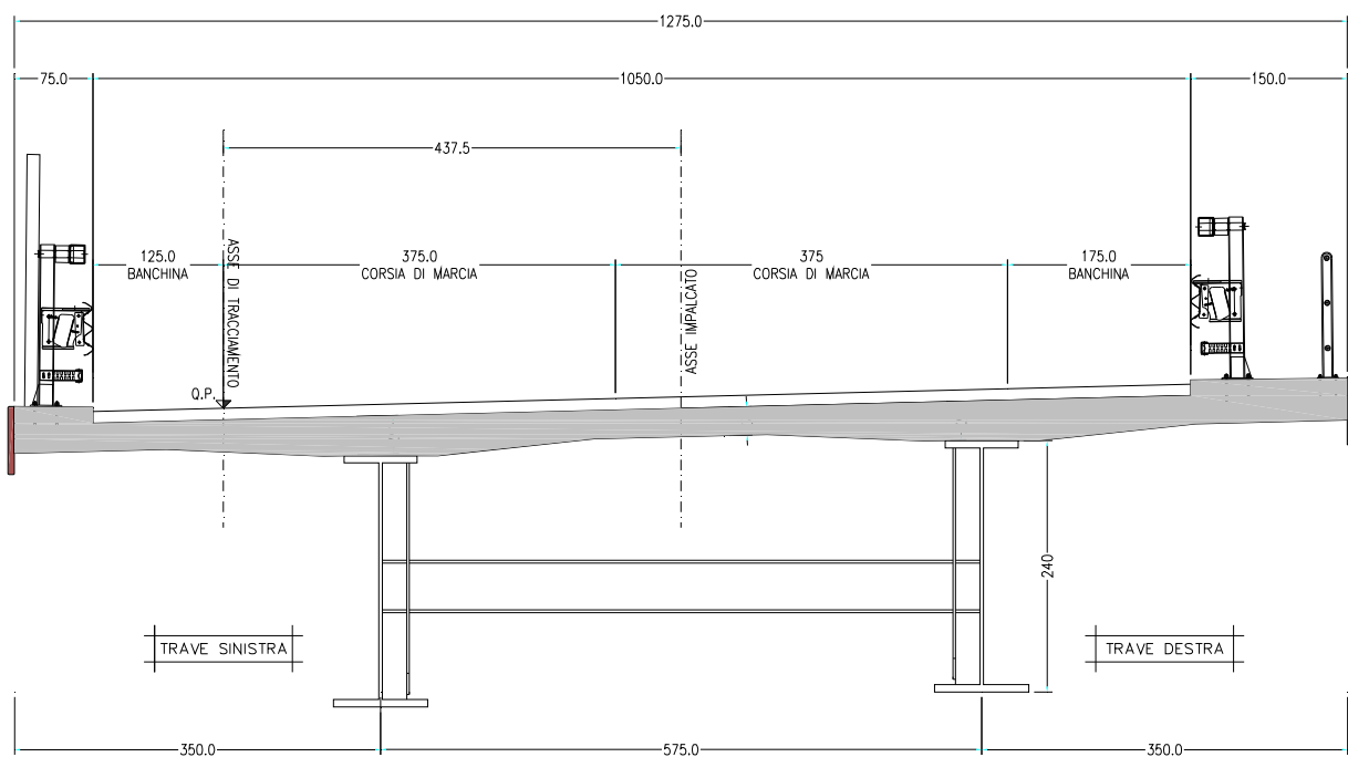
Figura 1.1 - Sezione trasversale impalcato
