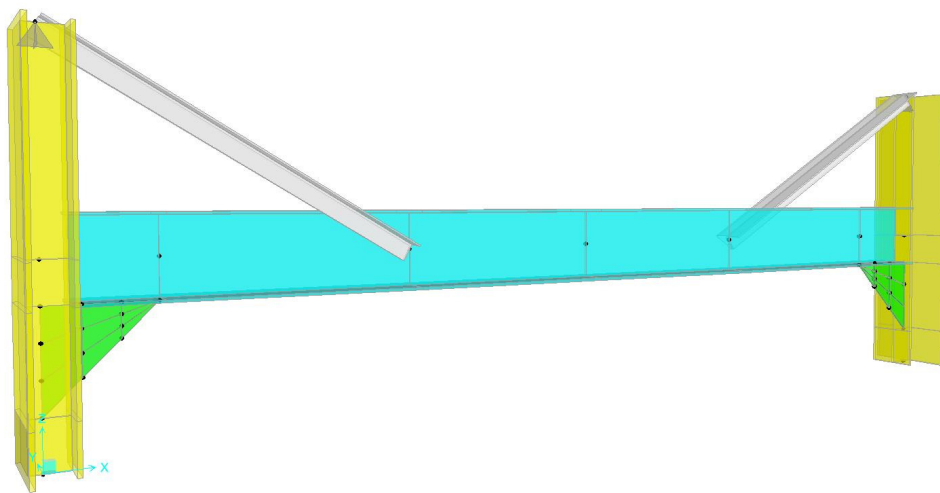
Figura 4.20 – Telaio trasversale corrente
