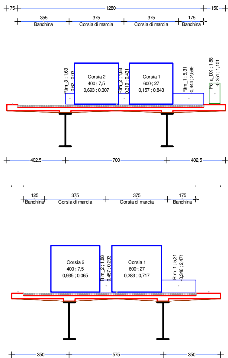
Figura 2.1 – Disposizione trasversale dei carichi mobili per il dimensionamento delle travi principali (SLE)
