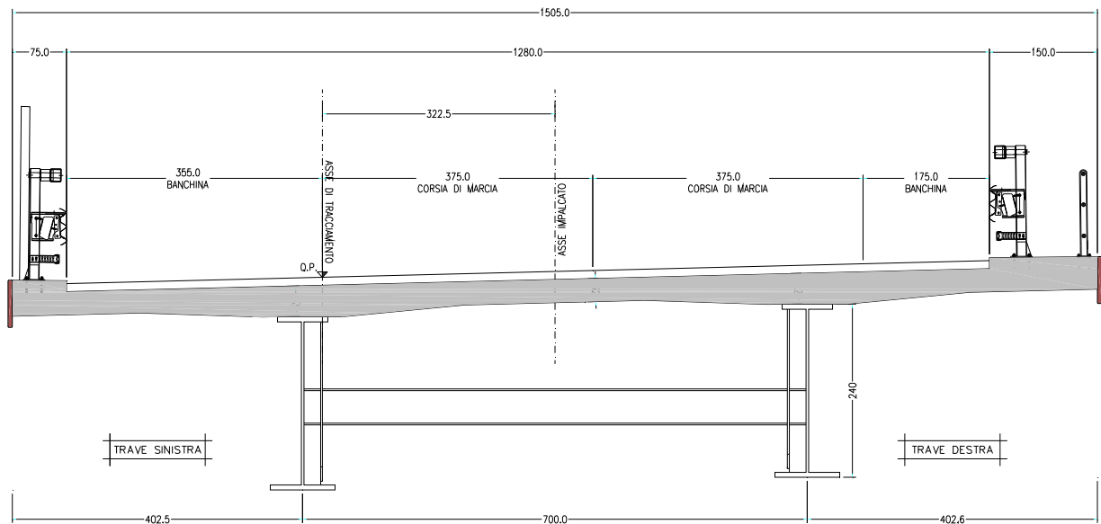
Figura 1.2 – Sezione trasversale impalcato
