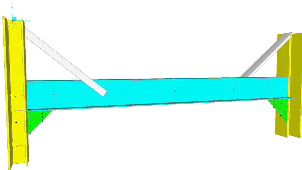
Figura 4.16 – Telaio trasversale corrente
