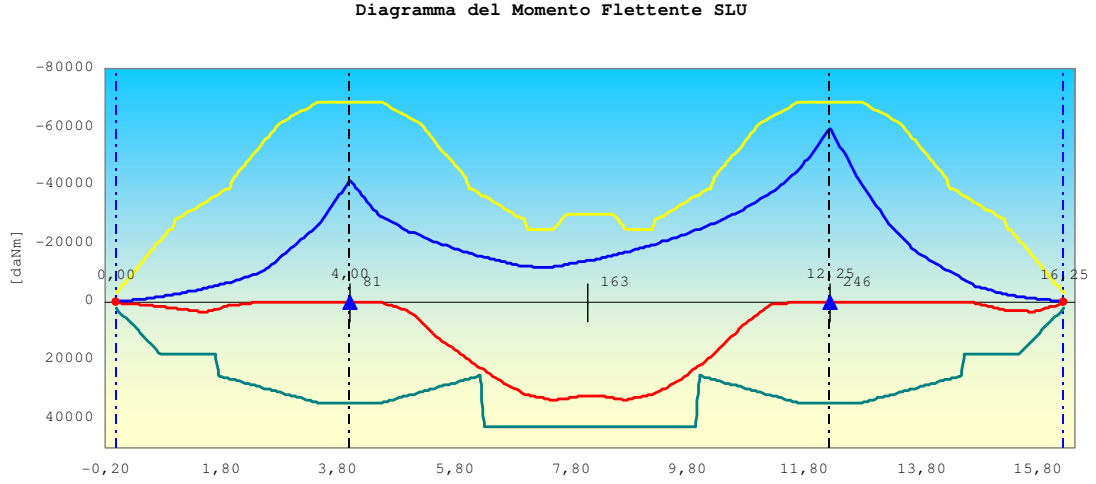
Figura 5.24 – Involuppo delle sollecitazioni flettenti (SLU) e diagrammi dei momenti resistenti delle armature
