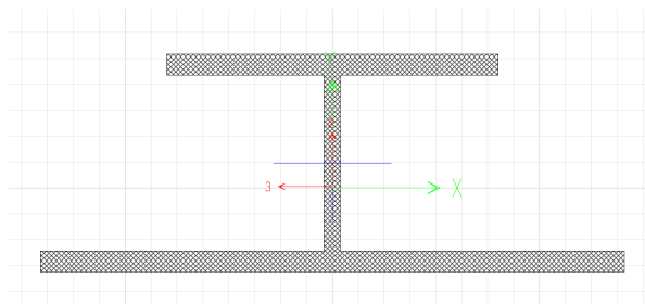
Figura 4.17 – Sezione del montante
