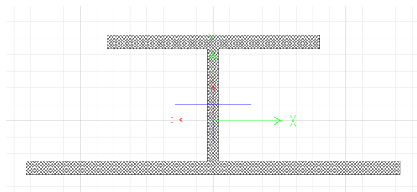
Figura 4.21 – Sezione del montante
