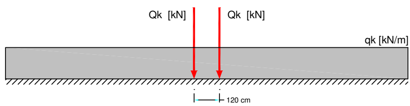
Figura 1.5 – Carico mobile agente sulla trave maggiormente sollecitata
