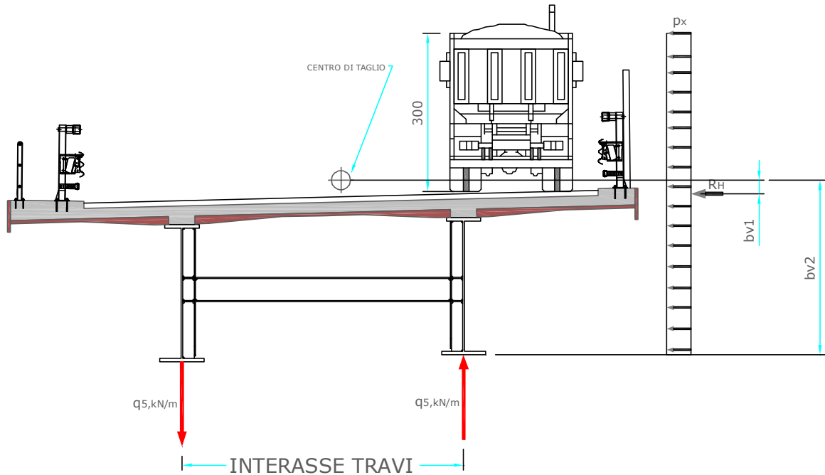
Figura 1.6 – Schema delle azioni indotte dal vento
