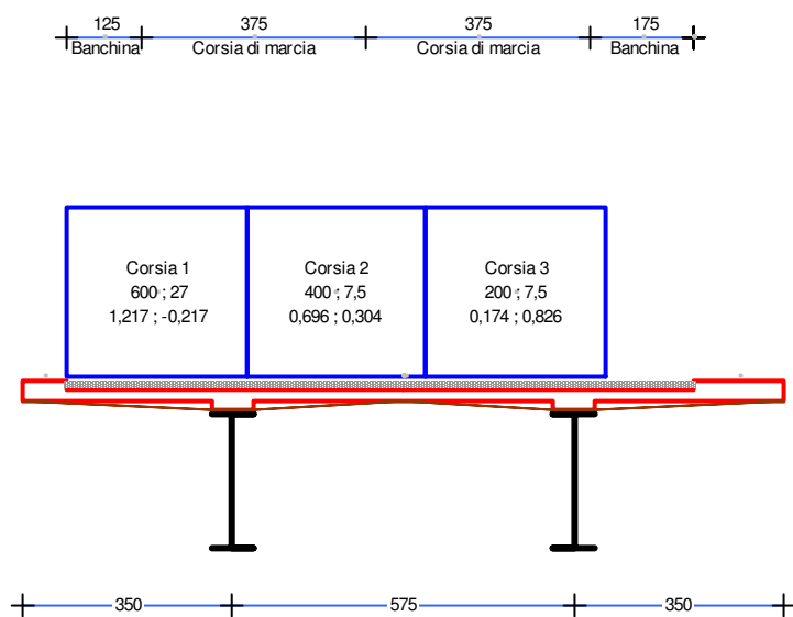
Figura 1.3 – Disposizione trasversale dei carichi mobili per il dimensionamento delle travi principali (SLU) per le zone dell’impalcato aventi larghezza della sezione trasversale pari a 12,75m
