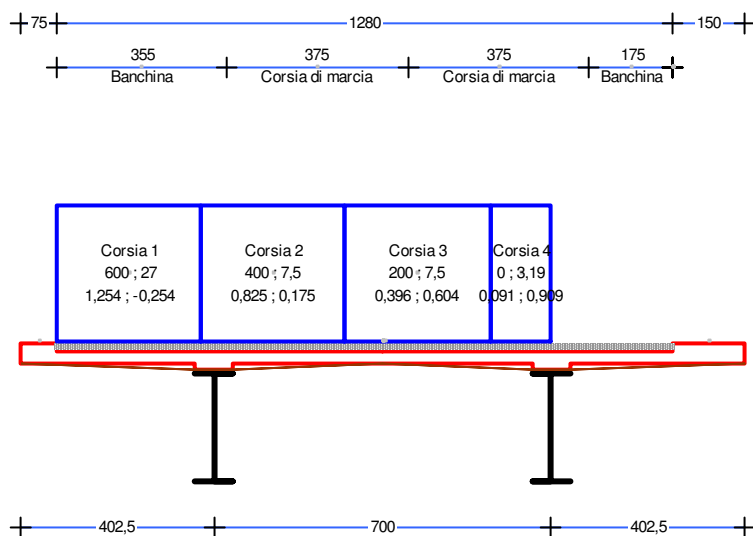
Figura 1.4 – Disposizione trasversale dei carichi mobili per il dimensionamento delle travi principali (SLU) per le zone dell’impalcato aventi larghezza della sezione trasversale pari a 15,05m
