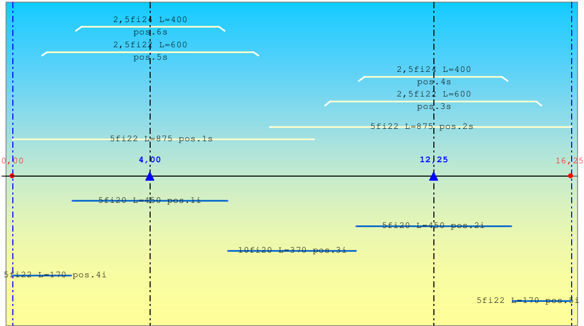
Figura 5.22 - Disposizione delle armature trasversali della soletta
