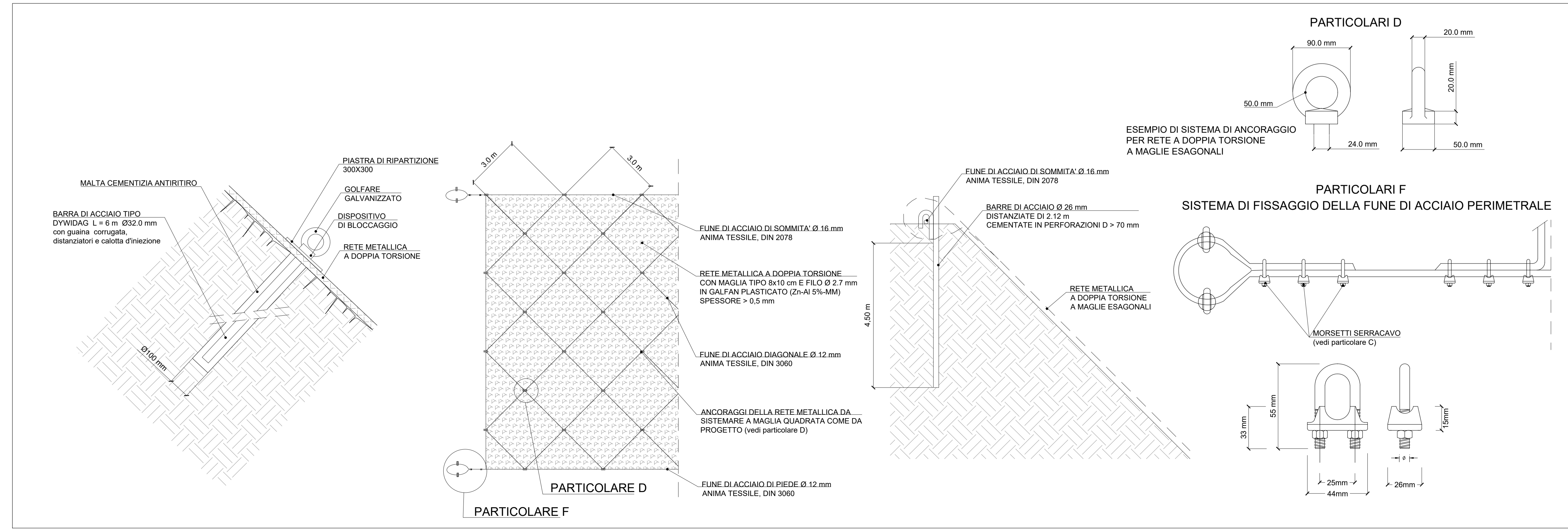
OPERE DI PROTEZIONE SCARPATA
