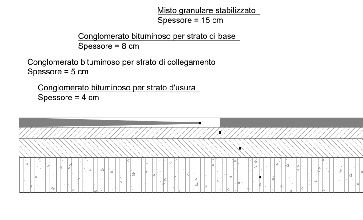
DETTAGLIO PACCHETTO PAVIMENTAZIONE Scala 1:10
