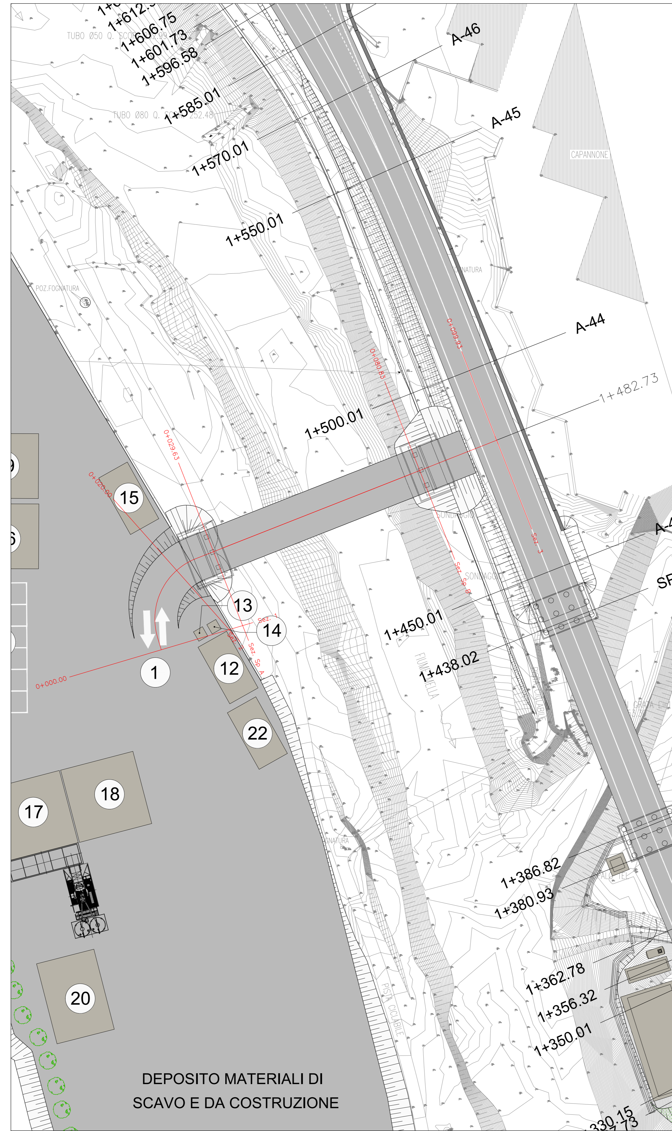
PLANIMETRIA DI PROGETTO Scala 1:500
