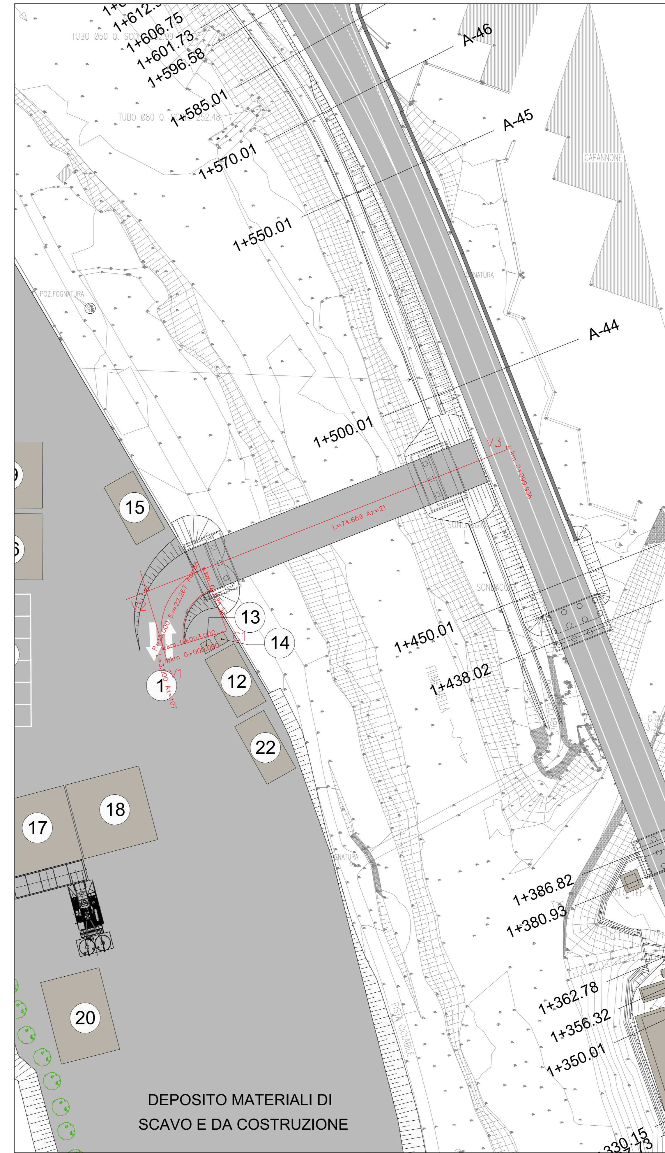
PLANIMETRIA DI TRACCIAMENTO Scala 1:500
