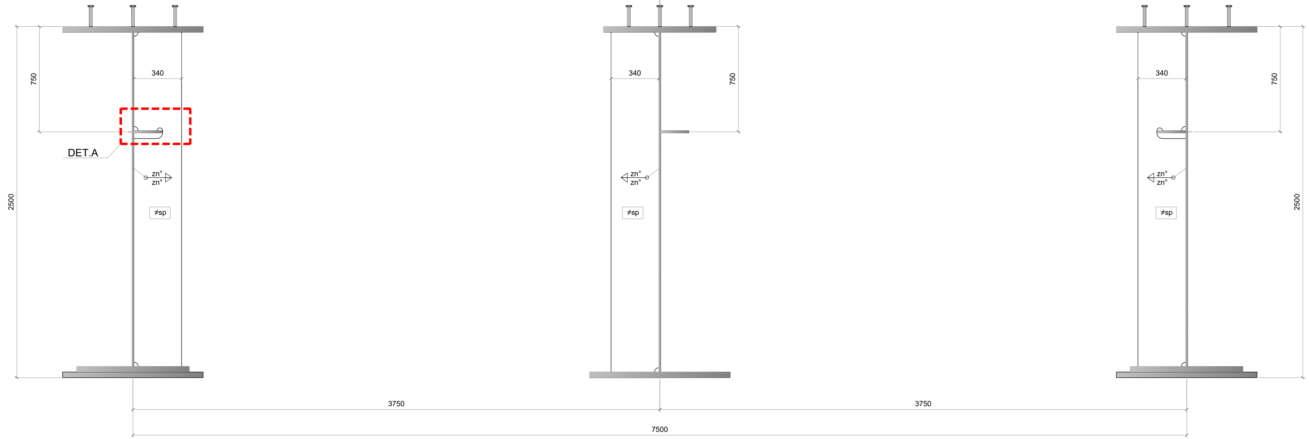
IRRIGIDENTE INTERMEDIO TIPICO I1-I2 - scala 1:15
