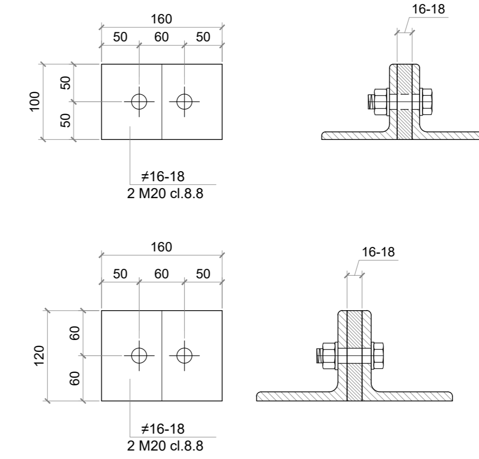
DETTAGLIO CALASTRELLI - scala 1:5
