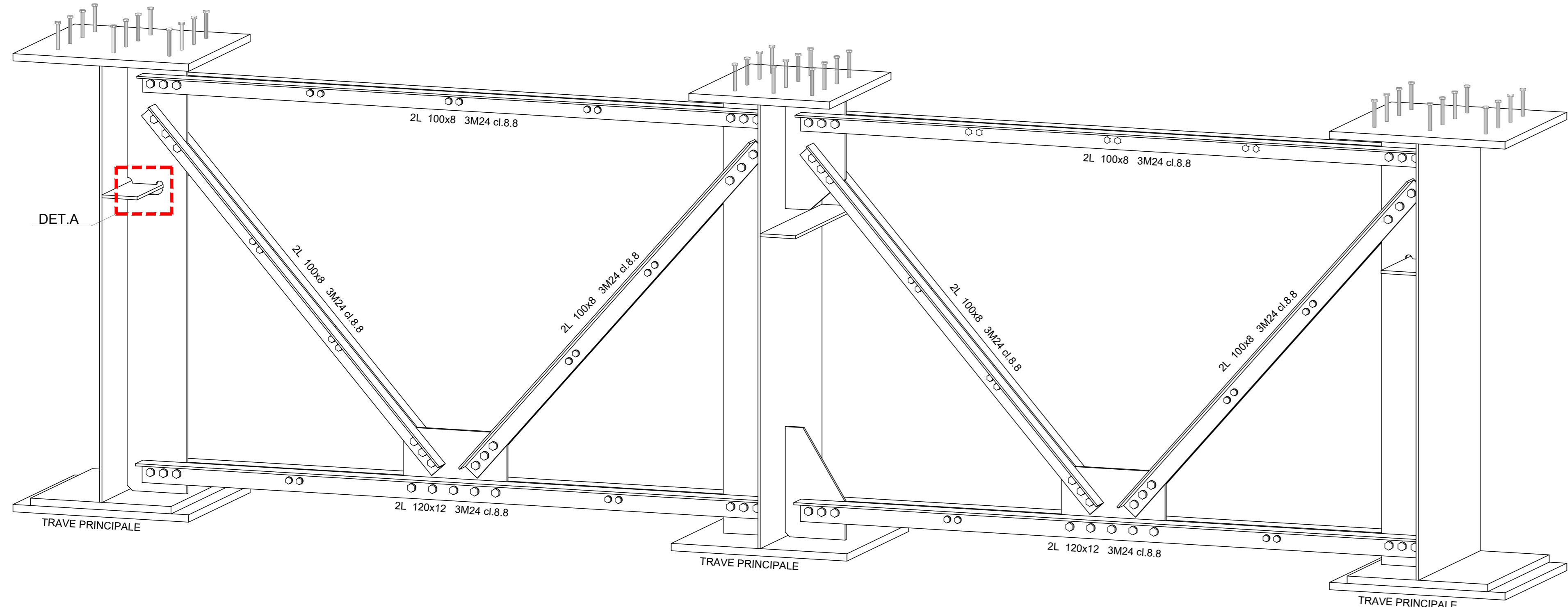
Vista assometrica diaframma intermedio - scala 1:15
