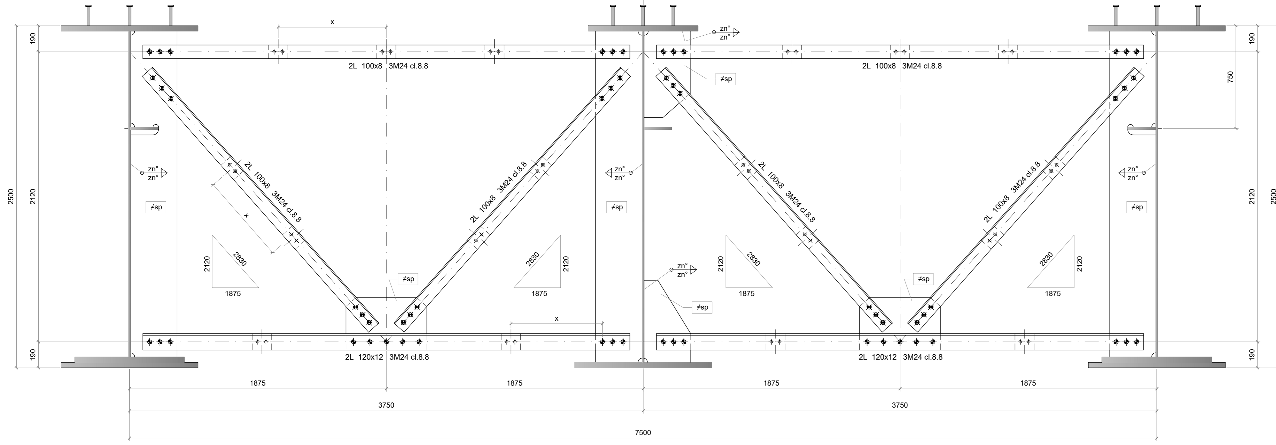
DIAFRAMMA INTERMEDIO TIPICO Di - scala 1:15
