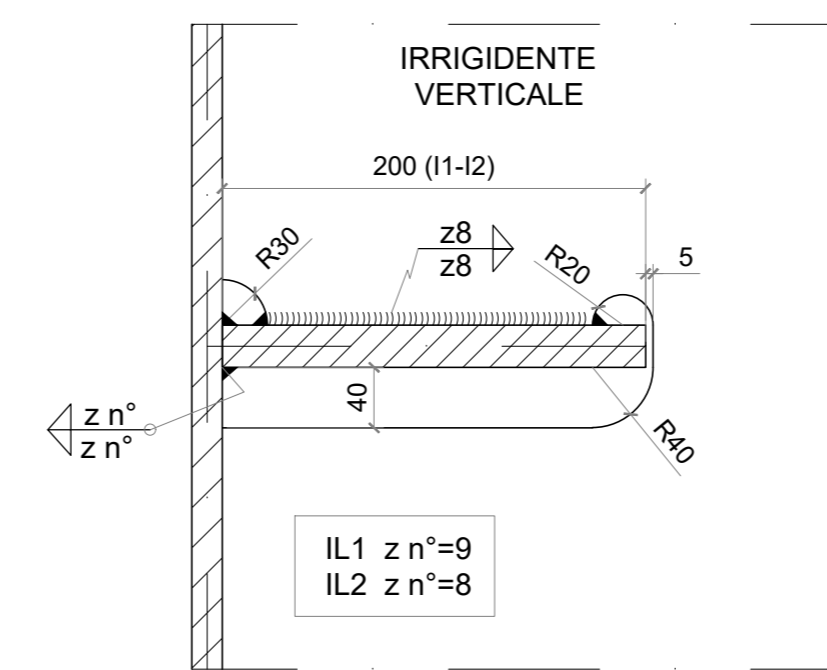
DETTAGLIO A - scala 1:5-
