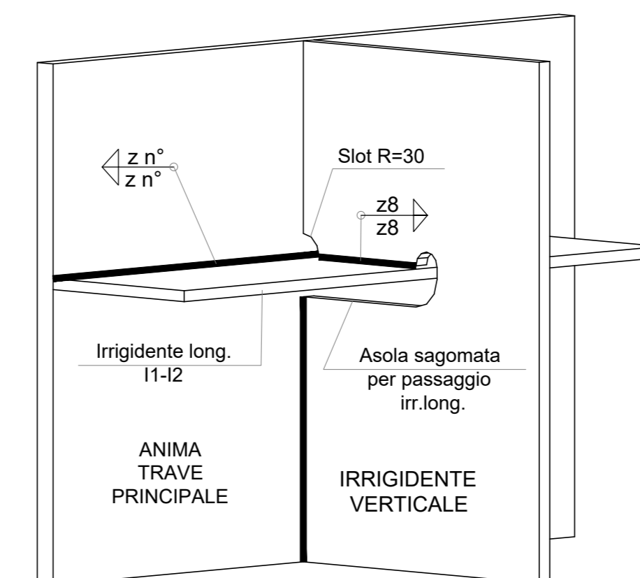
Vista assometrica
