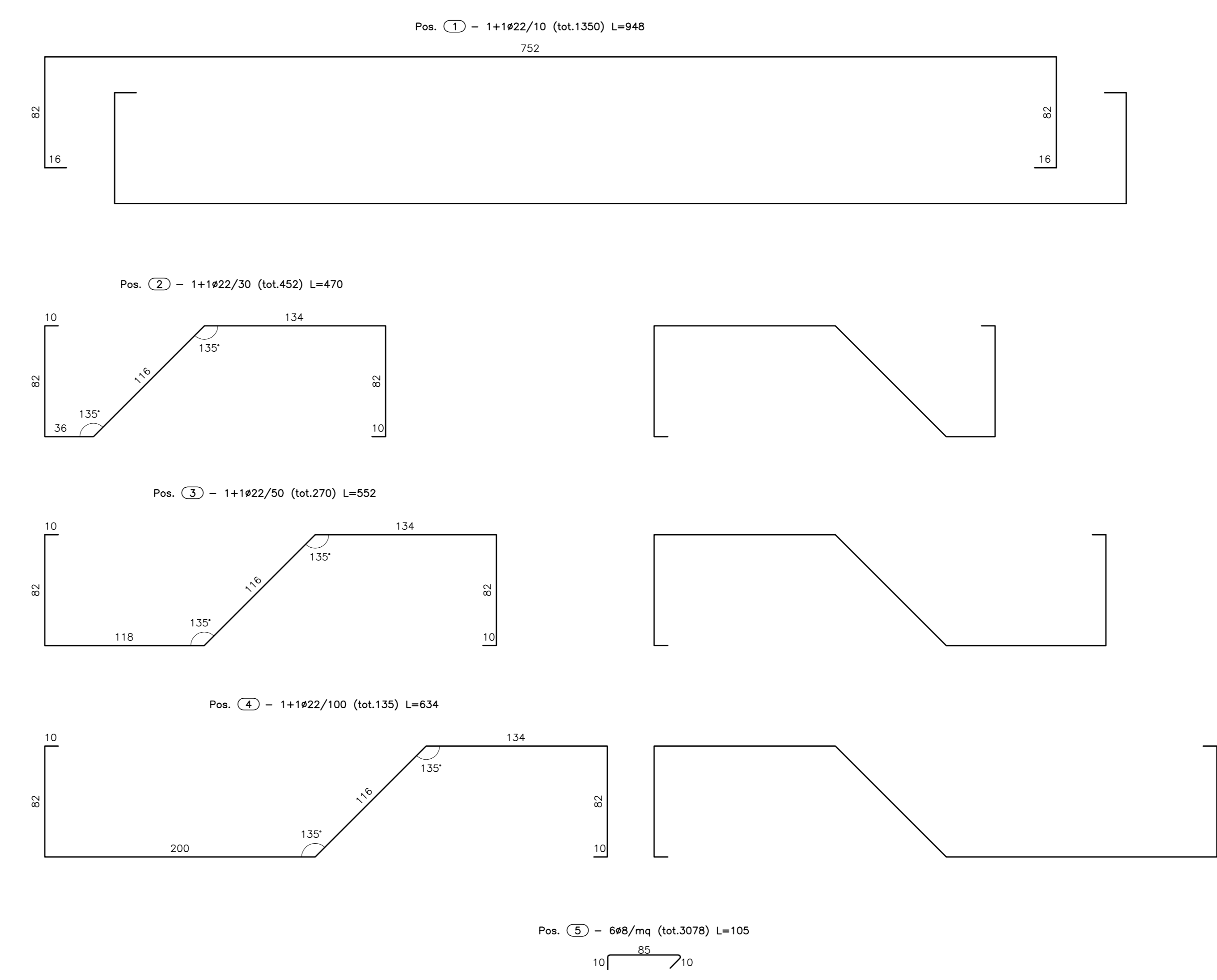
ARMATURA FONDAZIONE
