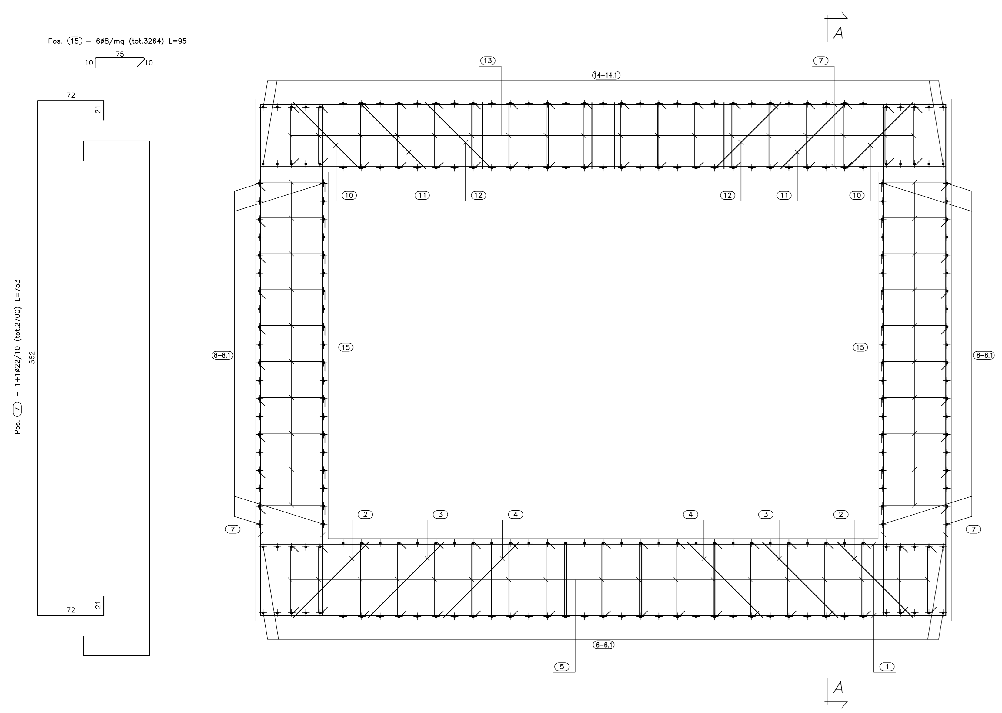
SEZ. B-B (SCALA 1:25)
