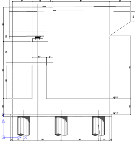
CARPENTERIA SPALLA "SpB" SEZIONE A-A SCALE 1:60
