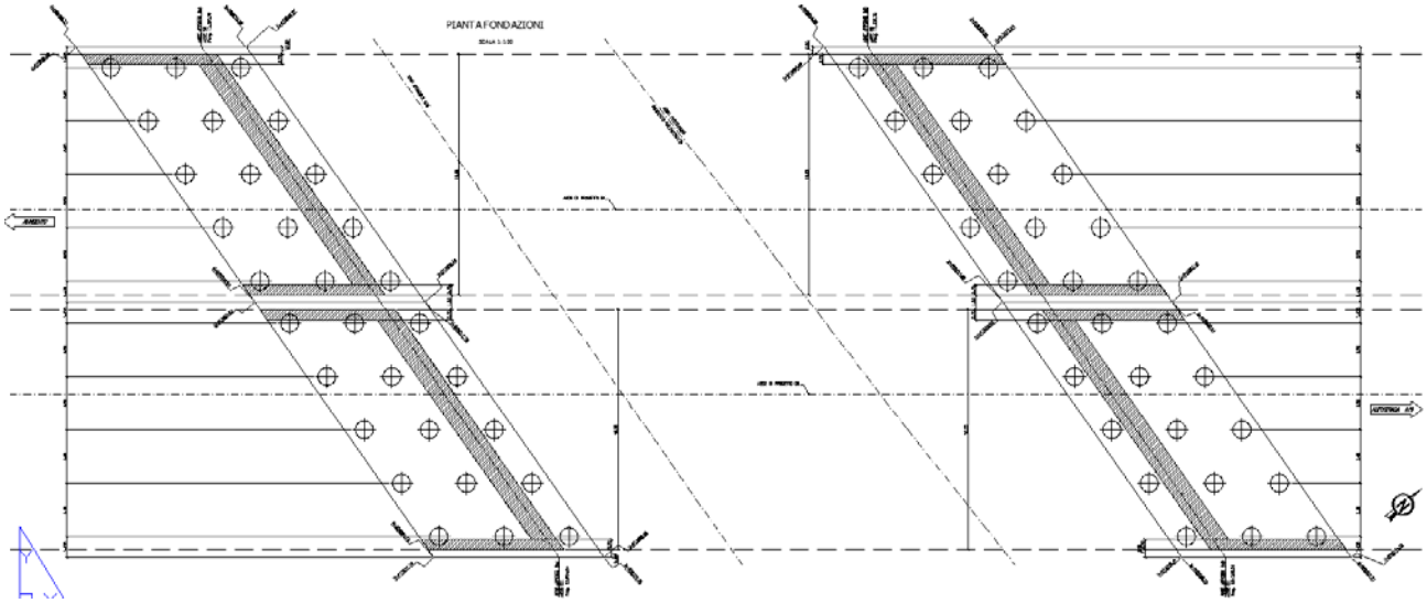
CARPENTERIA SPALLA "SpA" SEZIONE A-A SCALE 1:60
