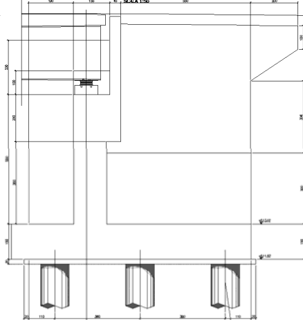
CARPENTERIA SPALLA "SpB" VISTA LATERALE SCALE 1:60
