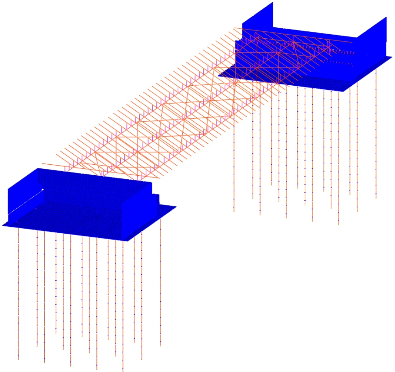
Modello 3d della struttura agli elementi finiti
