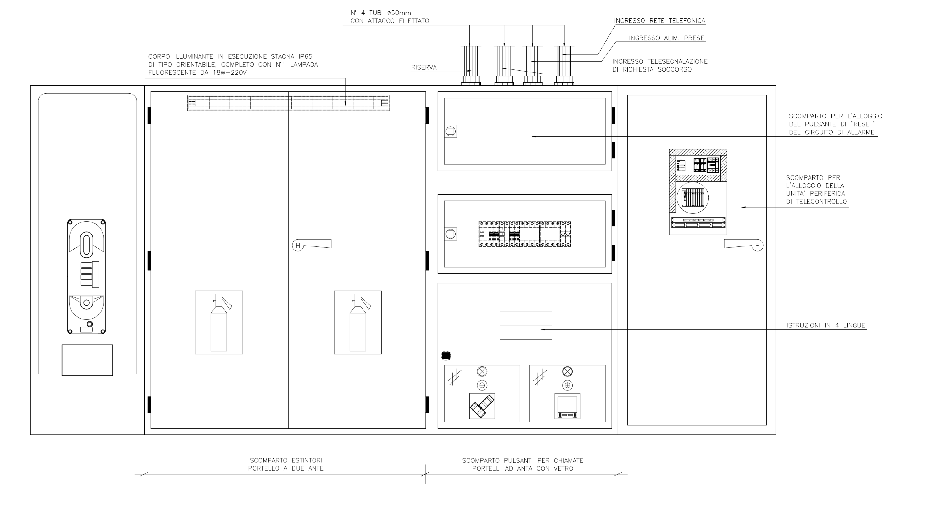
CASSETTA DI SEGNALAZIONE SOCCORSO IN GALLERIA
