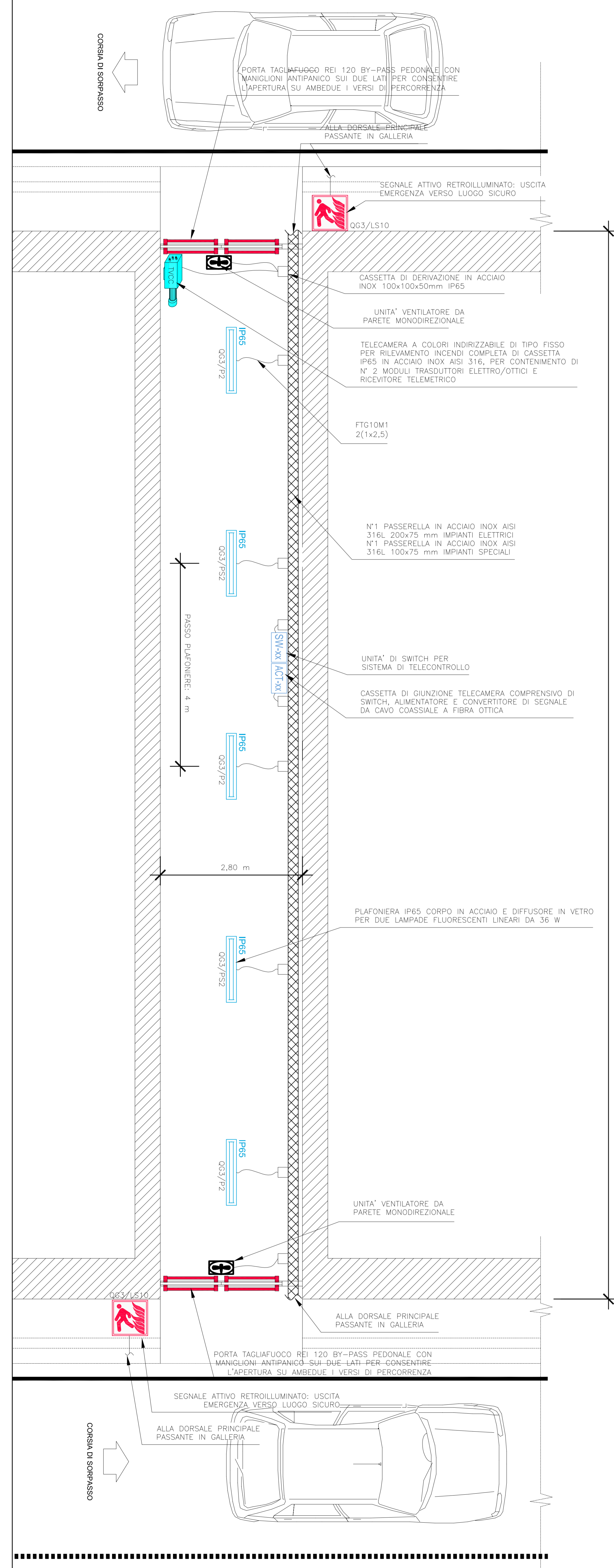
TIPICO ATTREZZAGGIO BY-PASS PEDONALE (SCALA 1:100)
