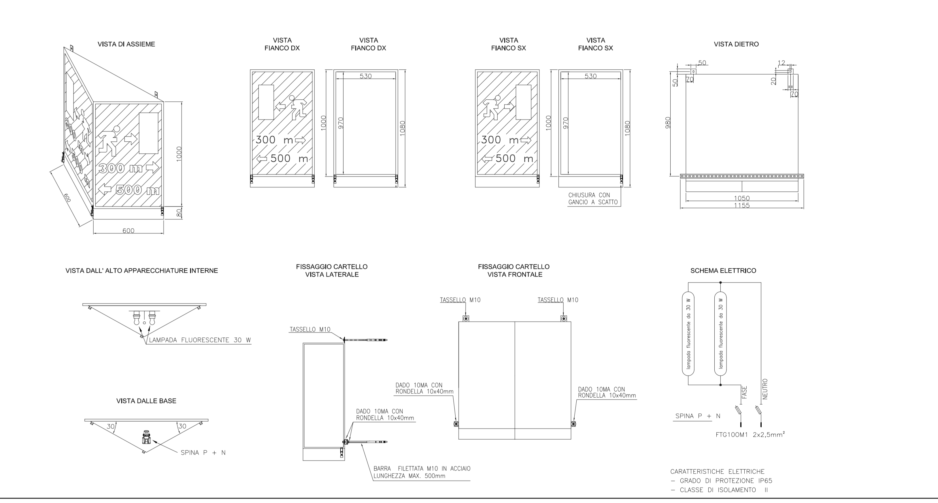
PARTICOLARE SEGNALE "DISTANZA DA LUOGO SICURO"
