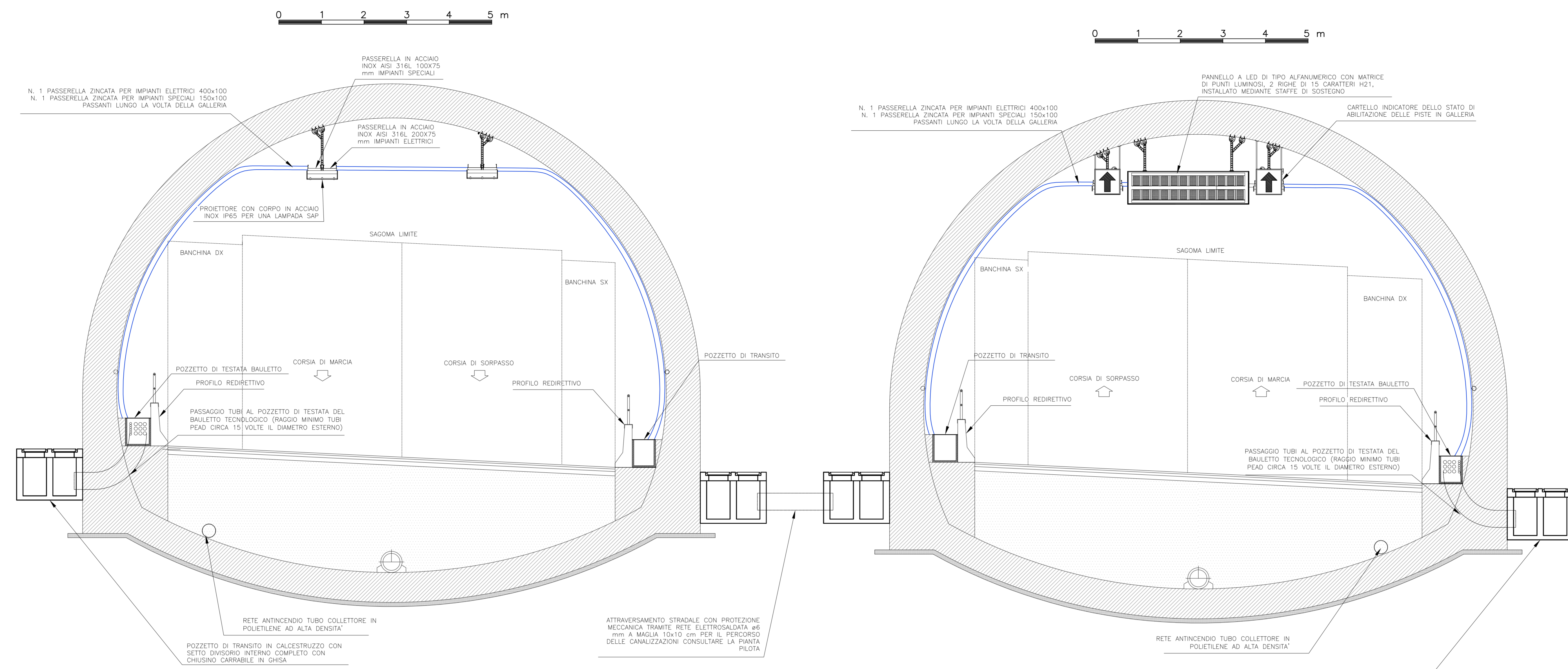
SEZIONE IN CORRISPONDENZA DELL'IMBOCCO LATO AGRIGENTO (SCALA 1:100)
