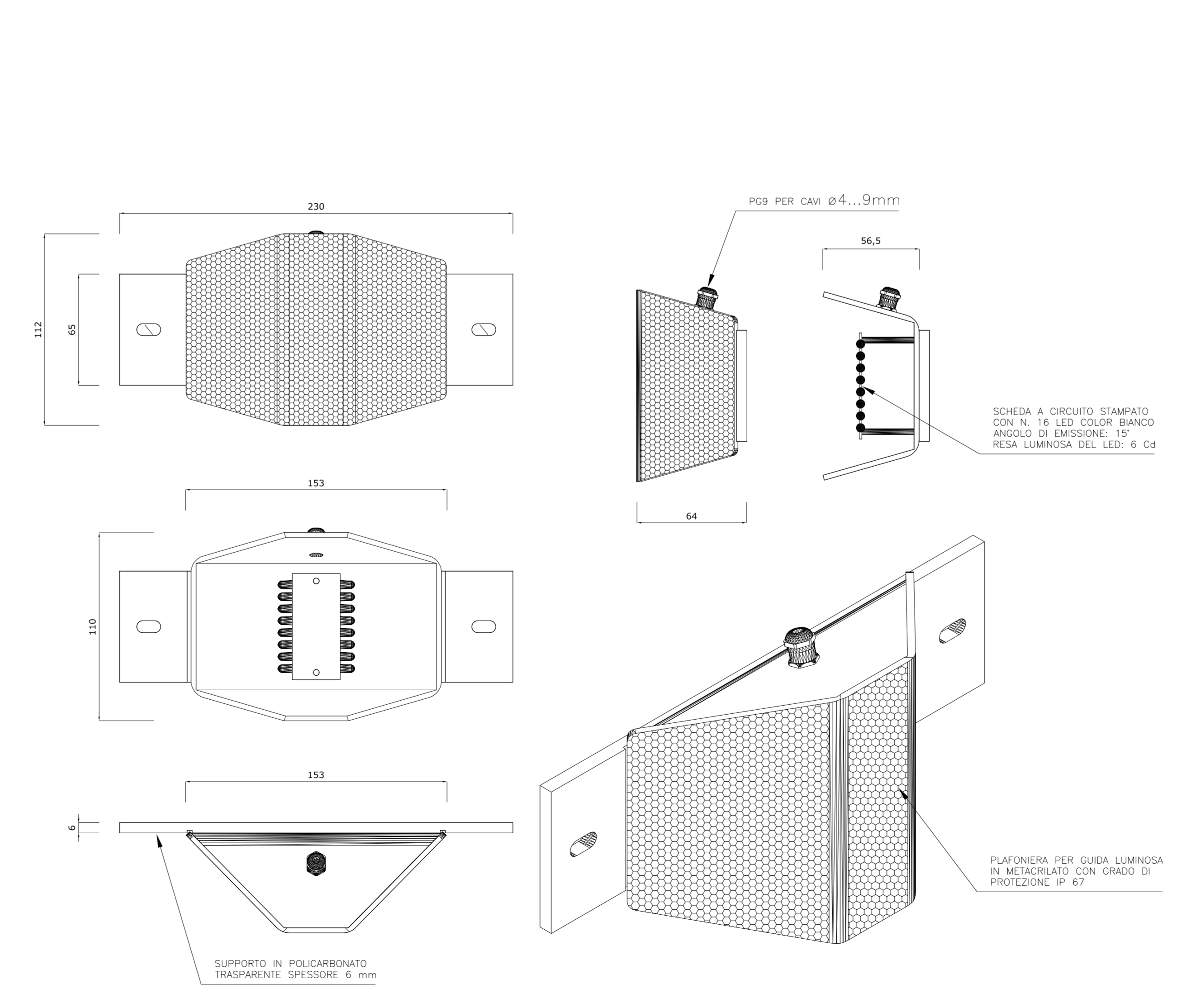
CORPO ILLUMINANTE A LED SU BARRIERA REDIRETTIVA PER ILLUMINAZIONE DI SICUREZZA (INDICAZIONE VERSO DI PERCORRENZA, ILLUMINAZIONE DEL CAMMINAMENTO)
