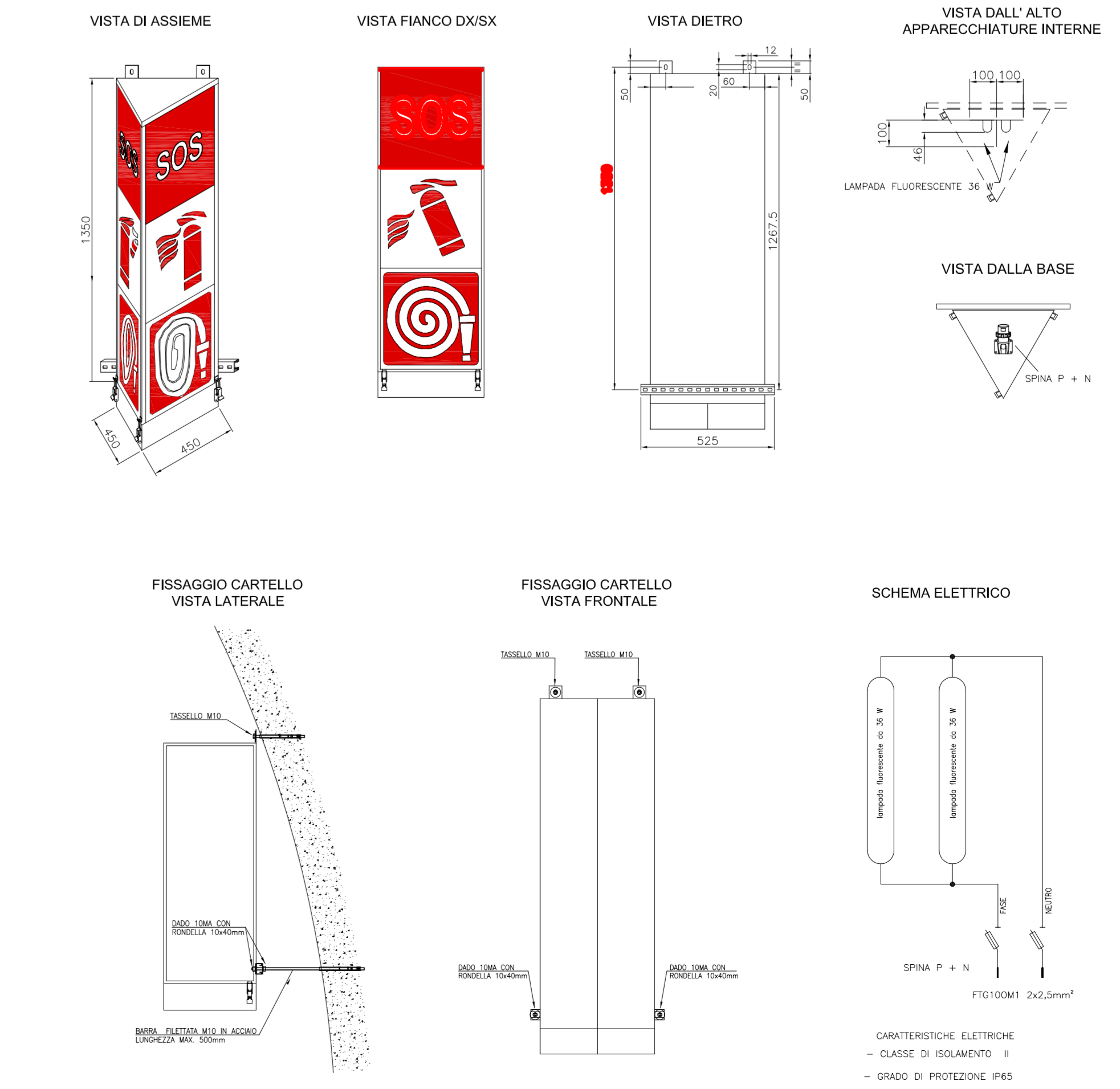
PARTICOLARE SEGNALE ARMADIO SOS CON ESTINTORE BIFACCIALE
