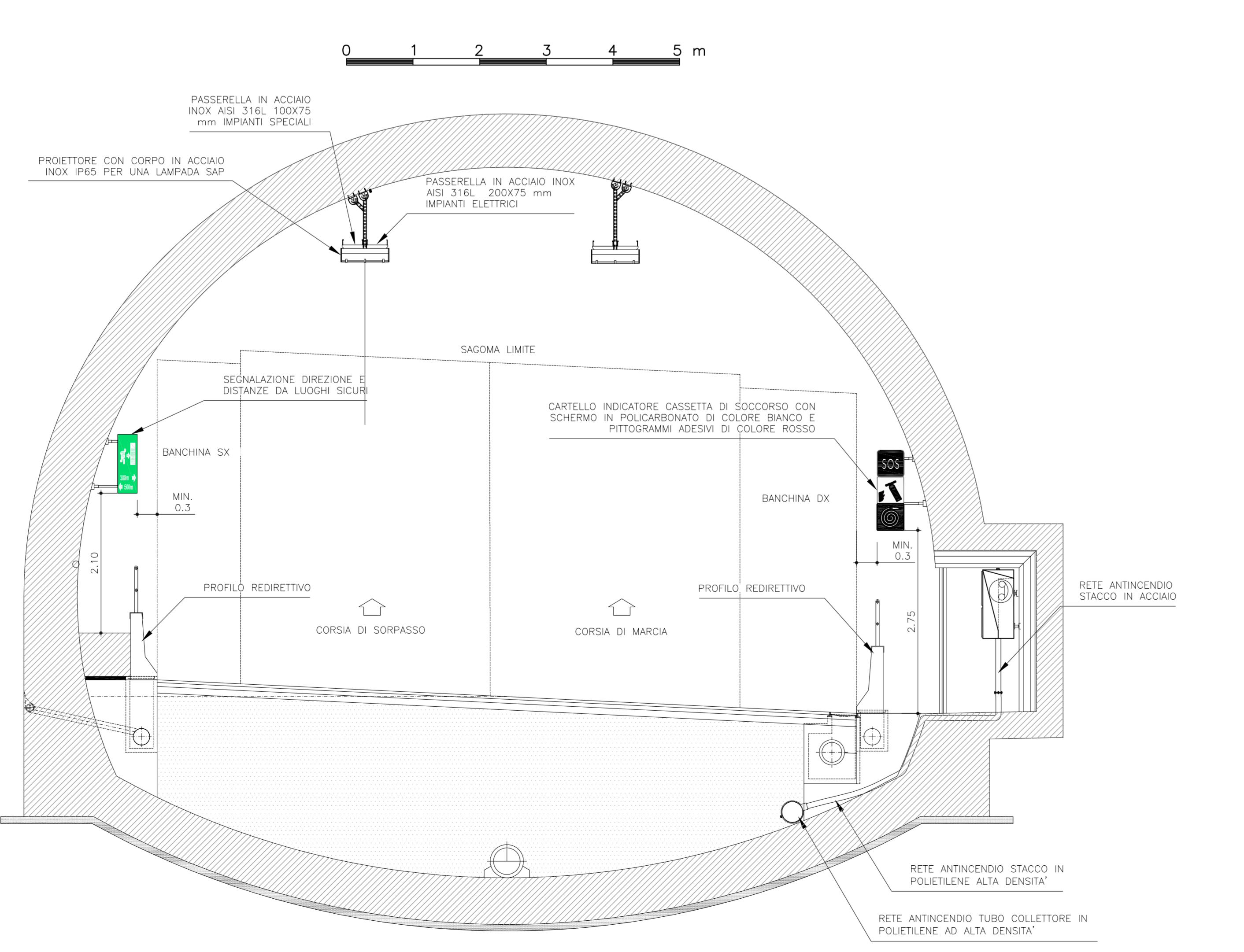
SEZIONE IN CORRISPONDENZA DELLA CASSETTA SOS E DEL CARTELLO COMPOSITO DI SEGNALAZIONE PERICOLO (SCALA 1:100)
