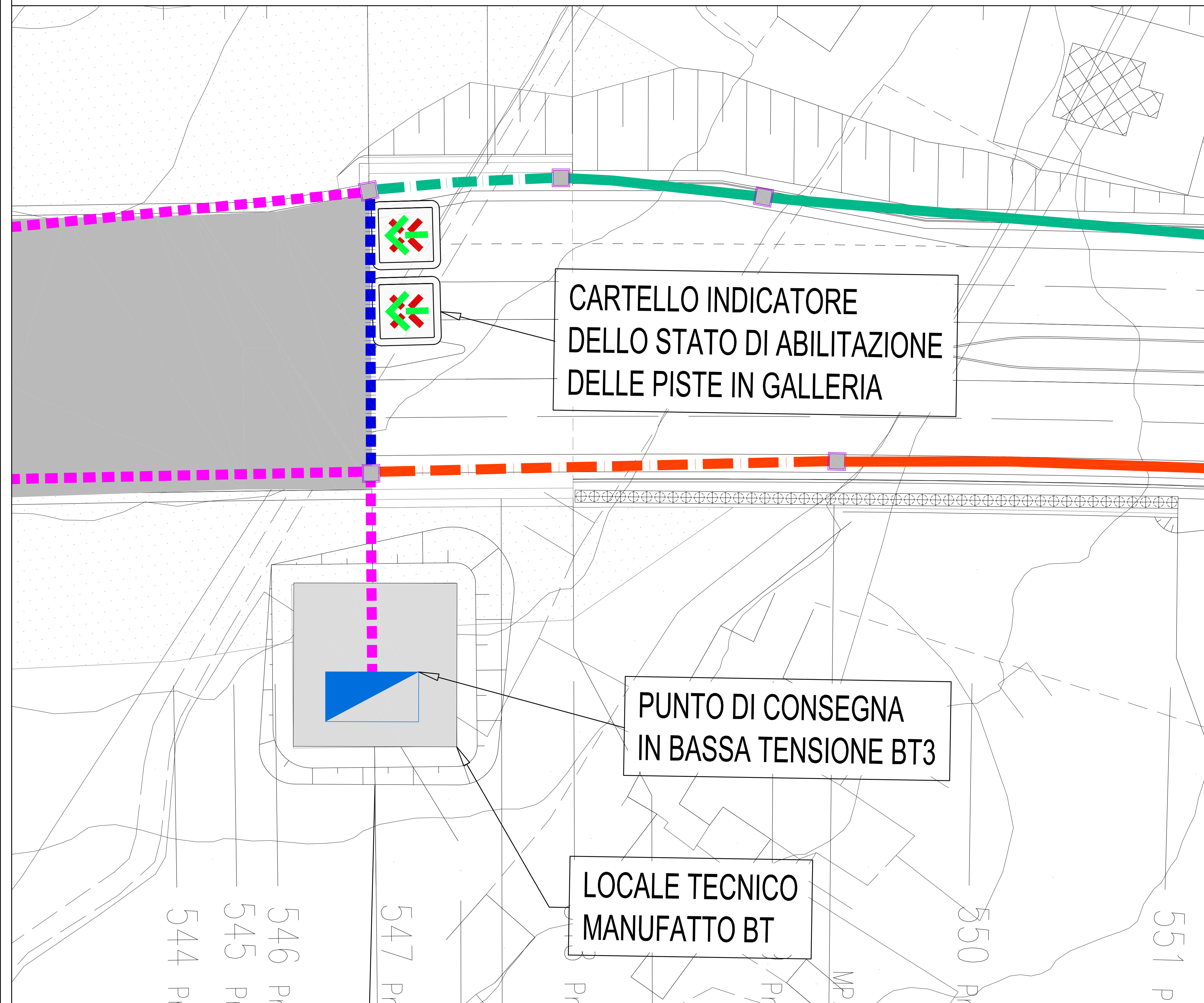
UBICAZIONE LOCALE TECNICO PER PUNTO DI ALIMENTAZIONE IN BASSA TENSIONE - SCALA 1:200
