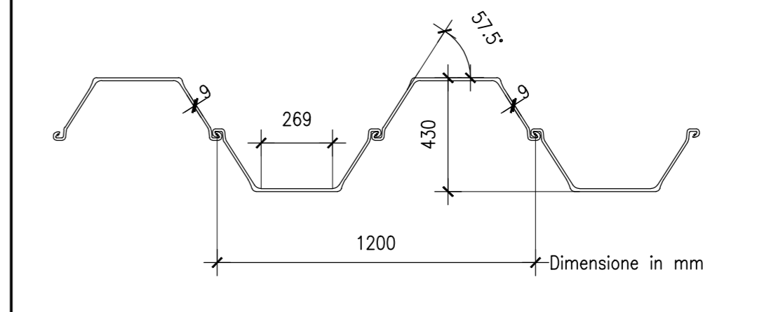
SEZIONE PALANCOLA PROVVISORIA TIPO "PU18" SCALA 1:5
