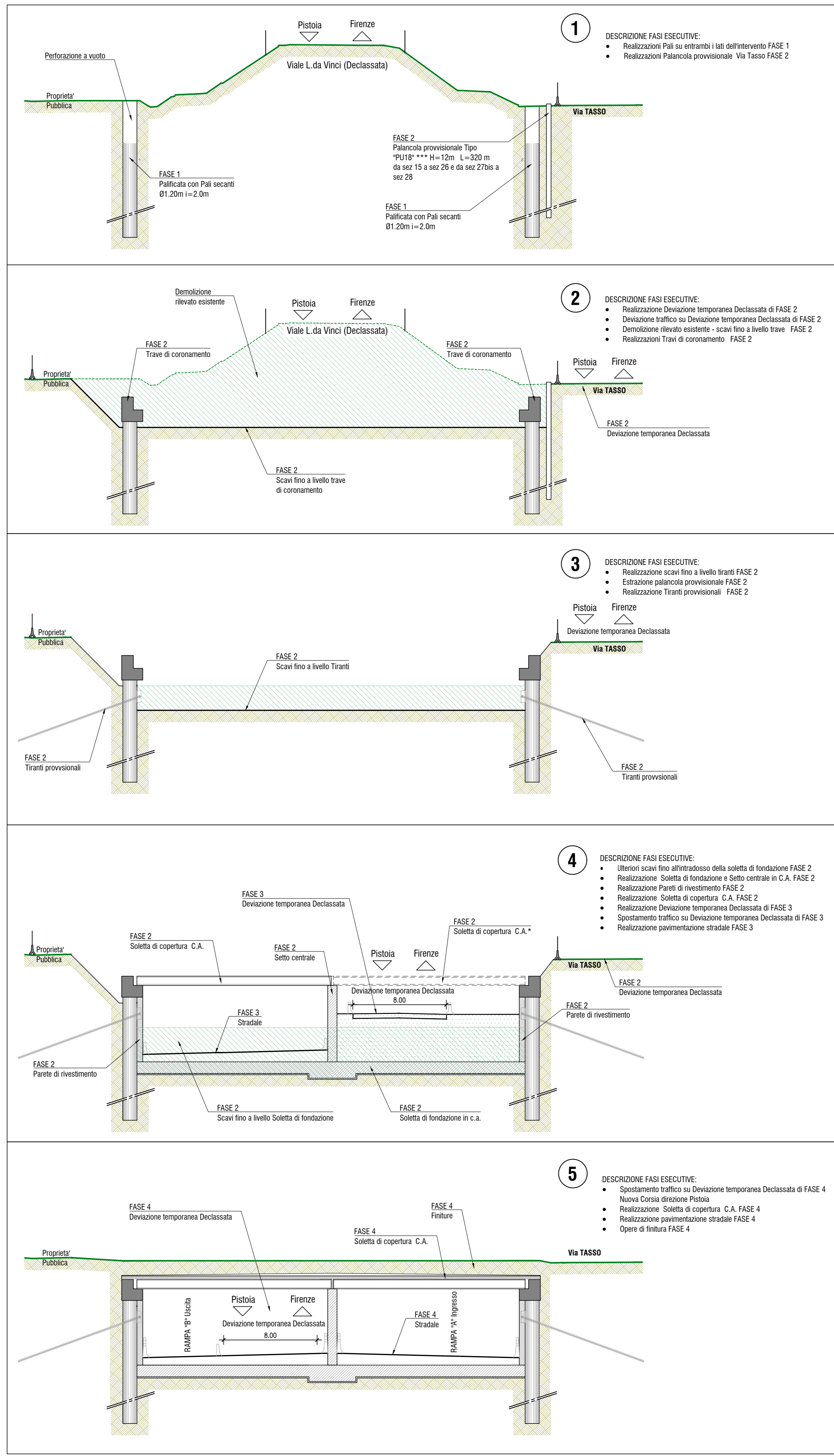
FASI ESECUTIVE SEZIONE TIPO TRATTO "C" scala 1:200
