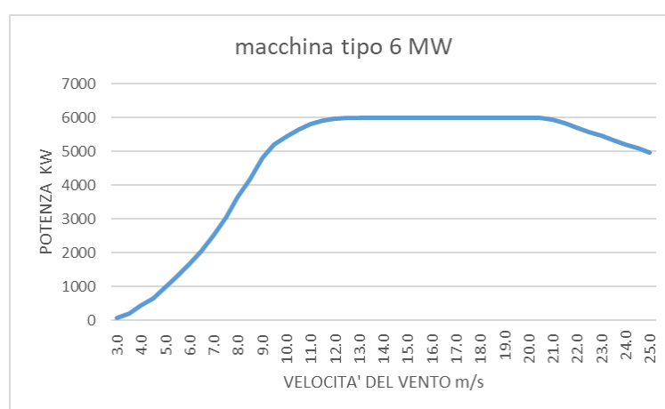
Caratteristiche Aerogeneratore tipo
