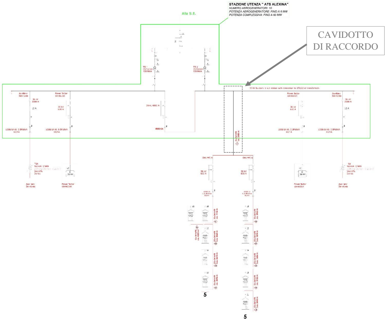
Schema elettrico unifilare (da tav.- Schema elettrico unifilare)
