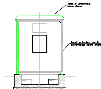
SEZIONE W-W
