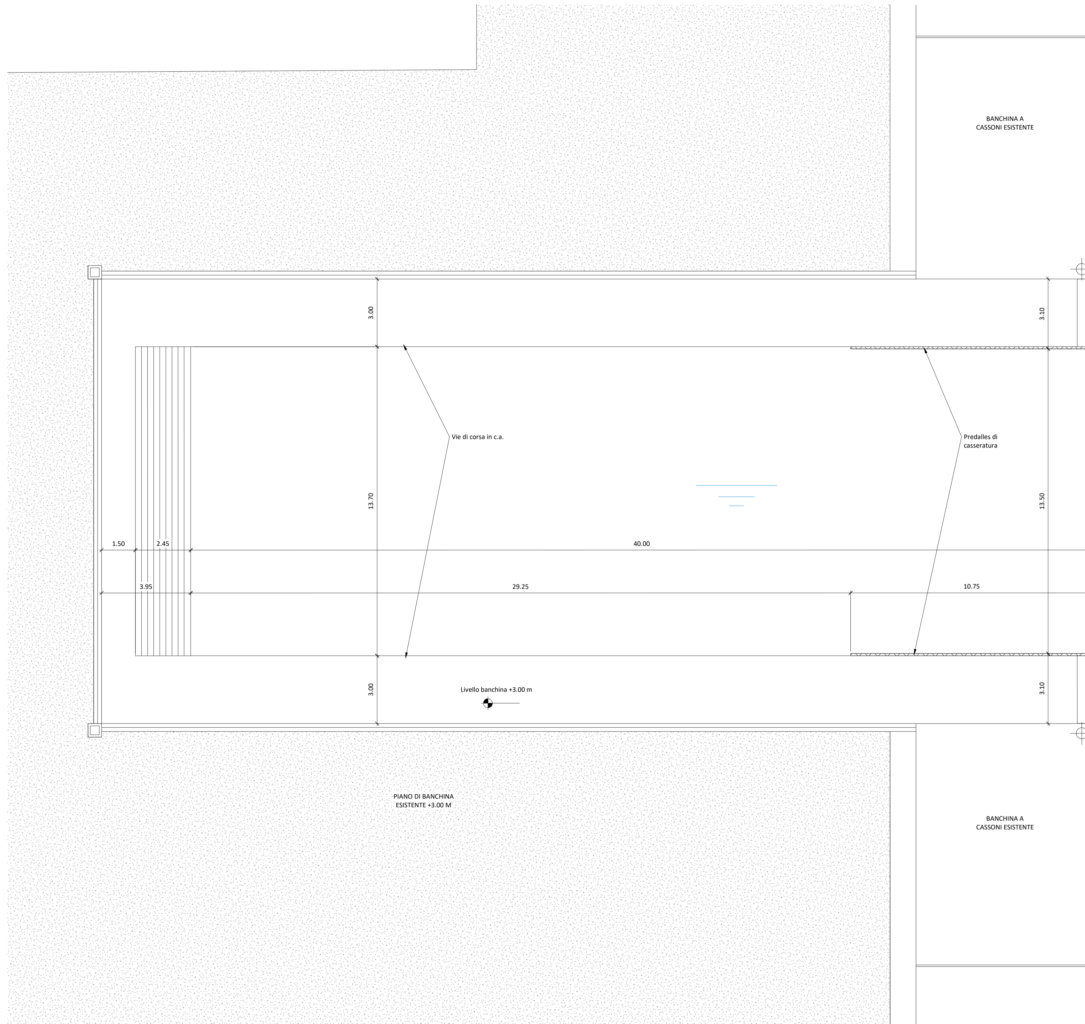
1 - Pianta quota banchina +3.00 m 1 : 100
