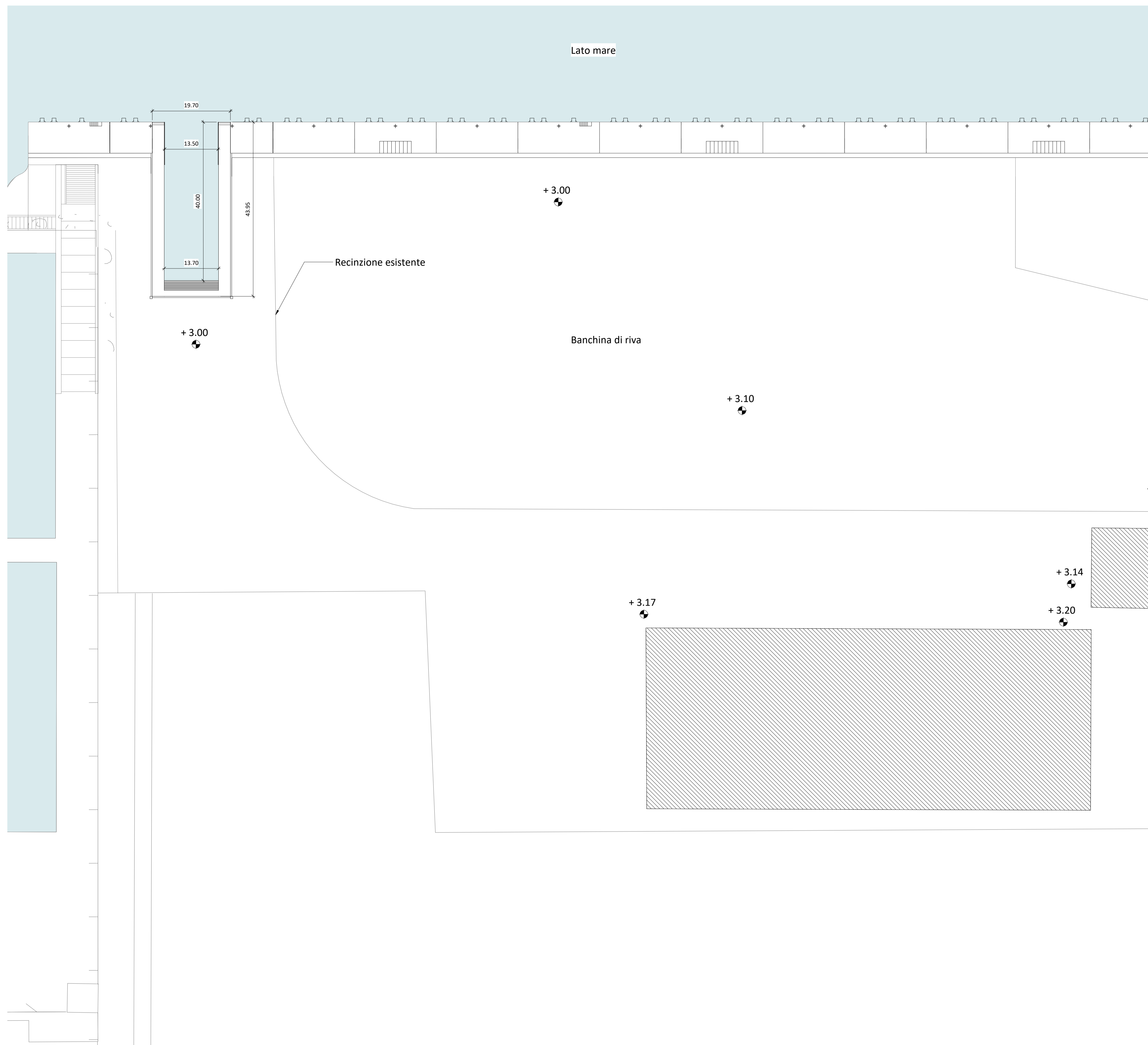
1 - Planimetria generale 1 : 500
