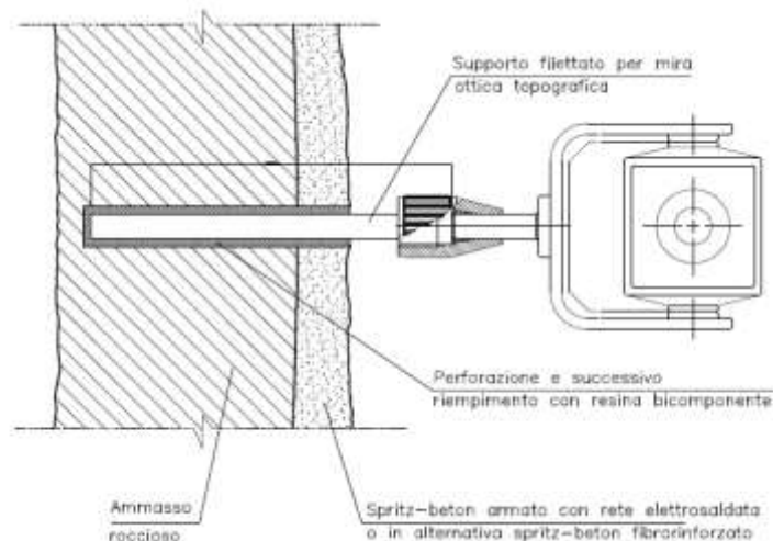
Figura 9-1. Particolare mira topografica per misure di convergenza del prerinvestimento
