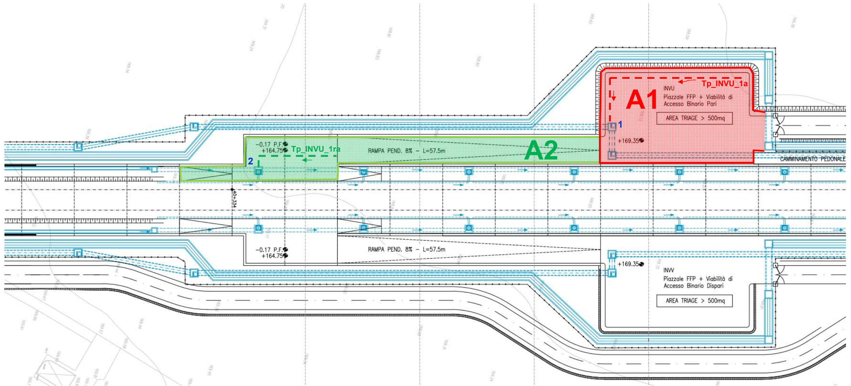
Figura 1 – Aree di captazione delle acque meteoriche
