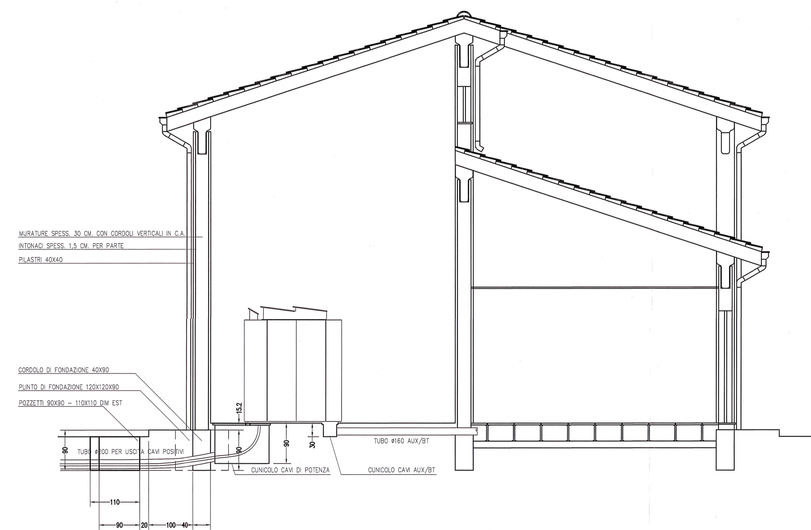
SEZIONE 1-1
