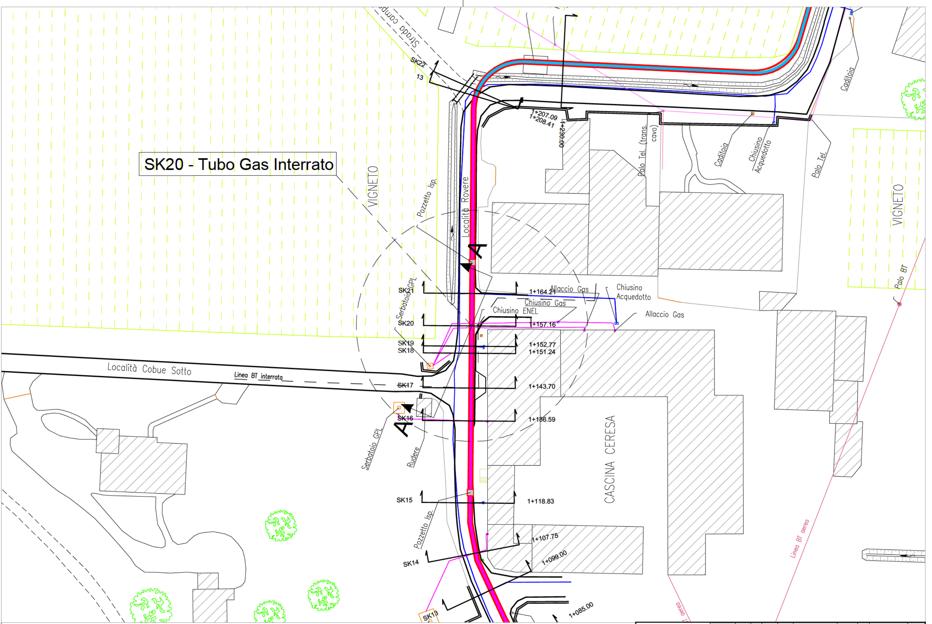
Stralcio planimetrico
