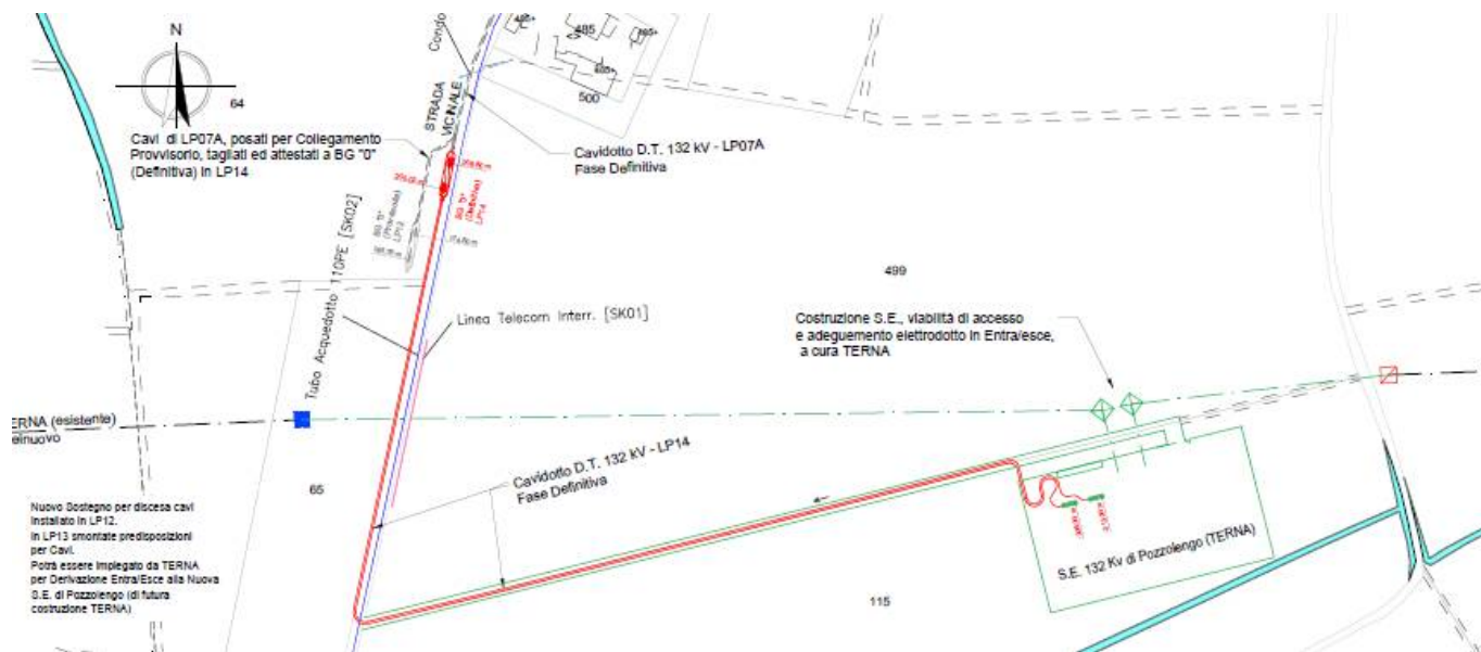
Inquadramento Territoriale del Tracciato del Cavidotto
