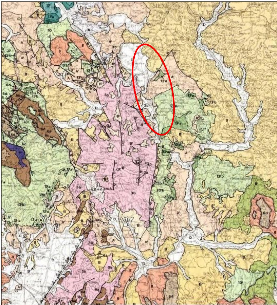
Figura 4-1 - Stralci della Carta Strutturale dell'Appennino settentrionale (tratta da CNR).
