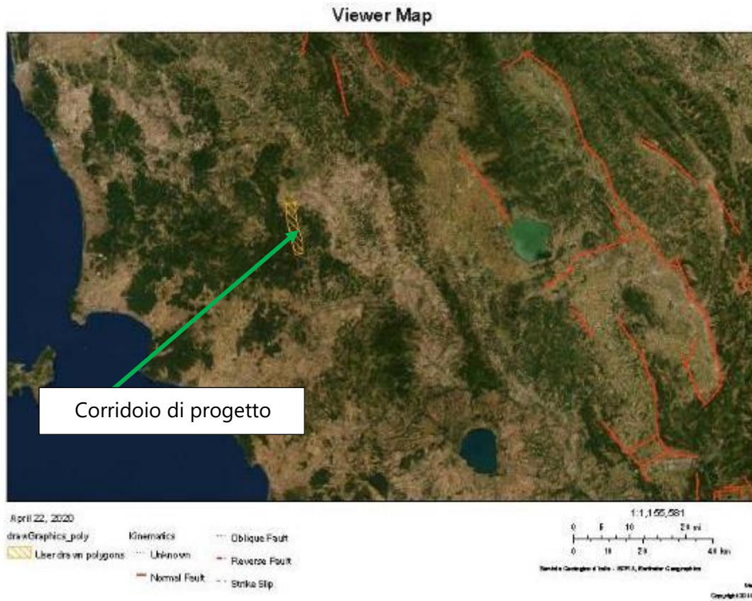
Figura 6-4 - Stralcio Carta delle faglie Capaci – Progetto ITHACA (ISPRA).
