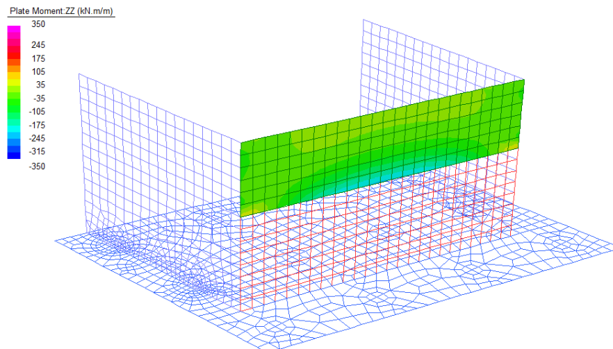
Figura 27: Momento Flettente verticale - Involuppo SLE
