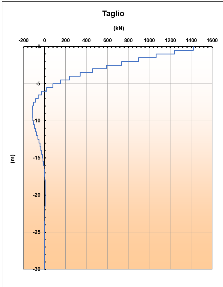
Figura 40 Diagramma del Taglio
