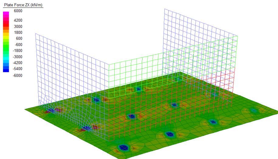
Figura 36: Sollecitazioni Taglianti V_{xz} - Involuppo SLU/SLV
