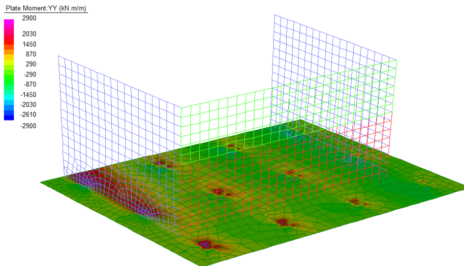
Figura 34: Momento Flettente trasversale - Inviluppo SLU/SLV
