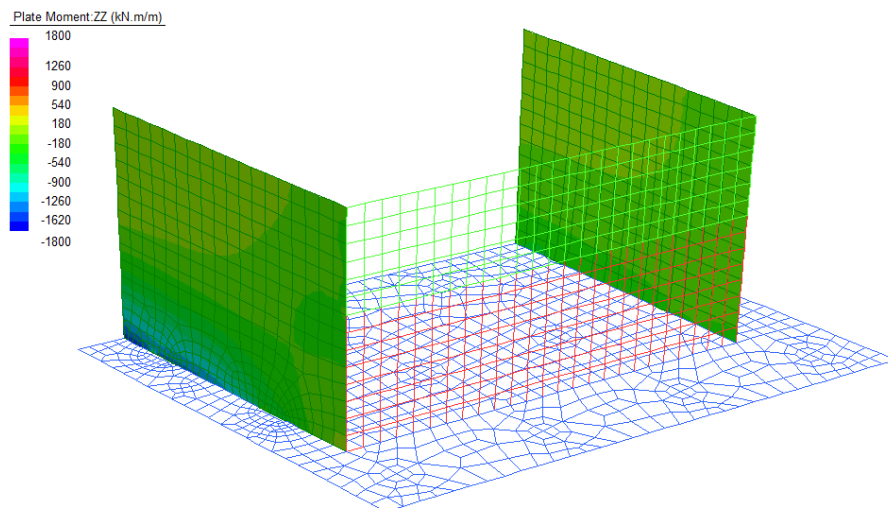
Figura 22: Momento Flettente verticale - Involuppo SLU/SLV
