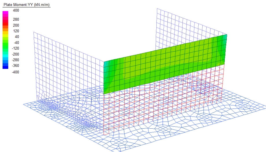
Figura 31: Momento Flettente orizzontale - Inviluppo SLE
