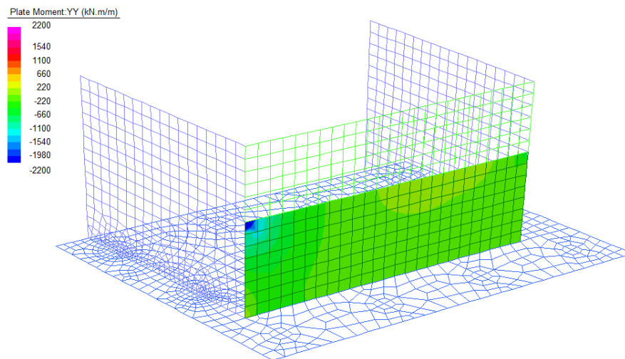
Figura 19: Momento Flettente orizzontale - Inviluppo SLE
