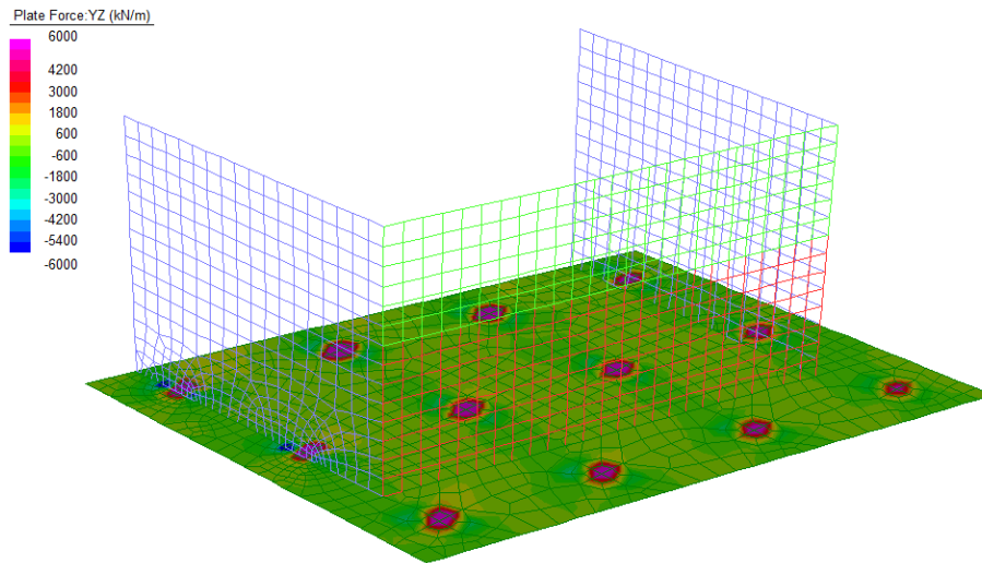
Figura 35: Sollecitazioni Taglianti V_{yz} - Involuppo SLU/SLV
