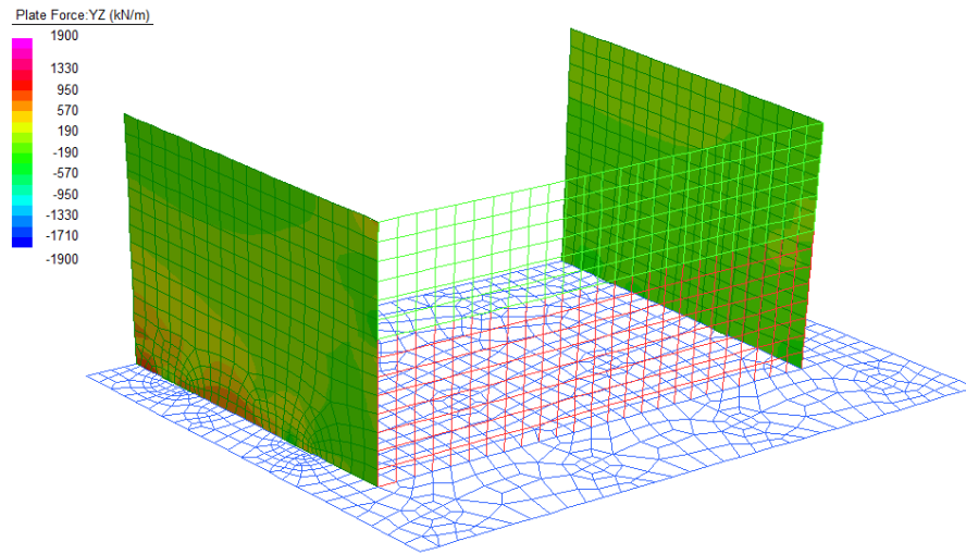
Figura 23: Sollecitazioni Taglianti V_{yz} - Involuppo SLU/SLV
