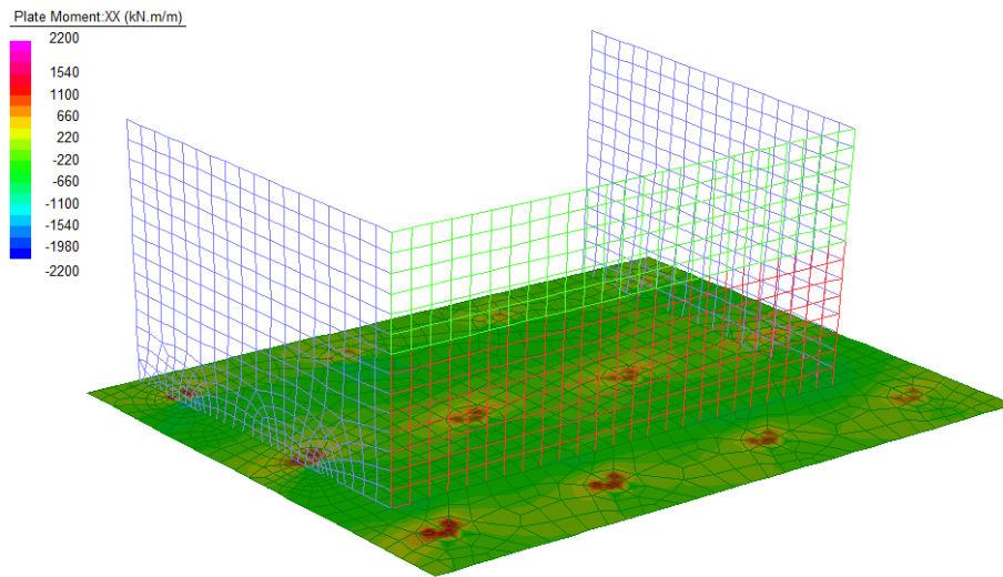
Figura 37: Momento Flettente longitudinale - Involuppo SLE
