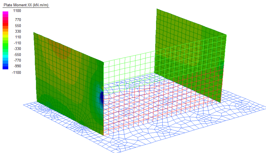
Figura 25: Momento Flettente orizzontale - Inviluppo SLE
