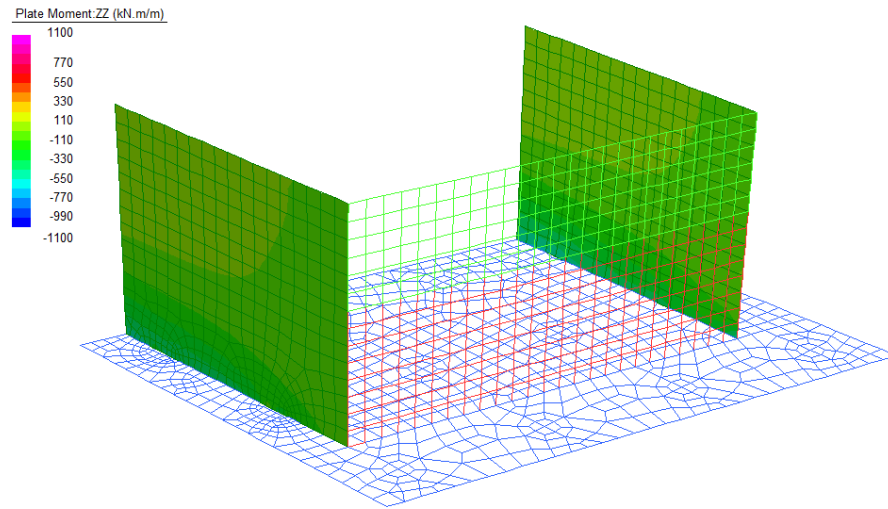
Figura 21: Momento Flettente verticale - Involuppo SLE
