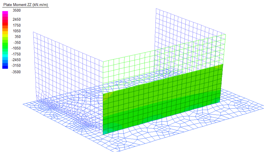
Figura 15: Momento Flettente verticale - Inviluppo SLE
