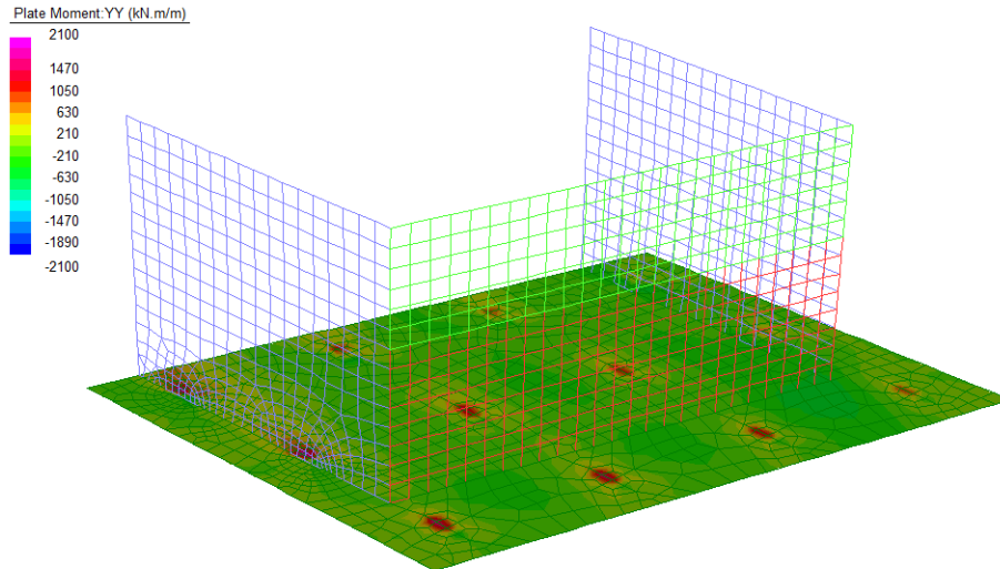
Figura 33: Momento Flettente trasversale - Inviluppo SLE
