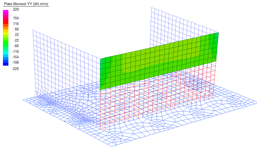
Figura 31: Momento Flettente orizzontale - Inviluppo SLE
