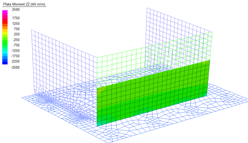
Figura 15: Momento Flettente verticale - Inviluppo SLE
